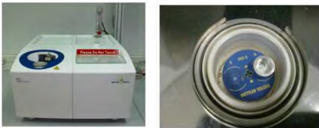
Figura 1. DSC - calorimetro differenziale a scansione e particolare del fornello contenente la zona per il campione ed il riferimento (crogiolo tappato vuoto)
