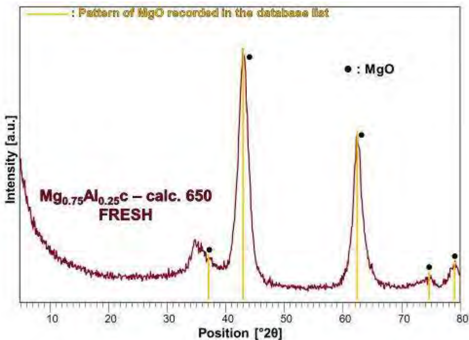
Figura 1. Diffattogramma del campione Mg_{0.75}Al_{0.25} calcinato a 650 °C per 12 ore
