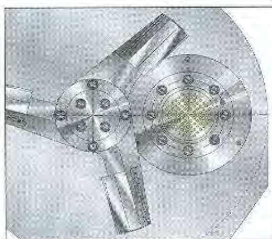
Figura 11. Particolare del taglio in testa: a sinistra si può vedere la lama a tre lobi che girando taglia ciò che esce dalla trafila direttamente a misura
