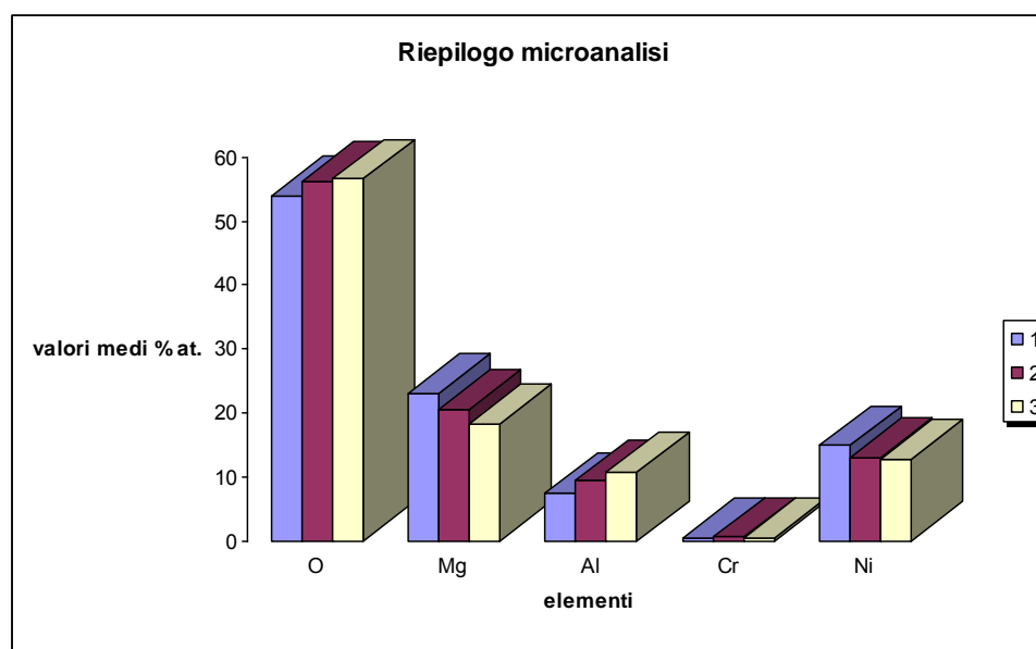
Figura 12. Riepilogo andamento valori medi delle percentuali atomiche elementi individuati nei tre catalizzatori
