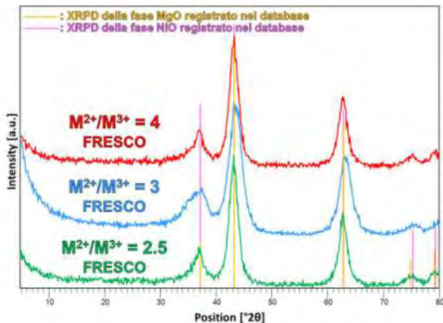
Figura 2. Spettri XRD dei campioni a diverso rapporto M^{2+}/M^{3+} , dopo calcinazione a 650\text{ }^\circ\text{C}
