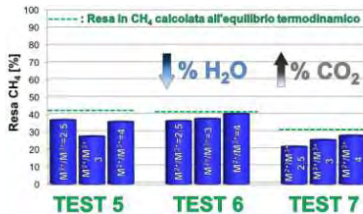
Figura 7. Resa in metano ottenuta con i campioni a diverso rapporto M^{2+}/M^{3+} nelle prove di metanazione (TEST 5, 6, 7) e confronto con i valori calcolati all'equilibrio termodinamico
