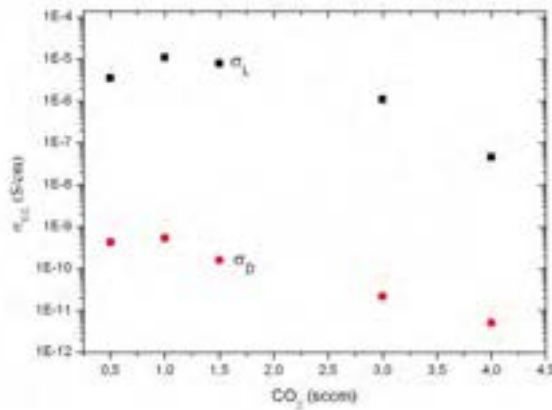
Figura 8: Effetto del flusso di CO_2 sulla conducibilità elettrica dark e light (serie ad H_2=120 sccm e P=6 W).
