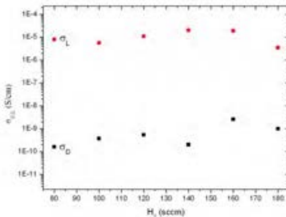
Figura 9: Effetto del flusso di H_2 sulla conducibilità elettrica dark e light (serie a CO_2=1 sccm e P=6 W).
