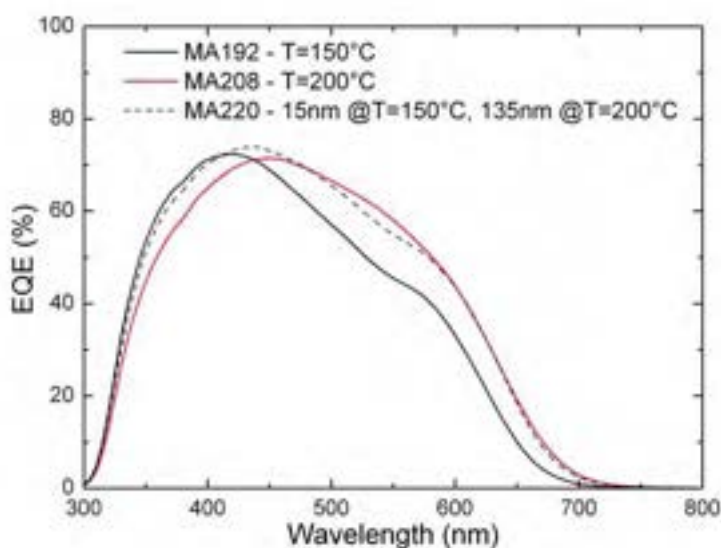
Figura 15 – Confronto tra le EQE misurate sulle celle il cui strato intrinseco in a-SiO x :H è cresciuto a temperatura diversa.
