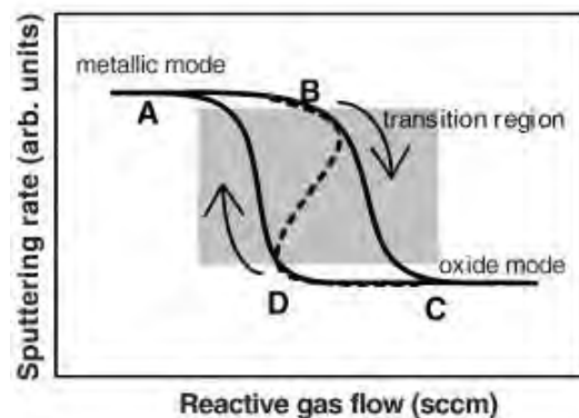
Figura 5. Curva d'isteresi tipica dei processi di sputtering reattivo.
