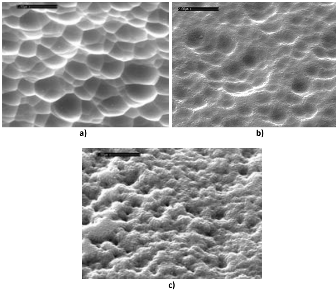
Figura 24. Immagini SEM della morfologia superficiale di: a) vetro testurizzato con processo AIT con trattamento basico in NaOH ed HF per 4 min, b) struttura GZO/vetro testurizzato con HF per 4 min, c) struttura GZO/vetro testurizzato con HF-HNO 3 per 150 sec.
