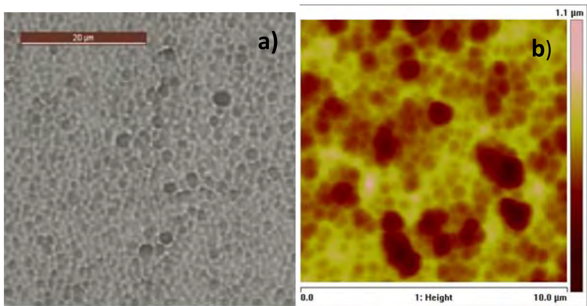
Figura 9. (a) Immagine al microscopio ottico; (b) immagine AFM che mostrano l'uniformità di testurizzazione su diverse scale di ingrandimento di vetri rugosi ottenuti da AlN (graded).
