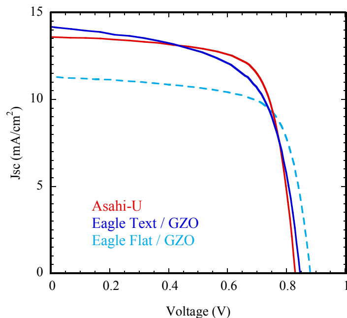
Figura 36 – Curve I-V misurate in condizioni di illuminazione AM1.5G su celle di silicio amorfo realizzate su substrato con elettrodo frontale di GZO su vetro flat e su vetro testurizzato con metodo AIT. E' riportato il confronto con substrato commerciale di Asahi-U.
