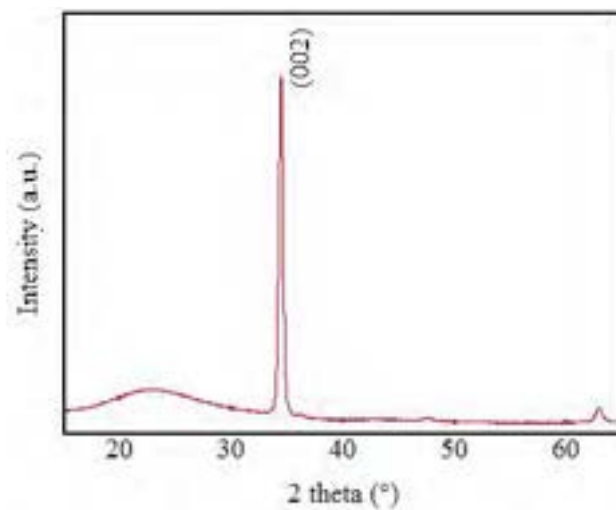
Figura 25. Spettro XRD di un film di GZO depositato su vetro testurizzato.
