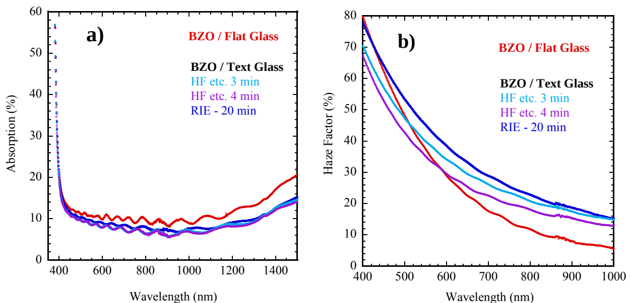
Figura 32. Andamento a) dell'assorbanza e b) del fattore di Haze di film di BZO depositati su vetro flat e su vetro rugoso.
