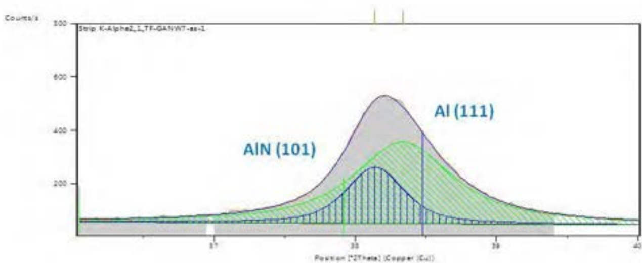
Figura 7. Deconvoluzione del picco a 2\theta=38.2^\circ relativo allo spettro di Fig.6 dell'AlN as deposited.
