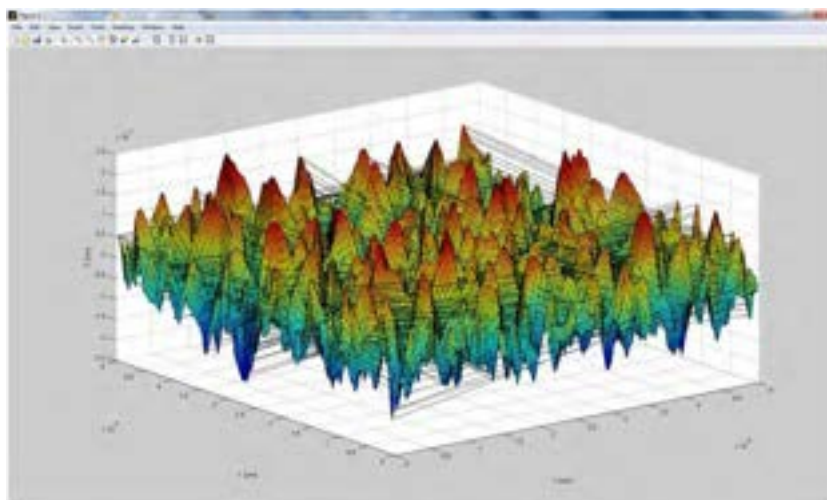
Figura 16. Immagine AFM rielaborata in MATLAB (scala dell'asse delle z dilatata).
