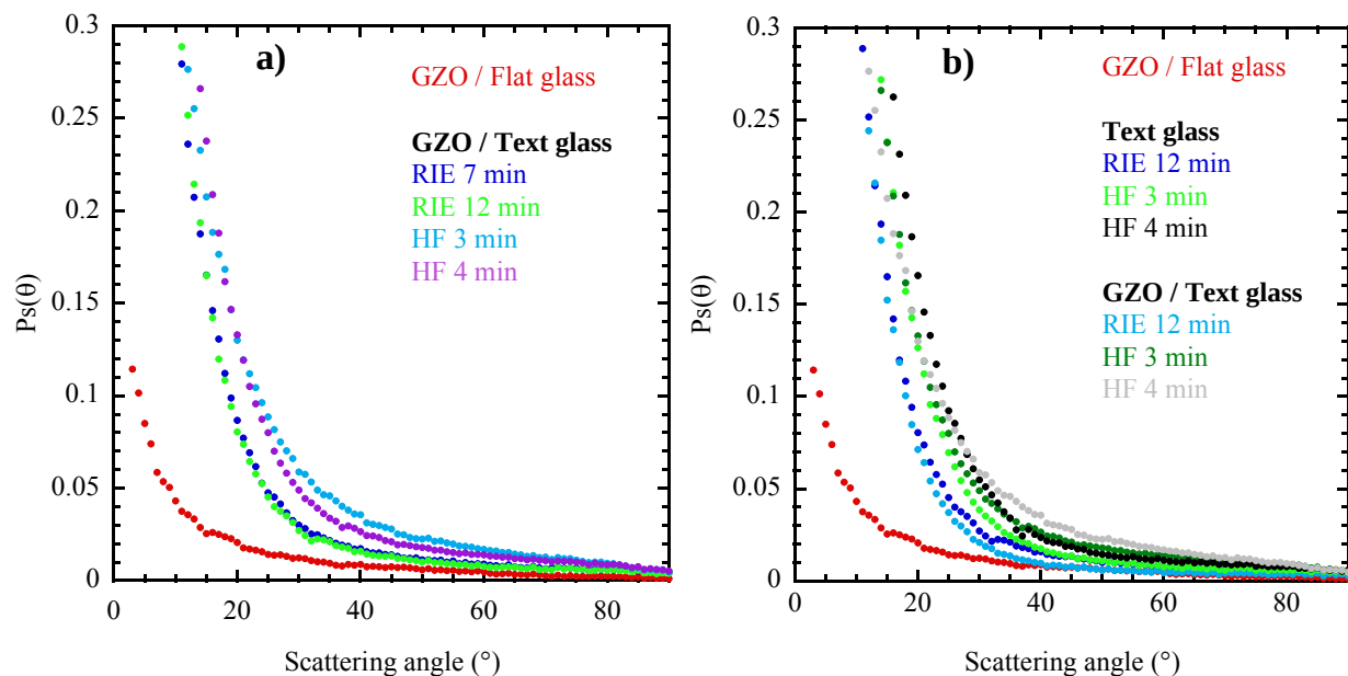
Figura 30. Curve di scattering al variare dell'angolo (ARS) di film di GZO depositati su vetro flat e su vetro rugoso.
