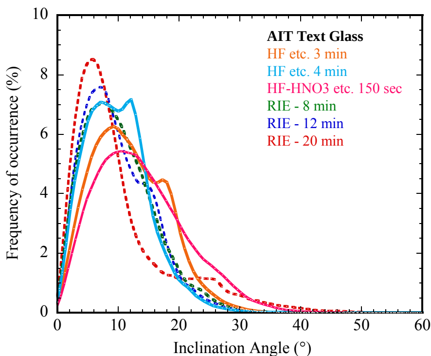
Figura 22. Istogramma della distribuzione degli angoli derivato dalle immagini AFM di vetri testurizzati con tecnica AIT con differenti trattamenti post-annealing.
