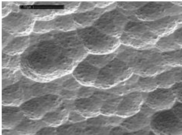
Figura 12. Particolari della morfologia superficiale di un substrato attaccato con RIE per 12 min.
