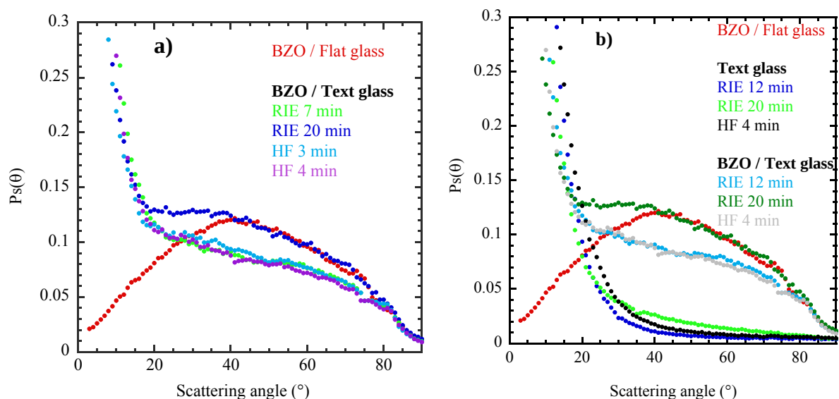
Figura 33. Potenza di scattering derivata dalla intensità trasmessa misurata con tecnica ARS in funzione dell'angolo di scattering per film di a) BZO depositati su vetro flat e su vetro rugoso e b) confronto con misure ARS del vetro testurizzato..
