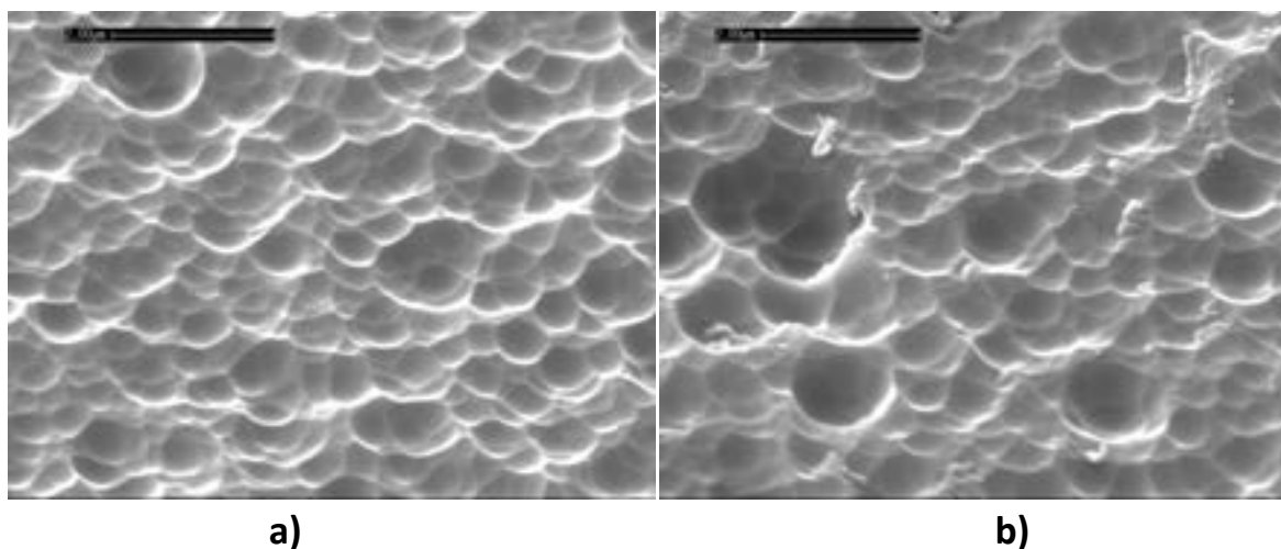
Figura 8. Immagini SEM della morfologia superficiale di vetri trattati con tecnica AIT utilizzando un film di AlN: a) 7 sccm di N 2 , b) graded.
