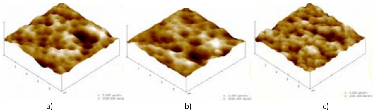
Figura 27. Immagini AFM di GZO/vetro testurizzato con differente durata di attacco chimico post-annealing: a) 3 min in HF, b) 4 min in HF e c) 150 sec in HF-HNO 3 .
