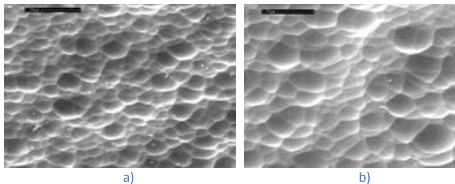
Figura 11. Immagini SEM della morfologia di vetri testurizzati. Effetto della durata dell'etching in HF: a) 3 min e b) 4 min.
