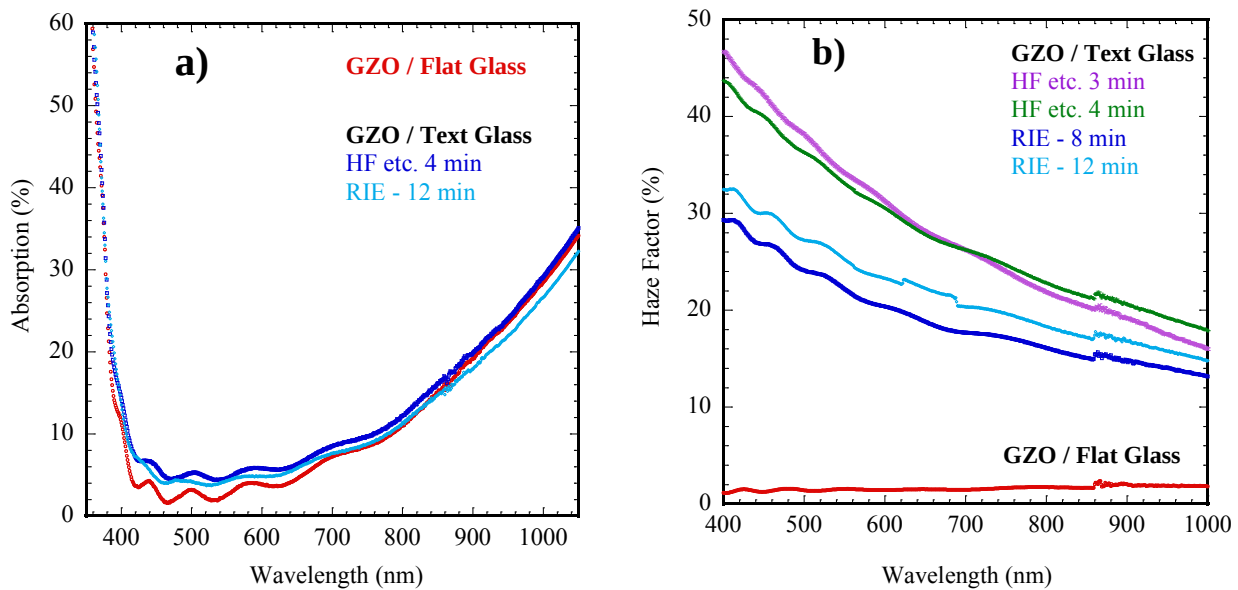
Figura 29. Andamento a) dell'assorbanza e b) del fattore di Haze di film di GZO depositati su vetro flat e su vetro rugoso con differenti condizioni di etching.
