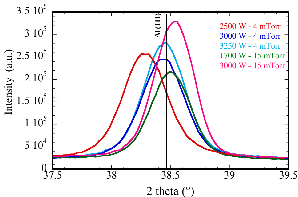
Figura 3. Spettri di diffrazione a raggi-x di film di Al depositati a differenti condizioni di potenza e pressione di processo.
