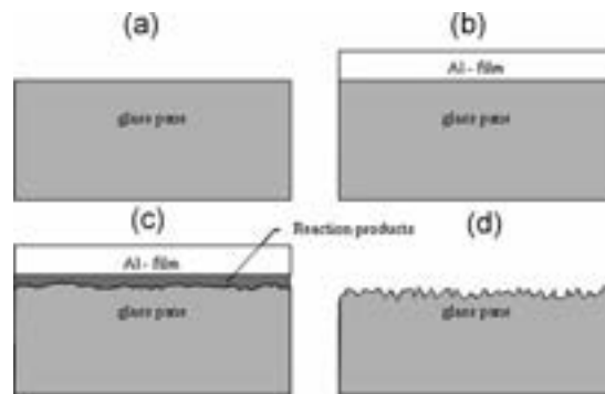
Figura 1. Sequenza del processo della tecnologia AIT.
