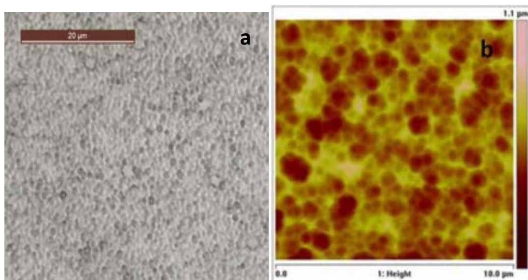
Figura 10. Immagini della morfologia superficiale a) ottica, b) AFM che mostrano l'uniformità di testurizzazione su diverse scale di ingrandimento di vetri rugosi ottenuti da AlN (7sccm).
