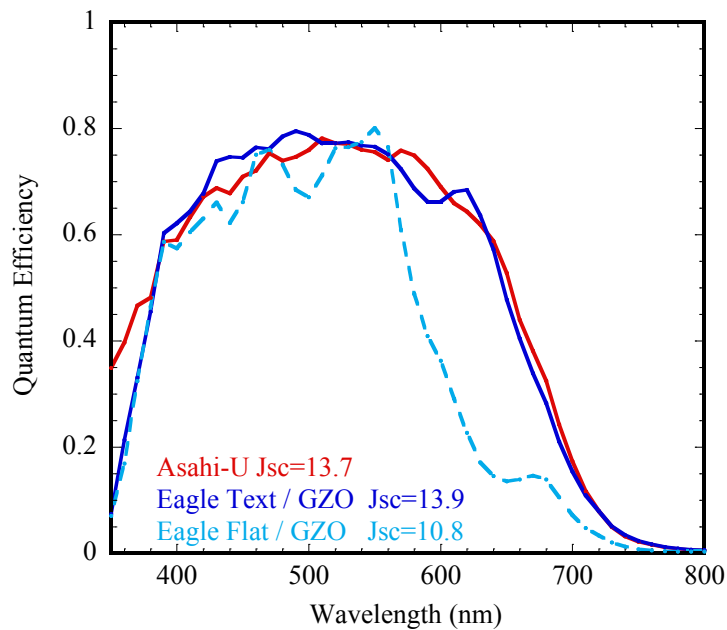
Figura 35. Confronto tra le curve di risposta spettrale misurate su celle di silicio amorfo realizzate su substrato con elettrodo frontale di GZO su vetro flat e su vetro testurizzato con metodo AIT. E' riportato il confronto con substrato commerciale di Asahi-U.
