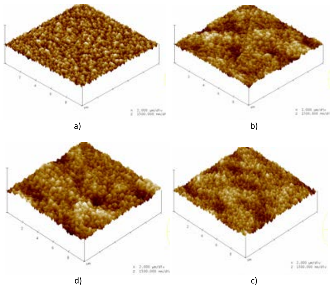
Figura 31. Immagini AFM della morfologia superficiale di un film di ZnO:B depositato per MOCVD su: a) vetro flat, b), c), d) vetro rugoso prodotto con tecnica AIT ed etching in HF per 3 min, 4 min e RIE 20 min rispettivamente.
