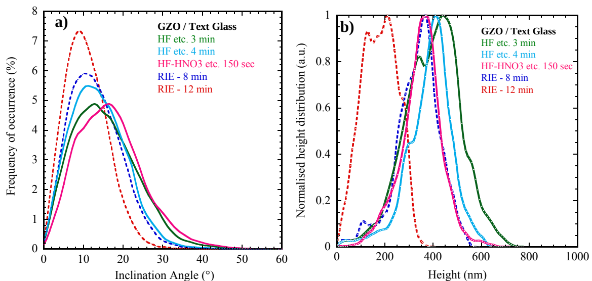
Figura 28. a) Istogramma della distribuzione degli angoli. b) distribuzione delle altezze derivate dalle immagini AFM di GZO/vetri testurizzati con tecnica AIT sottoposti a differenti trattamenti post-annealing.
