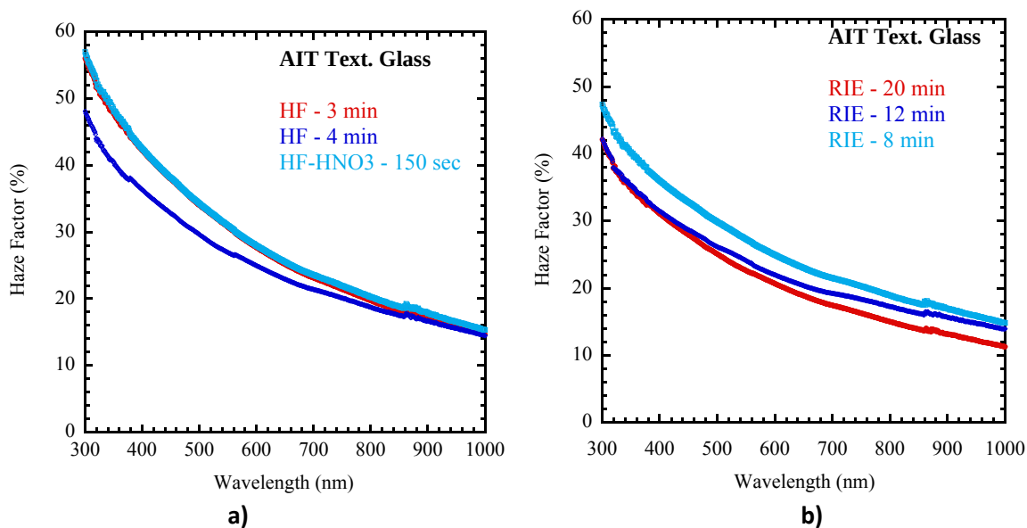
Figura 13. Andamento dell'Haze factor di superfici di vetro ottenute da: a) etching chimico e b) trattamento RIE dopo etching chimico.
