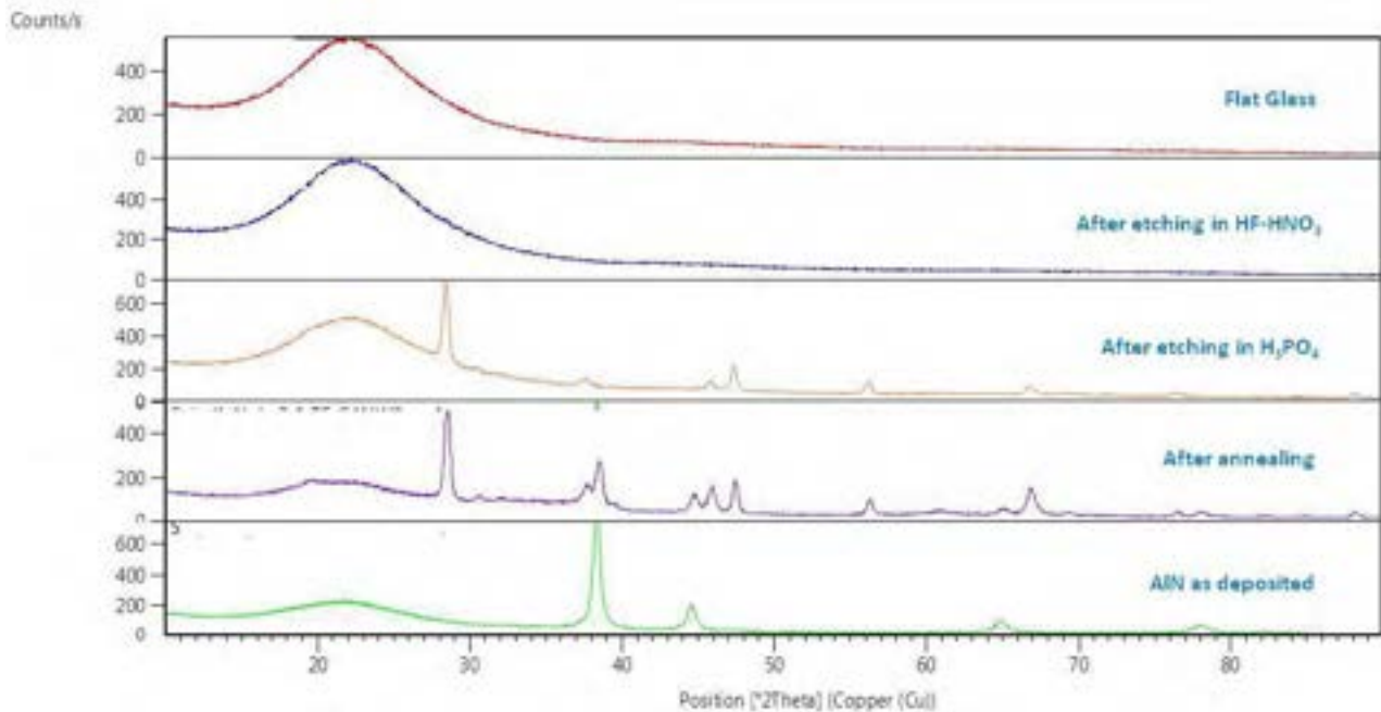
Figura 6. Spettri di diffrazione a raggi-x di un substrato di vetro Corning con film di AlN, prima e dopo annealing in forno e dopo attacco chimico.
