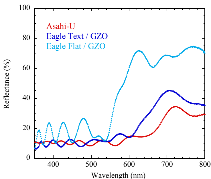
Figura 34. Confronto della riflettenza misurata su celle di silicio amorfo realizzate su substrato con elettrodo frontale di GZO su vetro flat e su vetro testurizzato con metodo AIT. E' riportato il confronto con substrato commerciale di Asahi-U.
