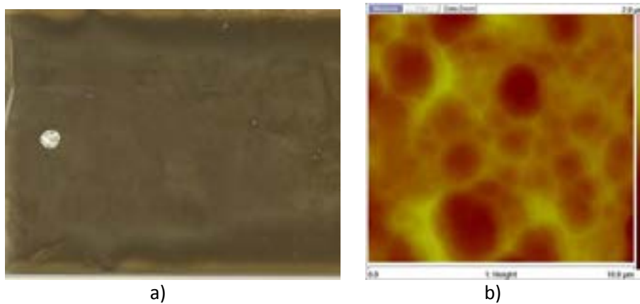
Figura 14. Substrato di vetro Boroflat: a) aspetto della superficie dopo annealing, b) immagine AFM della superficie dopo wet-etching.
