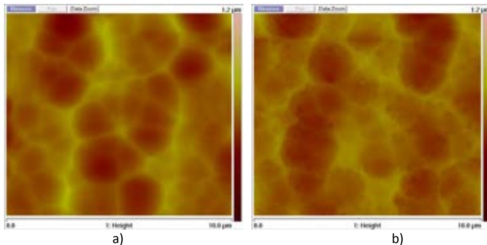
Figura 21. Immagini AFM di vetri sottoposti ad attacco mediante RIE con CF 4 per tempi differenti: a) 8 min e b) 20 min.
