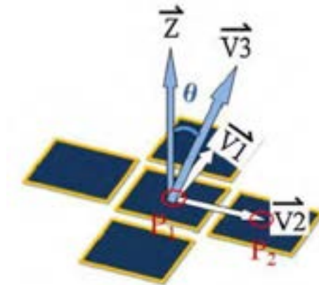
Figura 17. Schema di principio per la misura dell'angolo di inclinazione dei pixel costituenti le immagini AFM.
