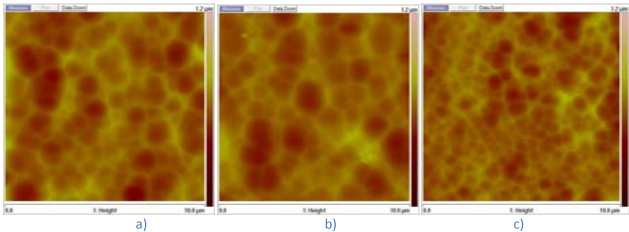
Figura 20. Immagini AFM. Confronto tra etching in HF di differente durata(a e b) e tra etching in HF e miscela HF-HNO 3 (c)
