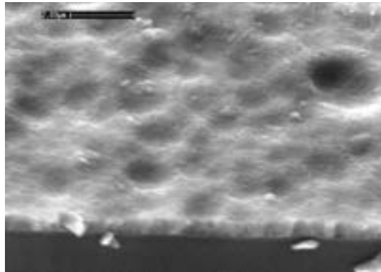
Figura 26. Immagini SEM della vista in sezione di un film di GZO/vetro testurizzato mostrando uniformità di spessore del deposito.
