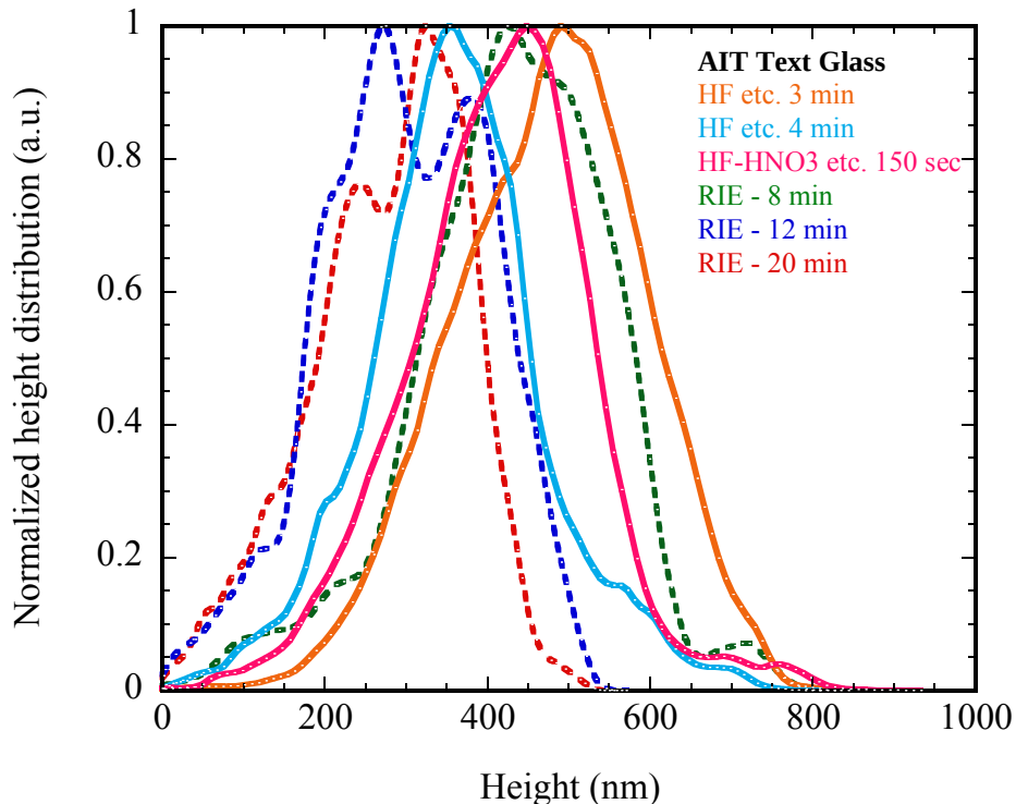
Figura 23. Istogramma della distribuzione delle altezze derivato dalle immagini AFM di vetri testurizzati con tecnica AIT con differenti trattamenti post-annealing.
