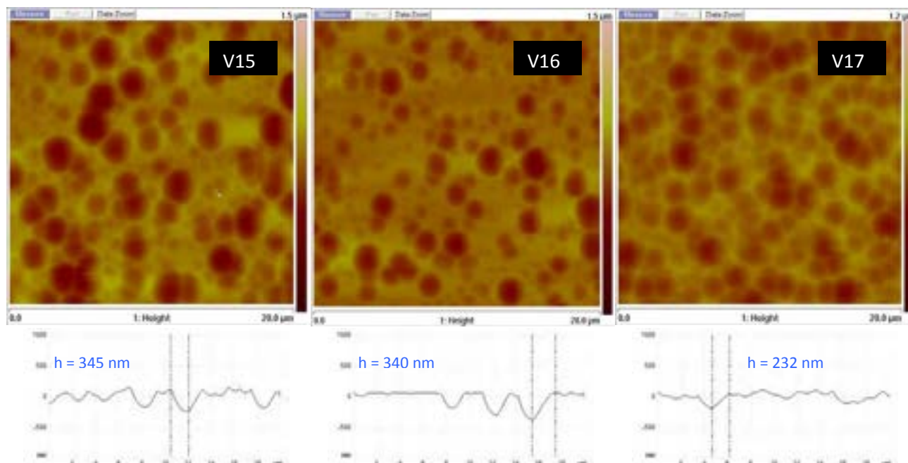
Figura 23. Immagini AFM della superficie testurizzata dei vetri di tipo V15, V16 e V17 con i relativi profili di scansione della profondità di scavo.
