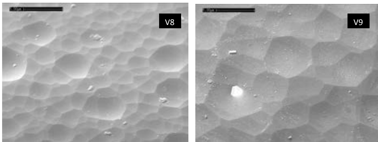
Figura 16. Immagini SEM della superficie testurizzata dei vetri di tipo V8 e V9.
