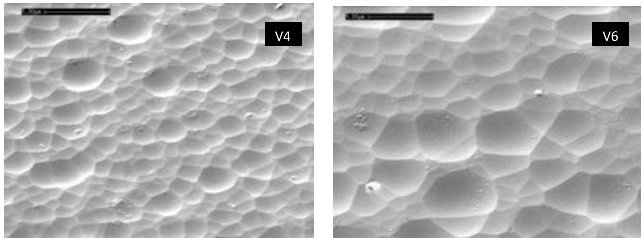
Figura 15. Immagini SEM della superficie testurizzata dei vetri di tipo V4 e V6.
