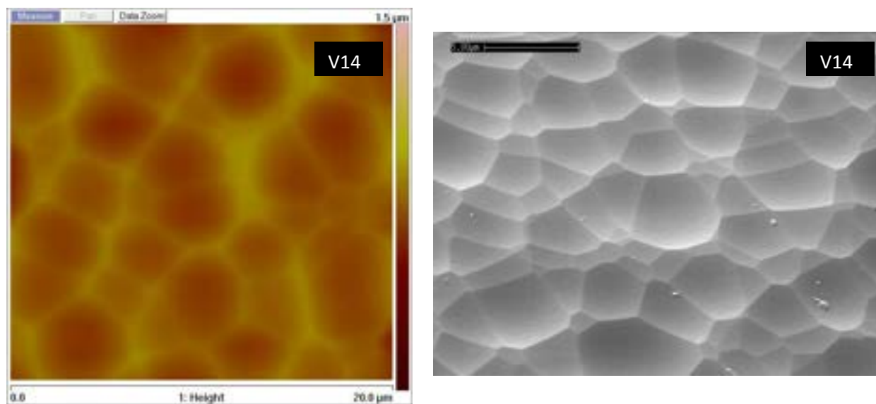
Figura 22. Immagini AFM (a sinistra) e SEM (a destra) della superficie testurizzata del vetro di tipo V14.
