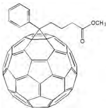
Figura 2. Struttura dell'estere metilico del [6,6]-fenil-C61-acido butirrico (PCBM).
