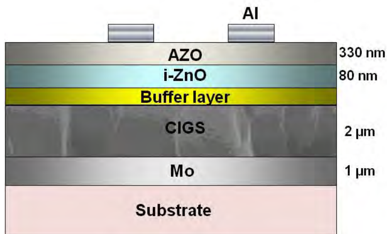
Figura 2. Schema delle celle in CIGS realizzate con i buffer layer alternativi.
