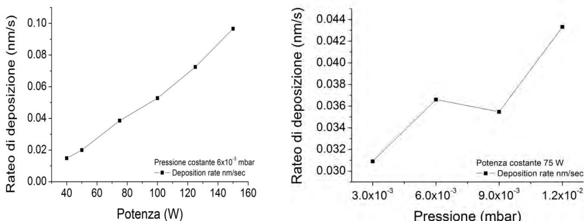
Figura 5: Dipendenza della velocità di deposizione per film di ZnS dalla potenza di deposizione (sinistra) e dalla pressione (destra).
