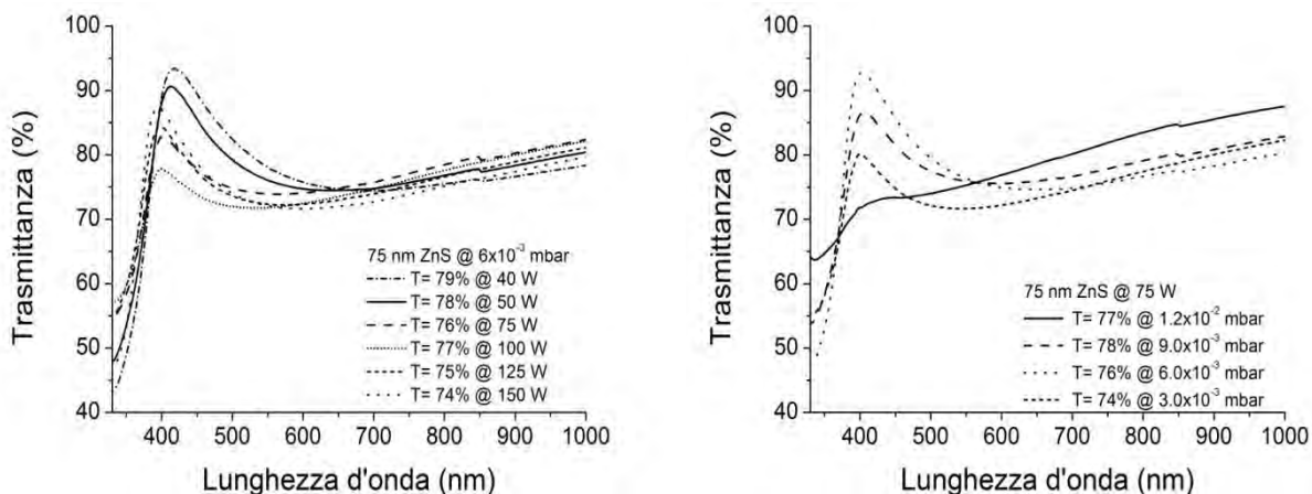
Figura 6. Spettri di trasmittanza di film di ZnS di spessore 75 nm in funzione della potenza di sputtering (sinistra) e della pressione (destra).
