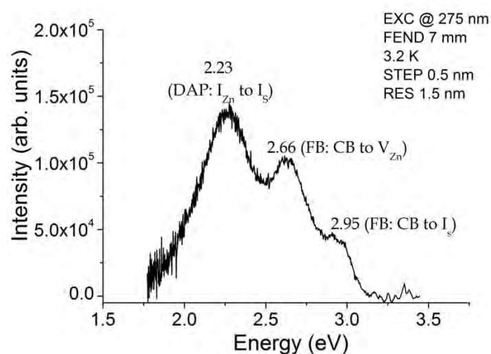
Figura 8. Esempio di spettro di fotoluminescenza a 3.2 K con \lambda di eccitazione a 275 nm di un film di ZnS. Le attribuzioni dei vari picchi a transizioni tra banda di conduzione (CB) e livelli energetici associati a difetti di punto sono indicati in [9]
