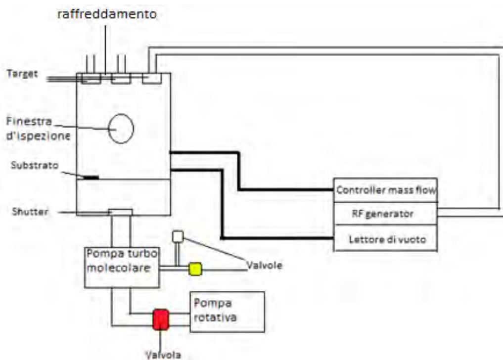
Figura 1 Schema dell'attrezzatura utilizzata per il processo di sputtering
