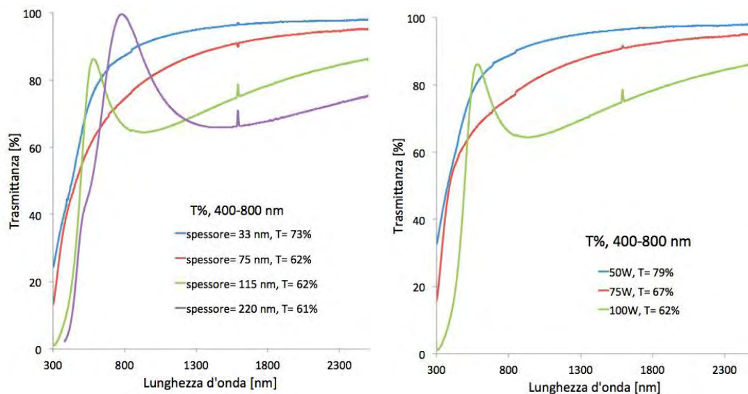
Figura 4. Trasmittanze di film di \text{In}_2\text{S}_3 per diversi valori di spessore (a) e di potenza (b)
