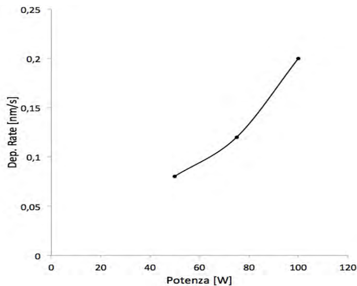
Figura 3. Dipendenza della velocità di deposizione di film di \text{In}_2\text{S}_3 in funzione della potenza di deposizione
