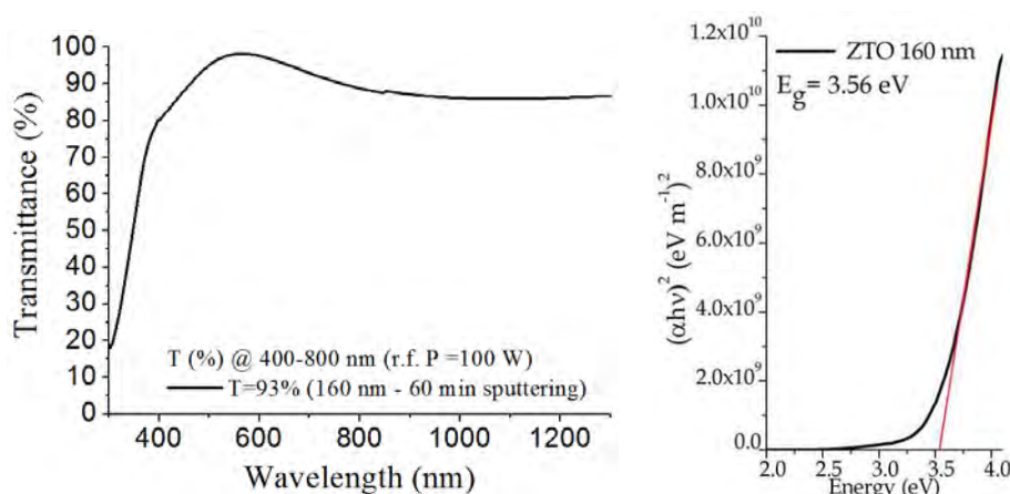
Figura 10: (a) Tipico spettro di trasmissione nel range spettrale 300-1300 nm (b) calcolo di energy gap di un campione di Zn_2SnO_4 di spessore 160 nm
