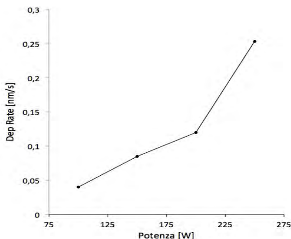
Figura 9: Dipendenza della velocità di deposizione per film di Zn_2SnO_4 dalla potenza di deposizione
