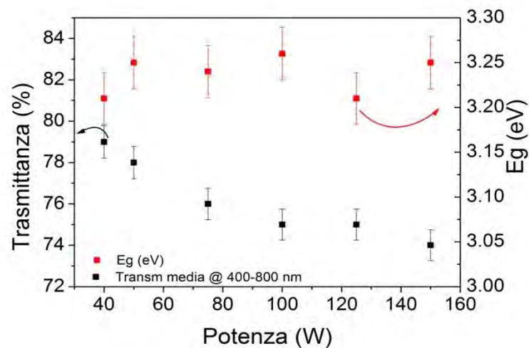
Figura 7. Trasmittanza media e optical Energy gap in funzione della potenza di sputtering.
