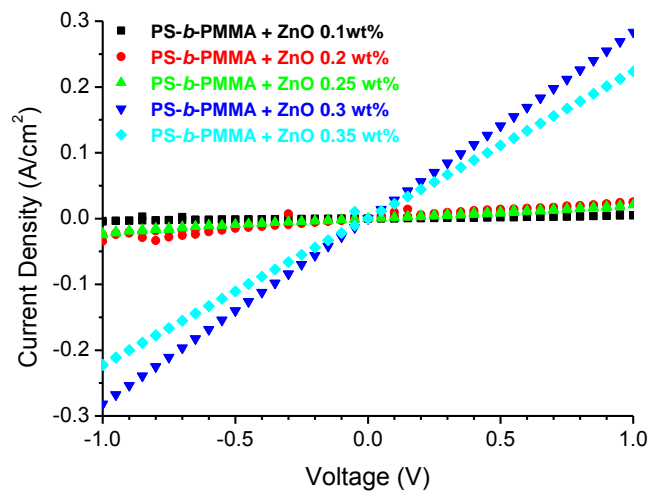
Figura 6. Caratteristiche I-V del dispositivo ITO/PS -PMMA:ZnO/Al. I films sono stati sottoposti a trattamento termico sotto vuoto per 6h a 150 h.
