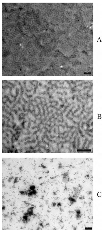
Figura 5. Microfotografie TEM di film sottili ottenuti da soluzione di toluene a concentrazione 1 wt% di BCP e 0.1 wt% di ZnO NPs (A, B) e da una soluzione di toluene a concentrazione 1% di PS omopolimero e 0.6 wt% di ZnO NPs. In A il contrasto è determinato dall'inclusione selettiva delle nanoparticelle di ZnO in specifici domini, in B il contrasto è potenziato dello staining con RuO 4 . Dal momento che RuO 4 marca in maniera selettiva i domini di PS, dal confronto tra le immagini A e B si deduce che ZnO è incluso in maniera selettiva nei domini di PS.
