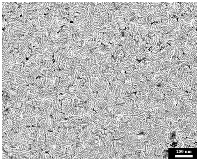
Figura 2. Microfotografia ottenuta attraverso microscopia elettronica in trasmissione (TEM) di un film sottile PS-PMMA (spessore \approx 70 nm), ottenuto per spin coating da una soluzione di toluene al 2wt% in BCP; dopo trattamento termico sotto vuoto per 6h, a 150 °C.
