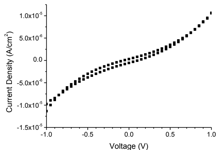
Figura 7. Caratteristiche I-V del dispositivo ITO/PS:ZnO/Al. La concentrazione di ZnO nella soluzione iniziale di toluene è 0.6 wt%.
