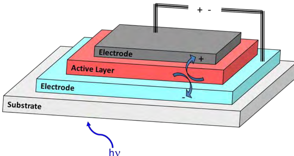
Figura 1. Schema di strato attivo in celle solari.
