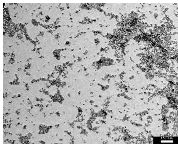
Figura 4. Microfotografia TEM delle nanoparticelle ZnO.
