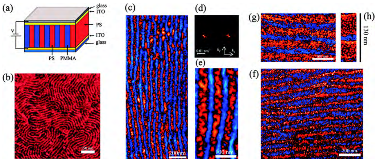
Figura 3. (a) Schema del capacitore verticale utilizzato per l'allineamento dei domini lamellari del BCP. (b) Immagine TEM bright-field (scala in false color) del film di PS-PMMA depositato su substrato di ITO prima dell'applicazione del campo elettrico (il campione è lo stesso di Figura 2 ma in una differente zona). (c) Microfotografia TEM di una zona del film sottile di PS-PMMA dopo allineamento in campo elettrico di 0.32 \text{ V } \mu\text{m}^{-1} (i domini lamellari di PS sono in rosso, quelli di PMMA in blu) e corrispondente (d) trasformata di Fourier. (e-h) Immagini TEM di altre regioni del film sottile a differenti ingrandimenti. I domini di PS sono marcati con \text{RuO}_4 per aumentare il contrasto. Nelle immagini f-h, nanoparticelle di Au sono state depositate selettivamente sul blocco di PS attraverso un processo di evaporazione/condensazione sotto vuoto spinto.
