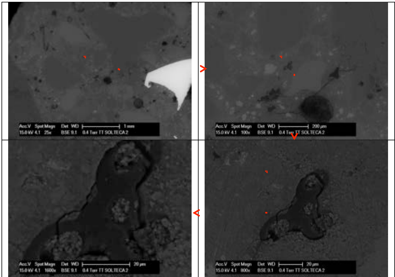
Figura 16 – Micrografie a ingrandimenti crescenti del calcestruzzo preparato con la miscela B dopo il trattamento is termico a 250°C per 4 ore. Zona contenente fibre di nylon.
