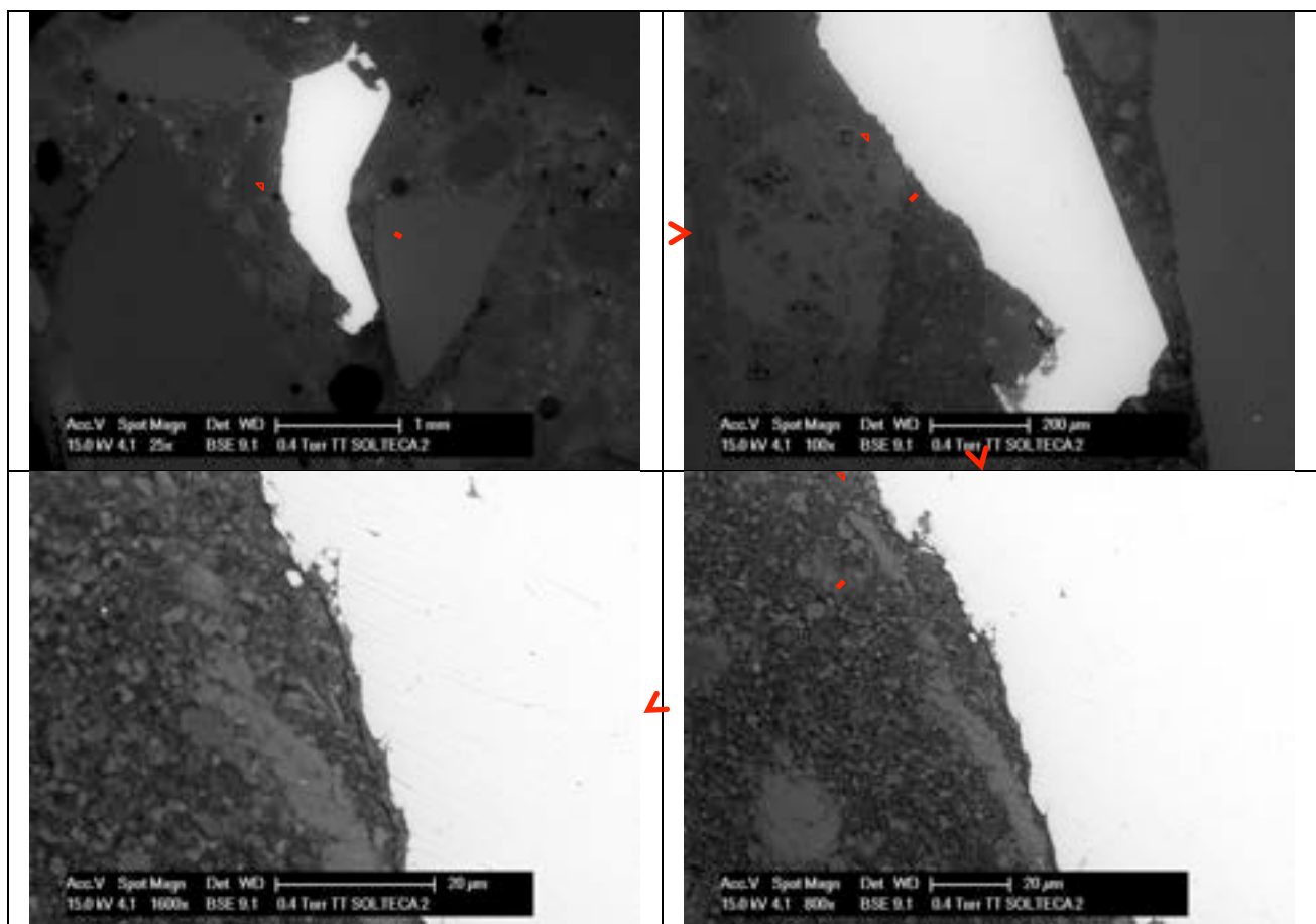
Figura 17 – Micrografie a ingrandimenti crescenti del calcestruzzo preparato con la miscela B dopo il trattamento isoteramico a 250°C per 4 ore. Zona contenente truciolo metallico
