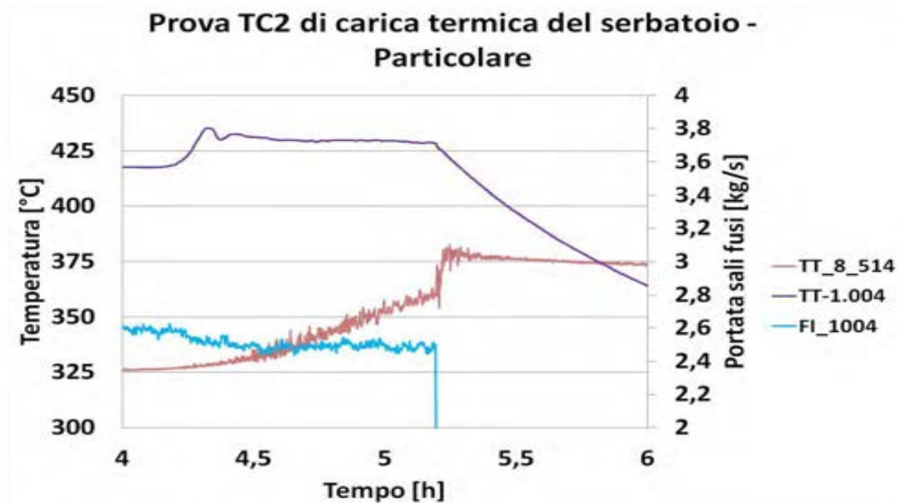
Figura 7 – Particolare della Prova TC2 con l'andamento oscillante della temperatura TT_8_514 dello strato più profondo
