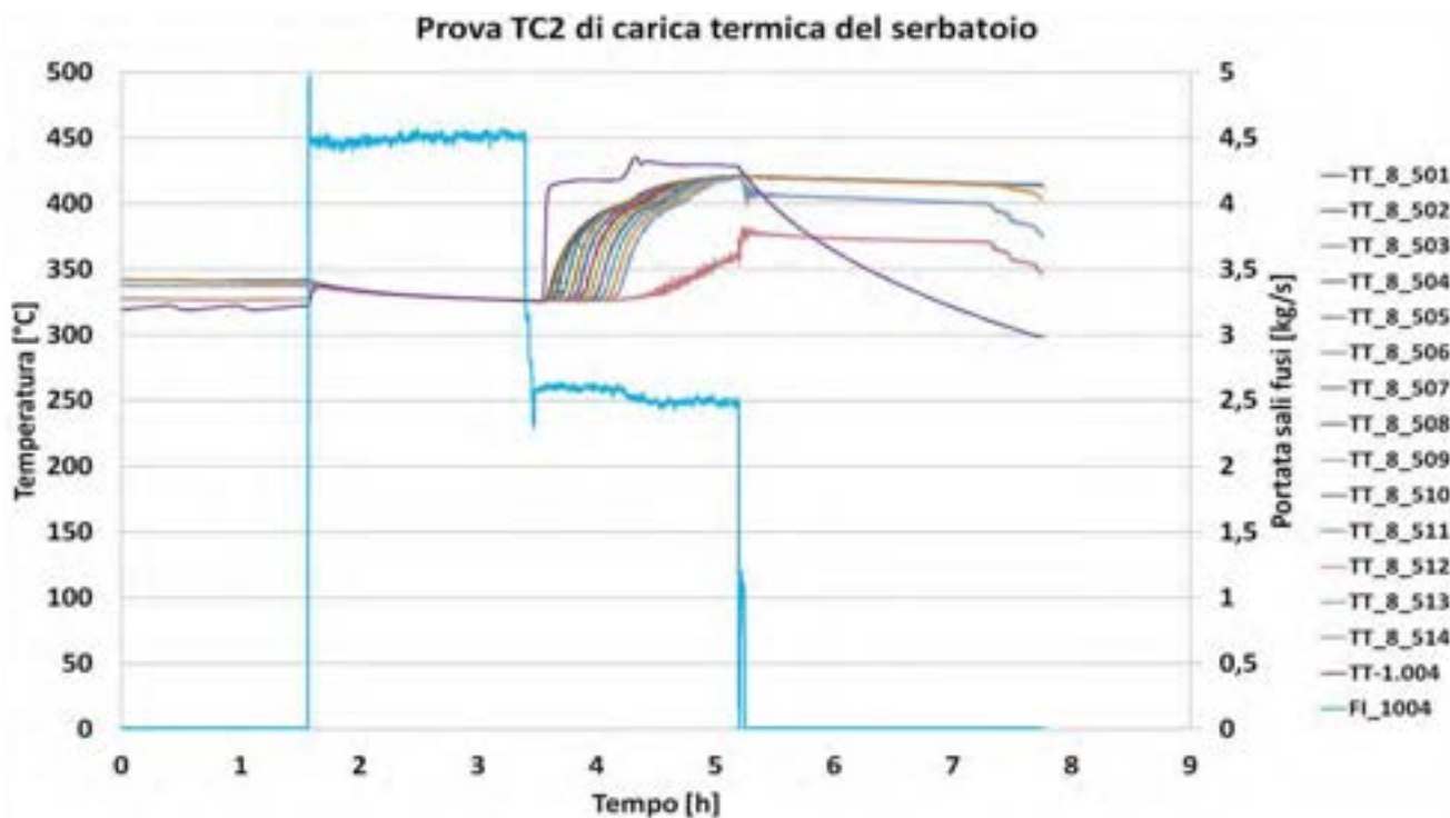
Figura 5 – Andamento delle temperature di stratificazione e della portata dei sali fusi nella Prova TC2
