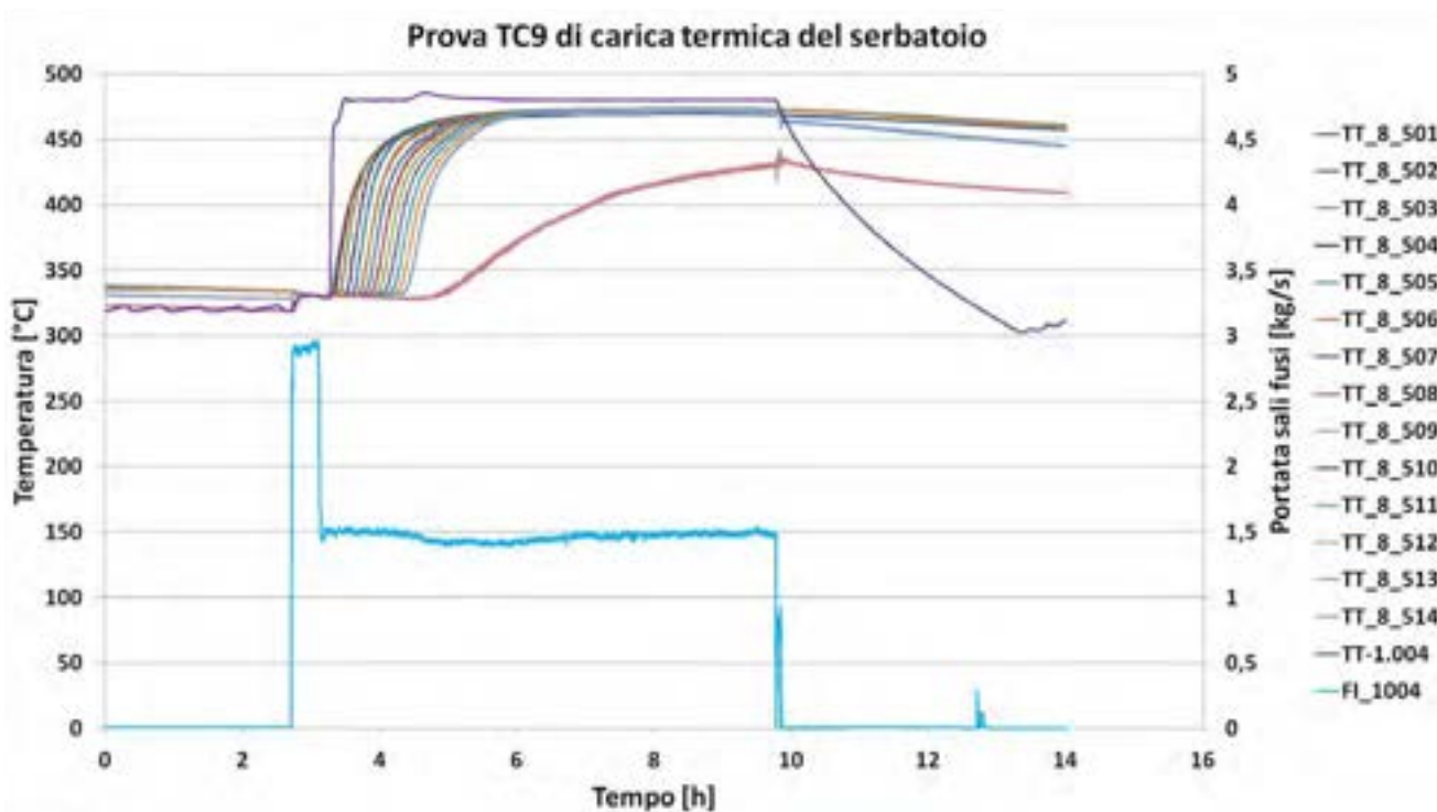
Figura 6 – Andamento delle temperature di stratificazione e della portata dei sali fusi nella Prova TC9
