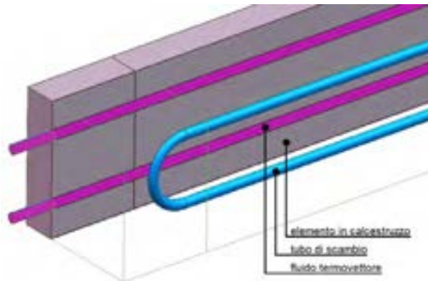
Fig. 17 Sezione modello 3D.
