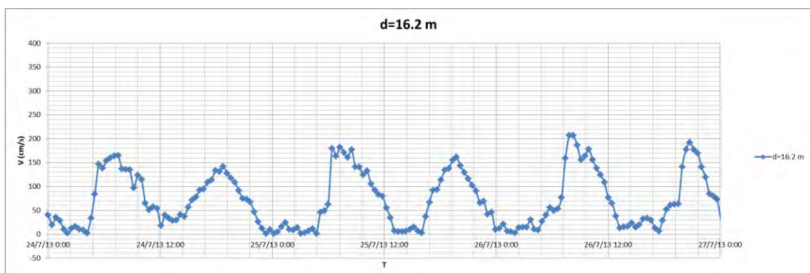
Figura 7. Modulo della velocità rilevata a 16.2 m di profondità.
