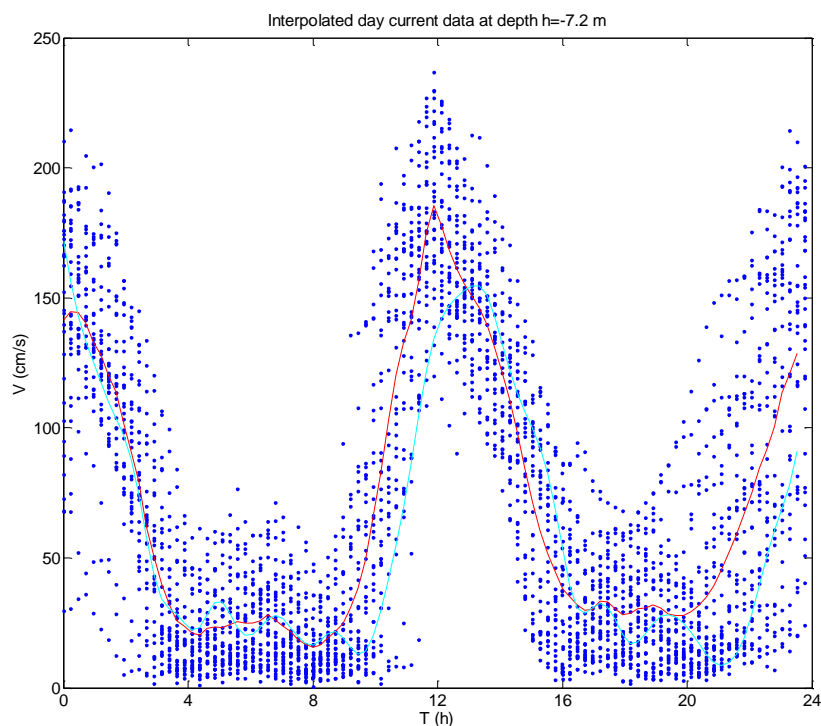
Figura 10. Sovrapposizione degli andamenti giornalieri medi, con l'individuazione di due picchi della velocità della corrente (profondità di 7.2 m).
