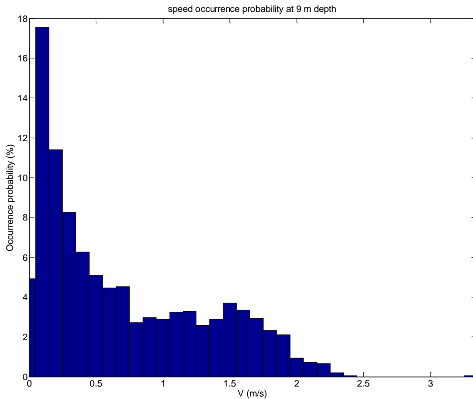
Figura 12. Istogramma della velocità nel sito di esempio, ad una profondità d 9 m.
