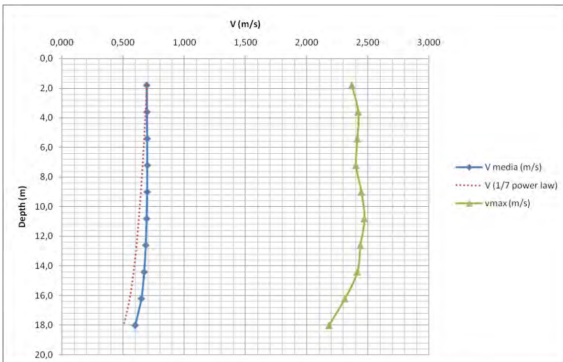
Figura 14. Velocità media al variare della profondità.
