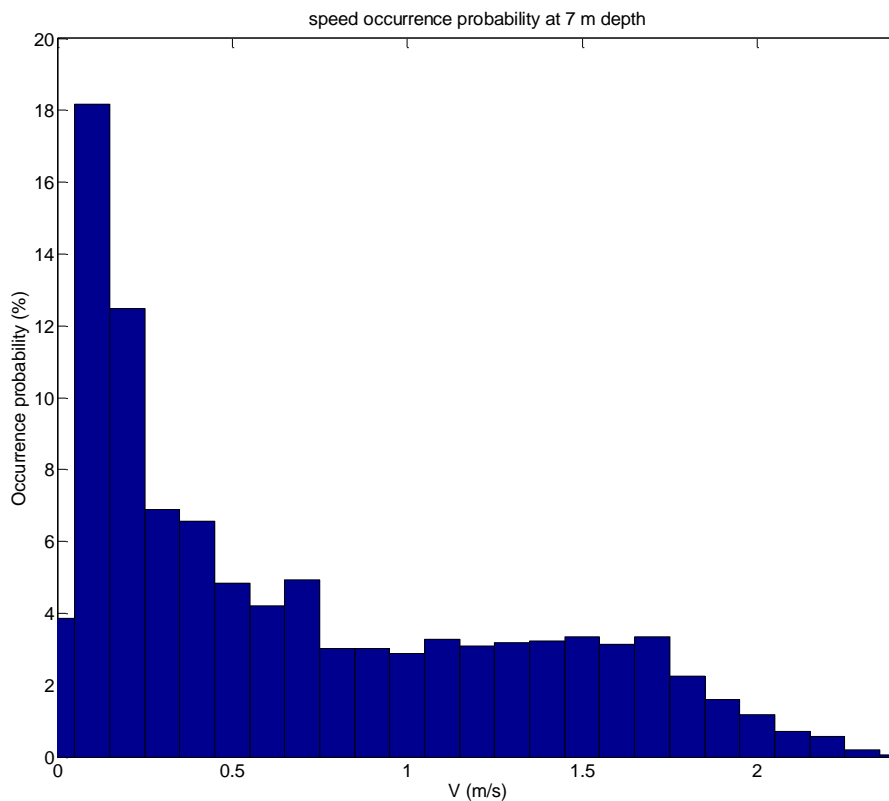
Figura 13. Istogramma della velocità nel sito di esempio, ad una profondità d 7 m.
