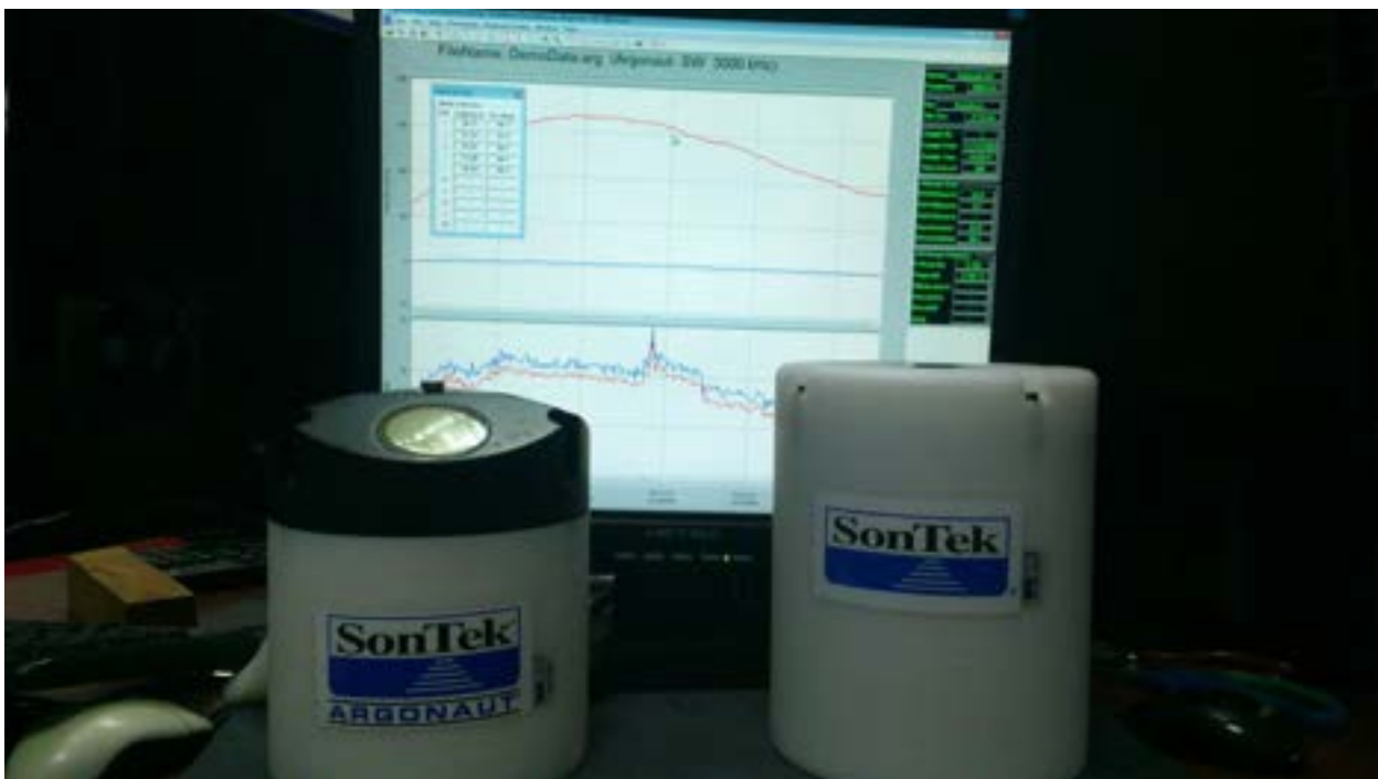
Figura 3. Sistema acquistato Argonaut-XR con batteria e software di gestione e controllo.
