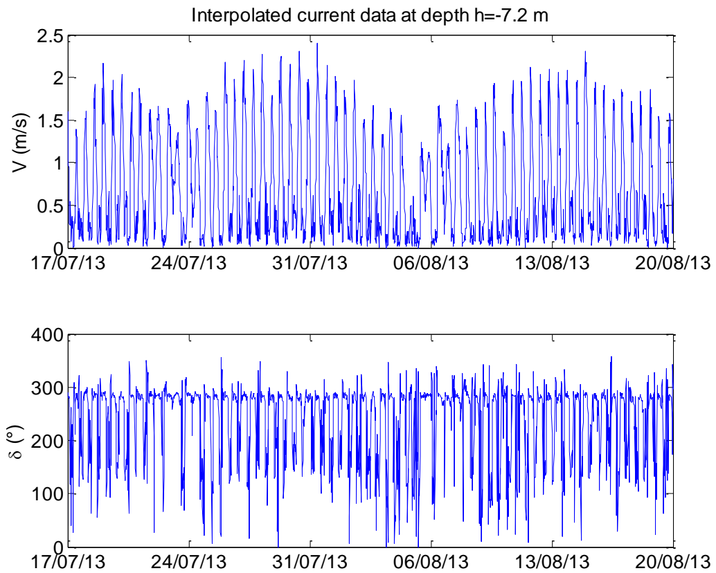
Figura 8. Velocità nel piano orizzontale e direzione della corrente nel sito di installazione a 7.2 m di profondità.
