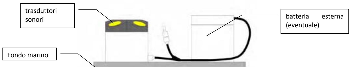
Figura 1. Schema di installazione dell'ADCP SonTekArgonaut XR (montaggio sul fondale, up-looking).
