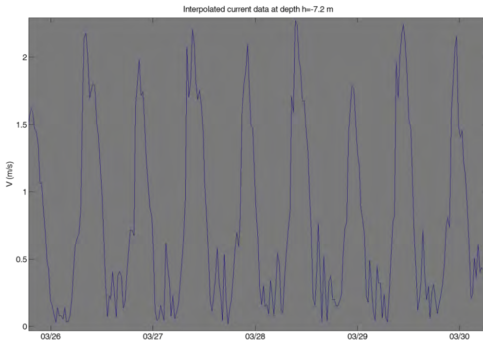
Figura 9. Velocità della corrente nel sito di esempio a 7.2 m di profondità (dettaglio temporale).
