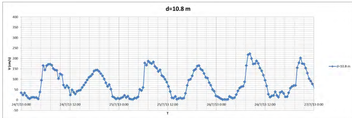
Figura 6. Modulo della velocità rilevata a 10.8 m di profondità.
