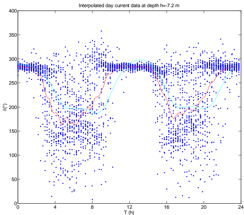
Figura 11. Variazioni giornaliere della direzione della corrente.
