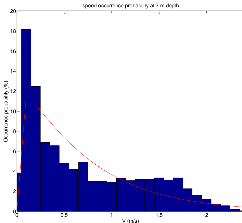
Figura 15. Distribuzione di Weibull (velocità alla profondità di 7 m).
