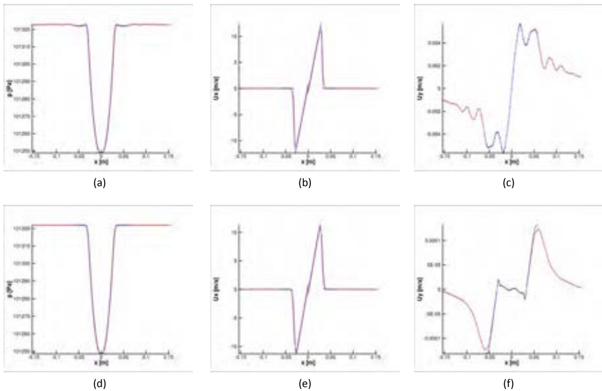
Figura 6.5: Campi Fluidodinamici di Pressione, Velocitá Tangenziale e Radiale
