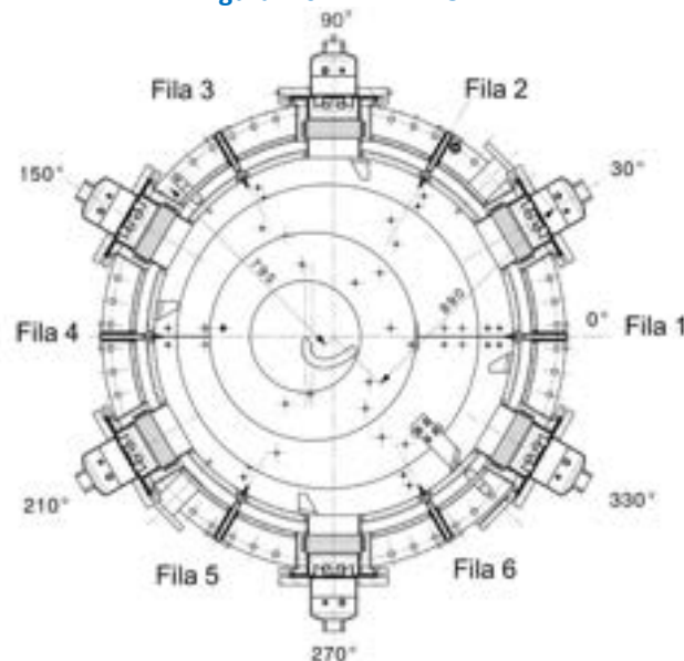
Figura 2.6 IRRADIATORE.
