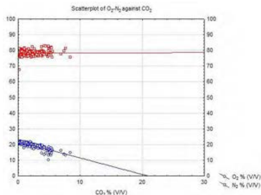
Figura 6 Scatterplot O2-N2 against CO2. Questo tipo di grafico dà indicazioni circa l'origine della CO2.
