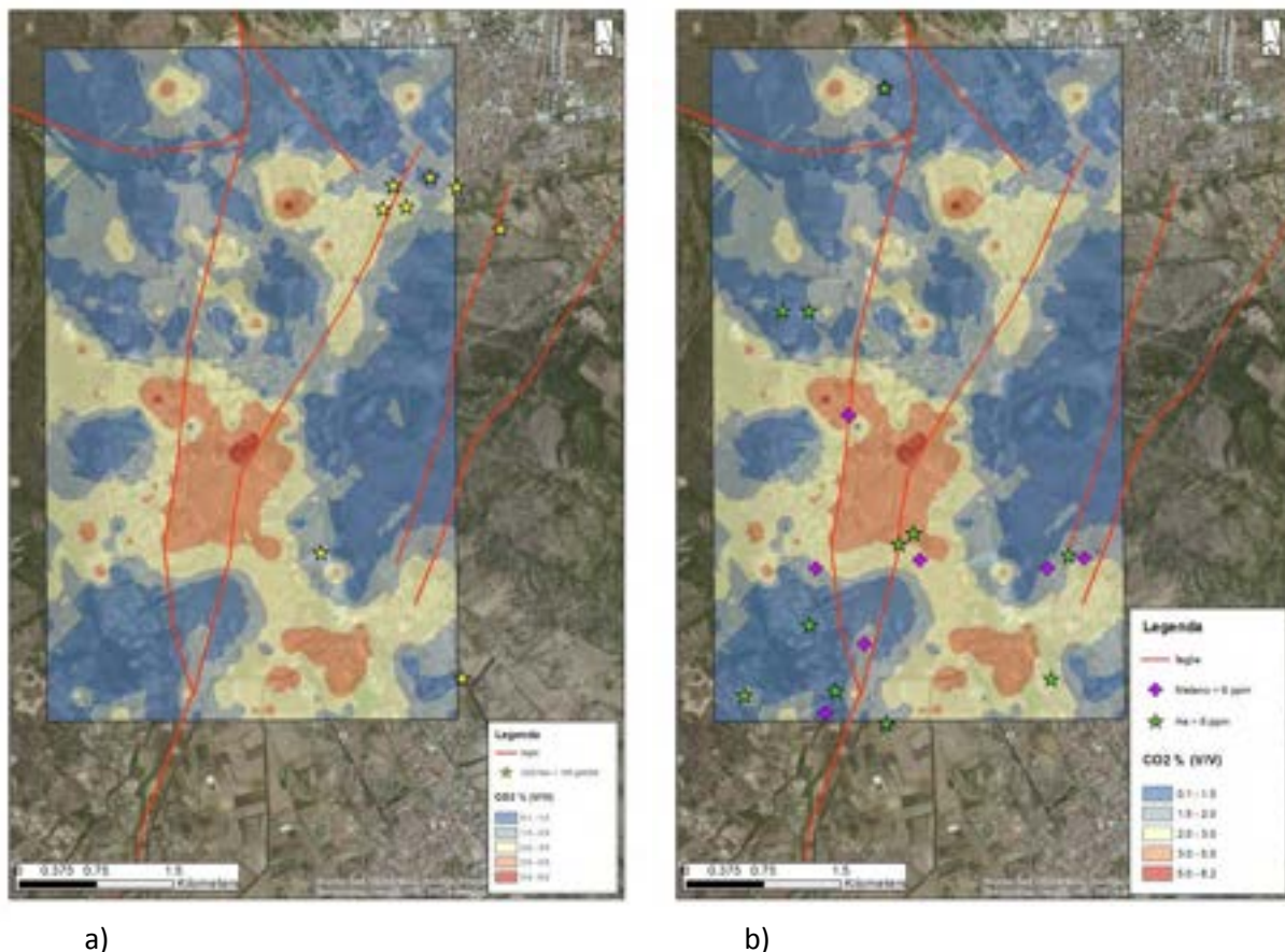
Figura 13 Contour map della CO 2 sovrapposta a classed post map di Flusso di CO 2 (13a) e He e CH 4 (13b)
