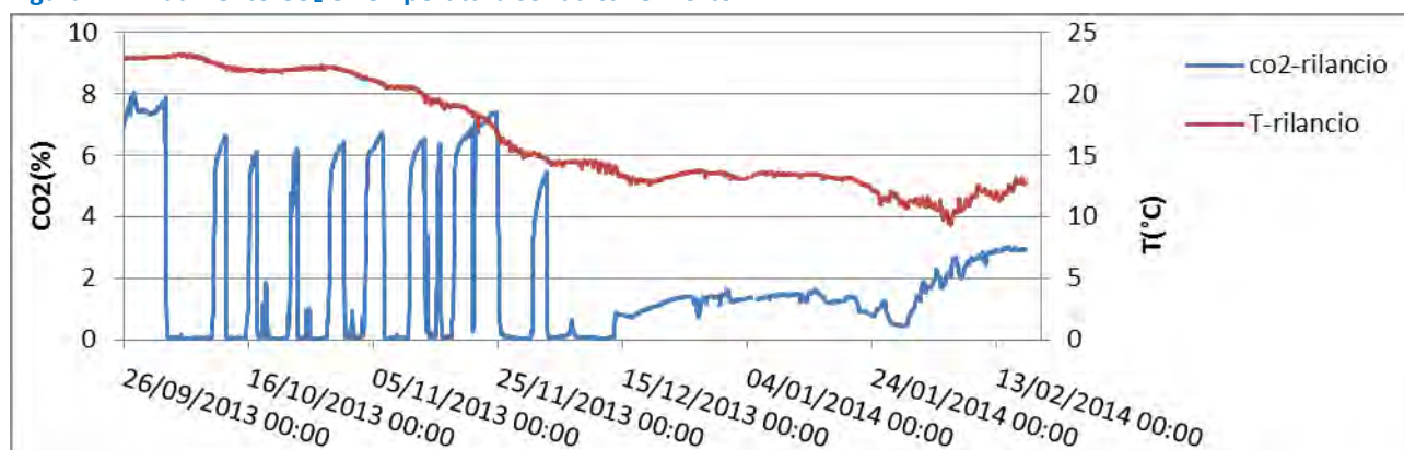
Figura 18. Andamento CO 2 e Temperatura sonda rilancio
