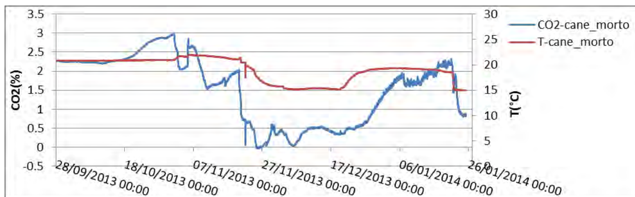
Figura 17. Andamento CO 2 e Temperatura sonda cane morto
