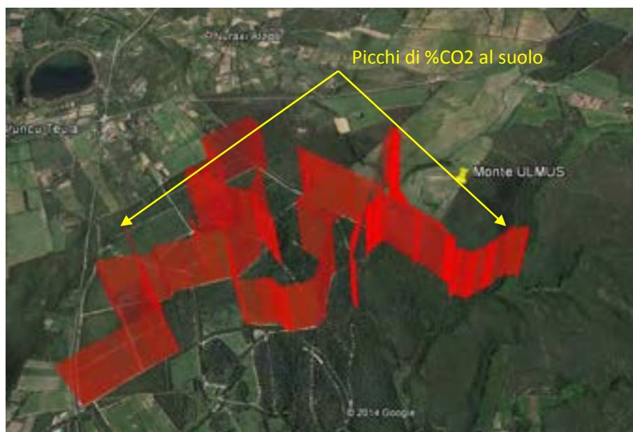
Figura 6 – Profilo della concentrazione della CO2 dal suolo in una zona di rimboschimento
