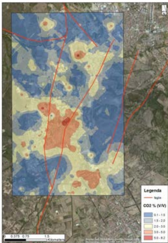
Figura 7 Contour map della CO 2 nella valle di Carbonia.
