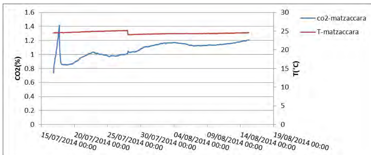
Figura 24. Andamento CO 2 e Temperatura sonda matzaccara
