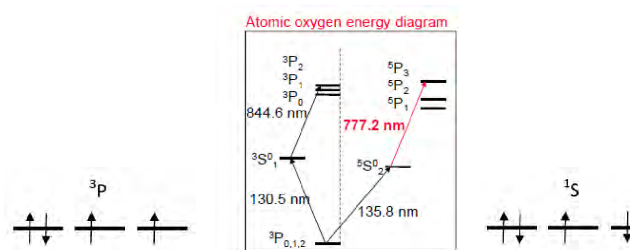
Fig 2 Configurazione elettronica dell'ossigeno atomico nello stato fondamentale (a sinistra) e schema dei livelli energetici che danno luogo alle righe spettrali (777.2 nm e 844.6 nm) nell'ossigeno atomico (a destra).
