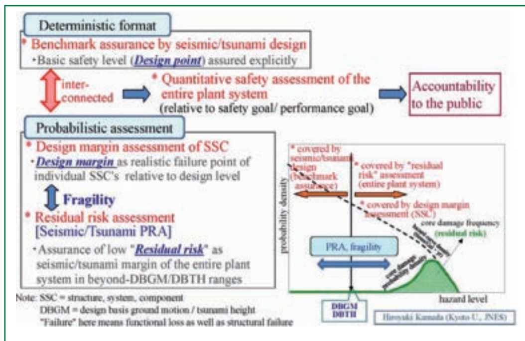
Schema per verifiche di sicurezza sismica/tsunami (safety)
