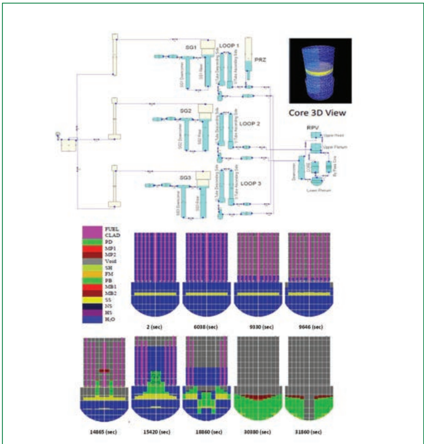
Nodalizzazione MELCOR di un generico reattore da 900 MW e analisi delle diverse fasi di degradazione del core predette dal codice MELCOR
