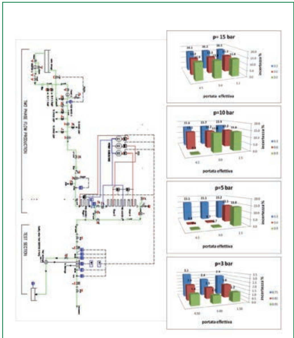
Schema di flusso strumentato dell'impianto di prova SPOOL PIECE e andamento dell'incertezza estesa della portata massica bifase in % al variare della pressione
