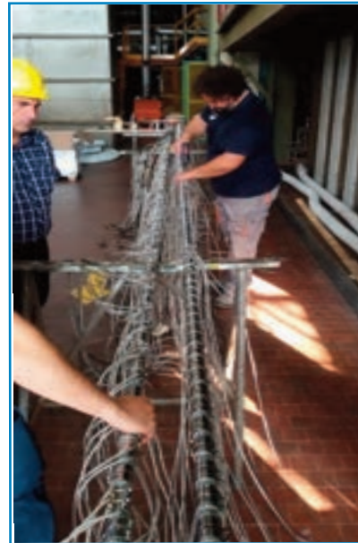
Resistenze scaldanti nell'apparecchiatura SIET HERO
