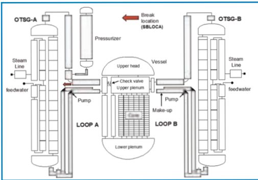
ASTEC
