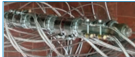
Resistenze posizionate su diversi angoli azimutali per ricostruire un flusso termico il più possibile simile a quello di generazione uniforme (dettagli)
