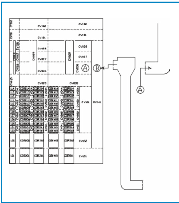
MELCOR
