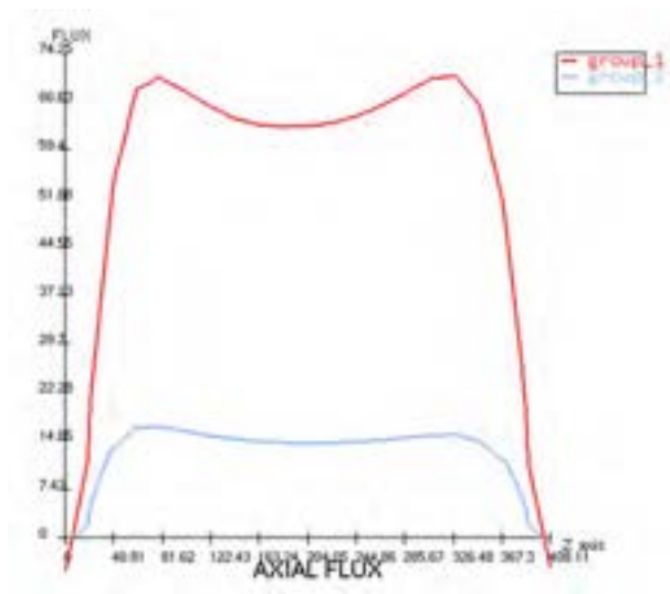
Fig. 31: Profilo assiale di flusso (u.a.) al centro del nocciolo a EOC (ARO).
