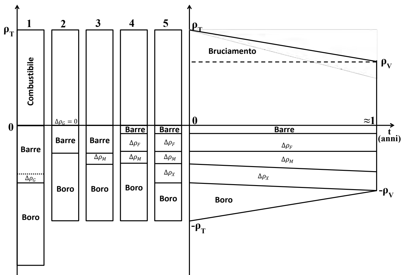
Figura 6: Schema del bilancio di reattività.
