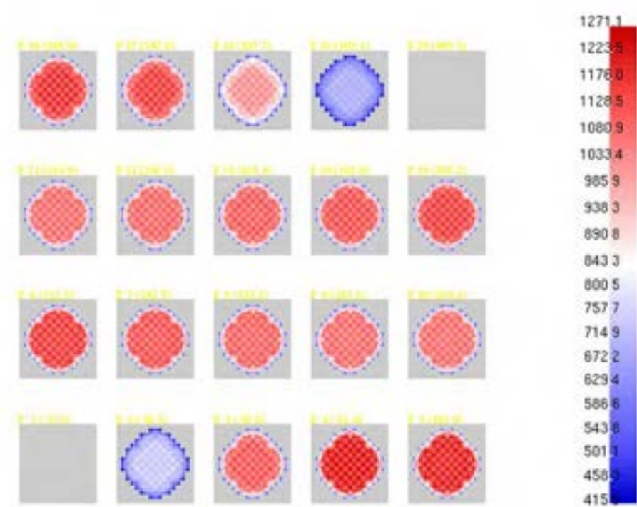
Figura 18: Distribuzione di temperatura center line (°C) a EOC (ARO).
