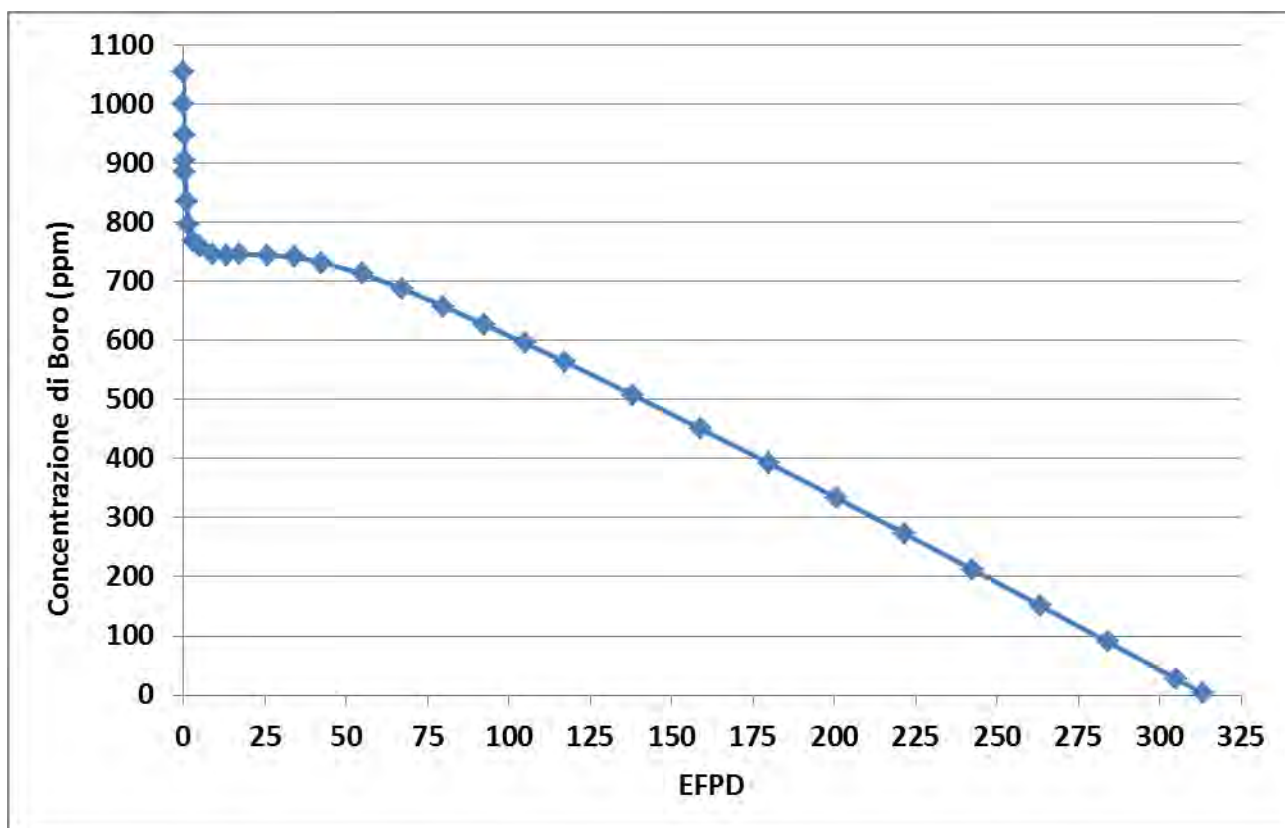
Figura 8: Curva di letdown del boro (ARO).
