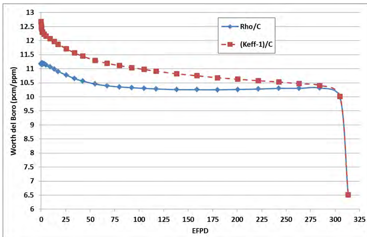
Figura 9: Worth del boro all'aumentare del bruciamento (ARO).
