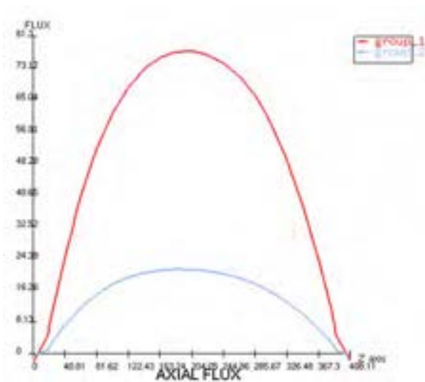
Fig. 30: Profilo assiale di flusso (u.a.) al centro del nocciolo a BOC (ARO).
