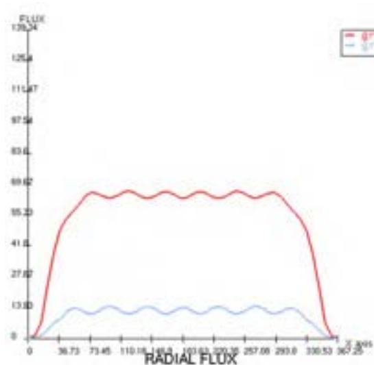
Fig. 29: Profilo radiale di flusso (u.a.) nel piano di mezzeria a EOC (ARO).
