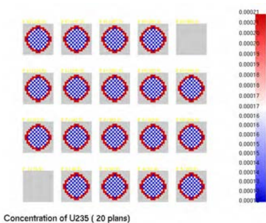
Figura 21: Distribuzione di U235 (#/b-cm) a BOC (ARO).
