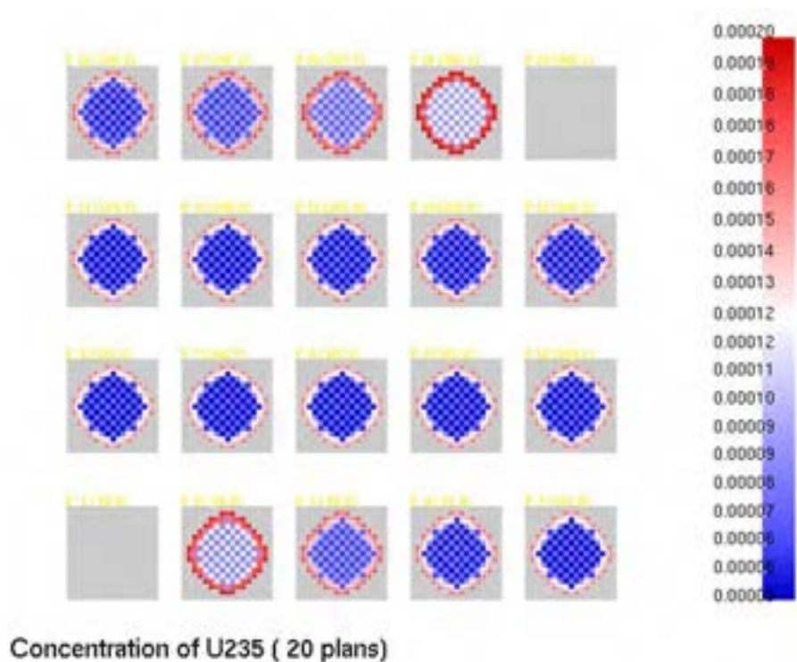
Figura 22: Distribuzione di U235 (#/b-cm) a EOC (ARO).
