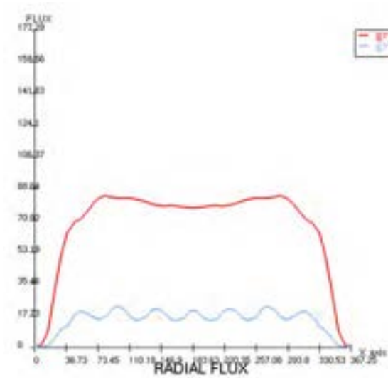
Fig. 28: Profilo radiale di flusso (u.a.) nel piano di mezzeria a BOC (ARO).
