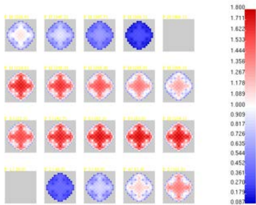
Fig. 45: Distribuzione del fattore di forma a BOC, HFP, con inserimento completo del gruppo G_18_G2.
