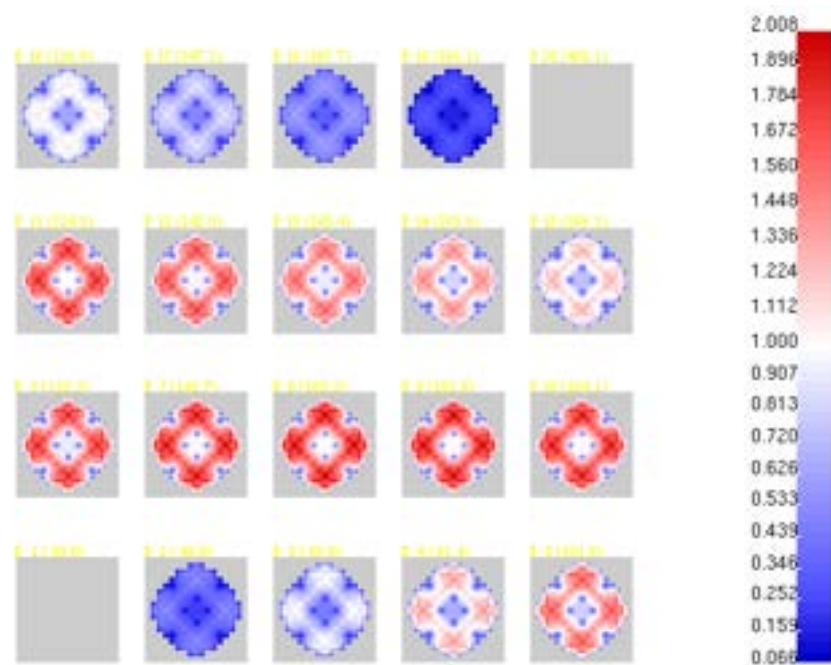
Fig. 46: Distribuzione del fattore di forma a BOC, HFP, con inserimento completo del gruppo G_18_N1.
