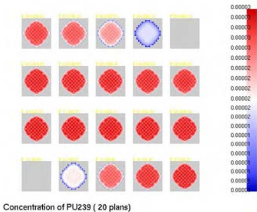
Figura 23: Distribuzione di Pu239 (#/b·cm) a EOC (ARO).
