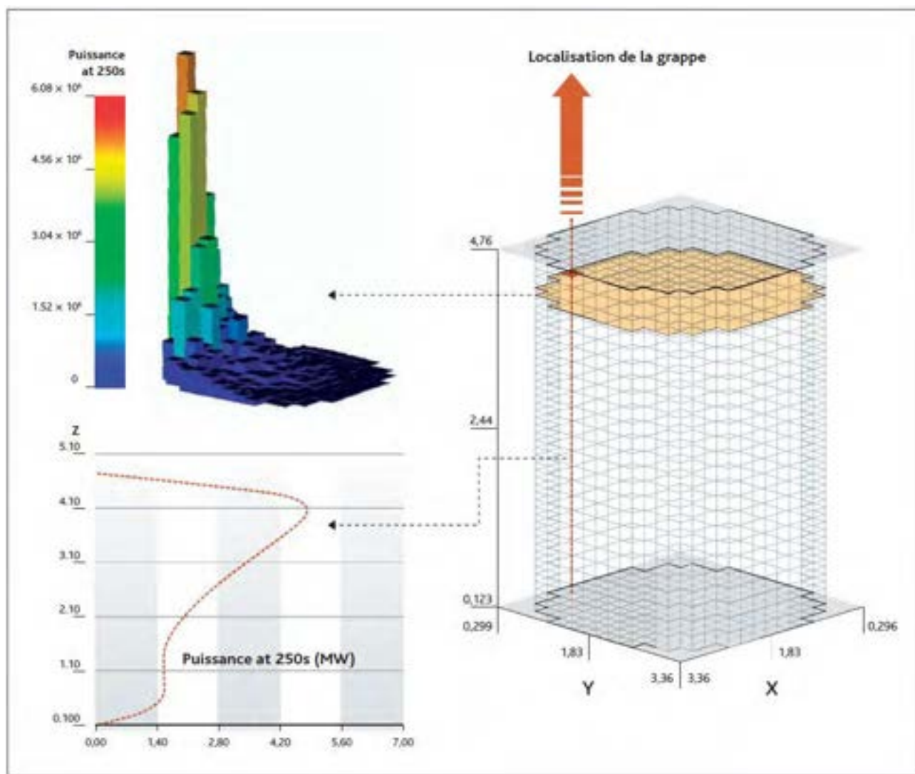
Figura 32. Distribuzione della densità di potenza a 250 s.
