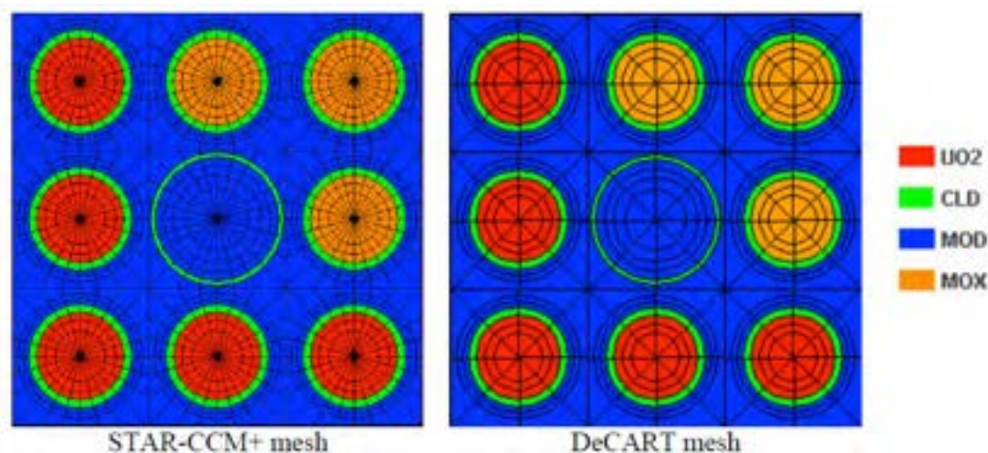
Figura 18. Discretizzazione spaziale di STAR-CCM+ e DeCART.
