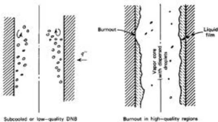
Figura 14. Fenomeni che portano al burnout della barretta.
