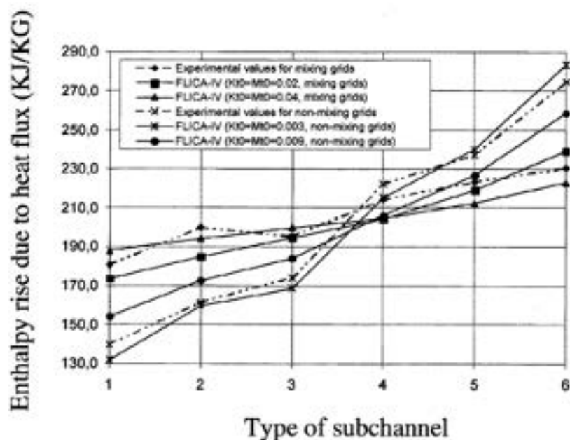
Figura 37. Confronto tra l'aumento di entalpia misurato e quella calcolata con FLICA4.
