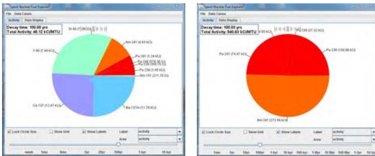
Figura 8 Attività dei U & Reactor-Grade Pu irraggiati, a 100 anni di decadimento
