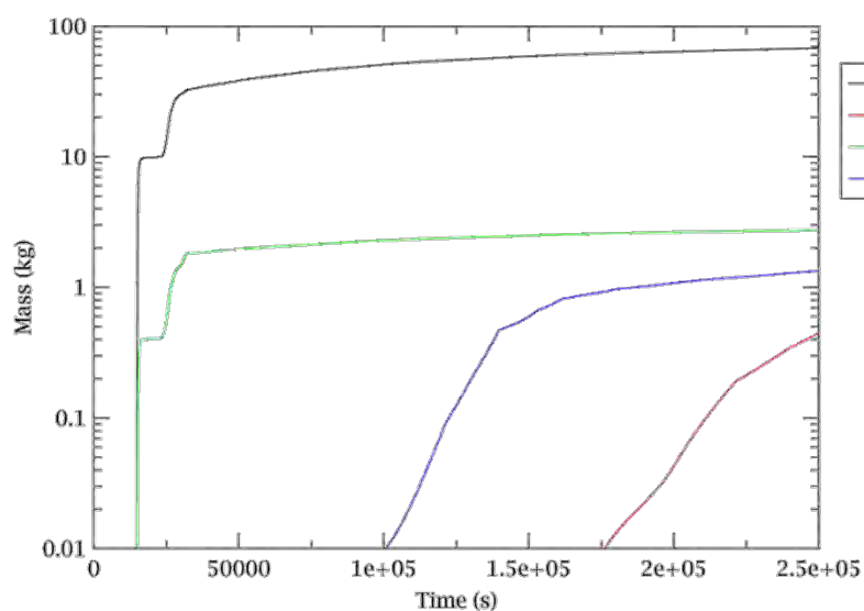
Figura 14: Masse di CS, I, Te che fuoriescono dal SRV del GV predette dal codice MELCOR.
