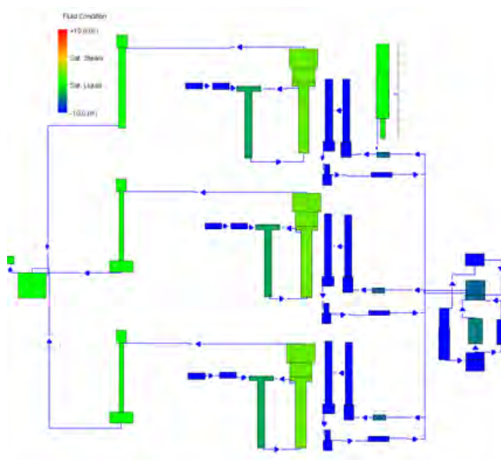
Figura 7: Visualizzazione delle condizioni termoidrauliche del fluido primario e secondario durante lo stazionario ottenuto con il codice MELCOR.
