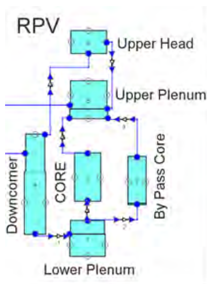
Figura 5: Nodalizzazione MELCOR del vessel del reattore di riferimento.
