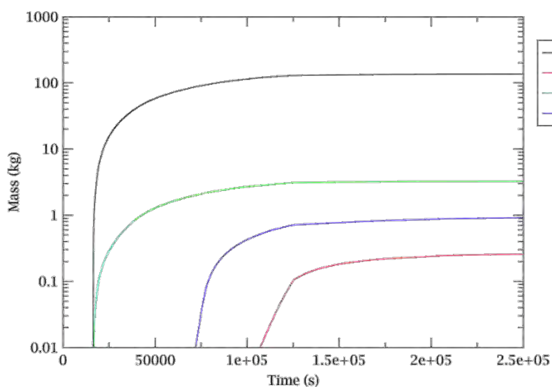
Figura 15: Masse di CS, I, Te che fuoriescono dal contenimento predette dal codice MELCOR.
