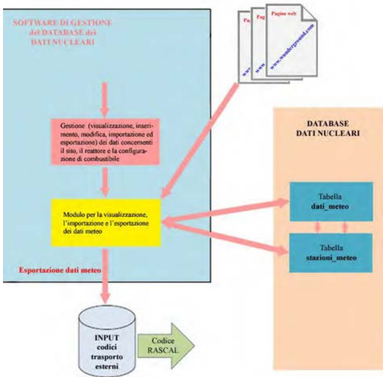
Figura 8 – Schema di funzionamento del sistema di acquisizione dati in tempo reale
