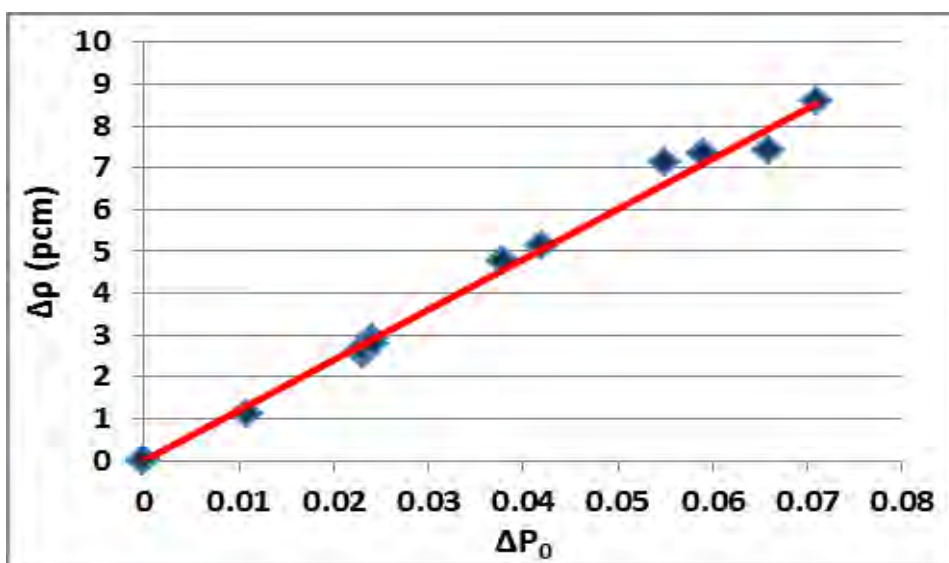
Fig. 9. Differenza del valore di antireattività al variare di \Delta P_0 .
