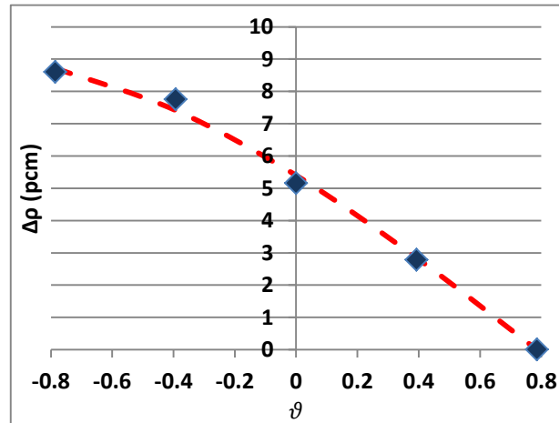
Fig. 11. Differenza di worth tra barre di controllo esterne simmetriche come funzione dell'azimut.
