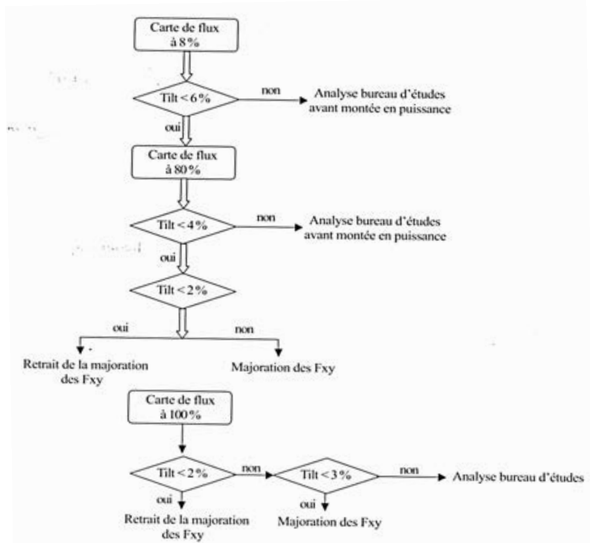
Fig. 3. Diagramma di flusso sul monitoraggio del tilt in fase di avviamento del reattore.
