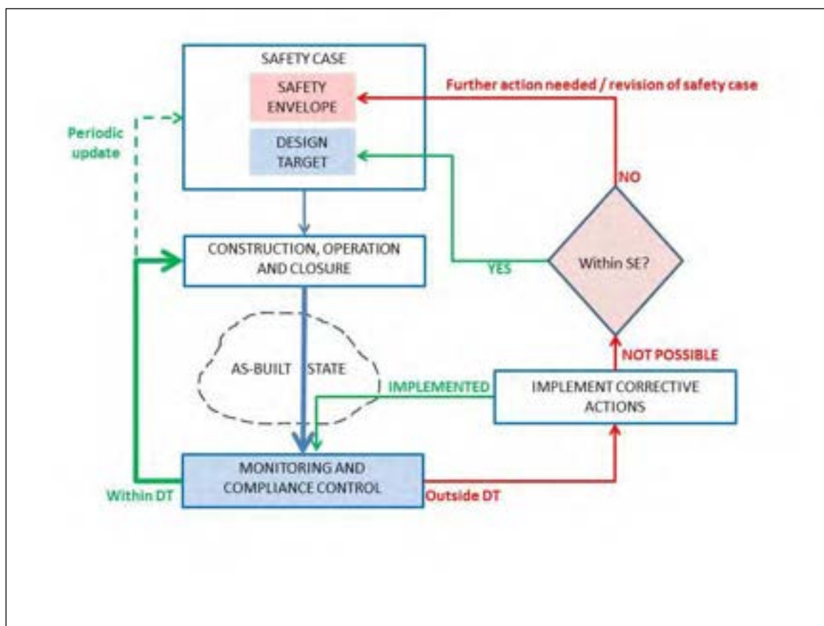
Figura 5 – Schema di flusso per le analisi di sicurezza durante la realizzazione e l'esercizio del deposito.
