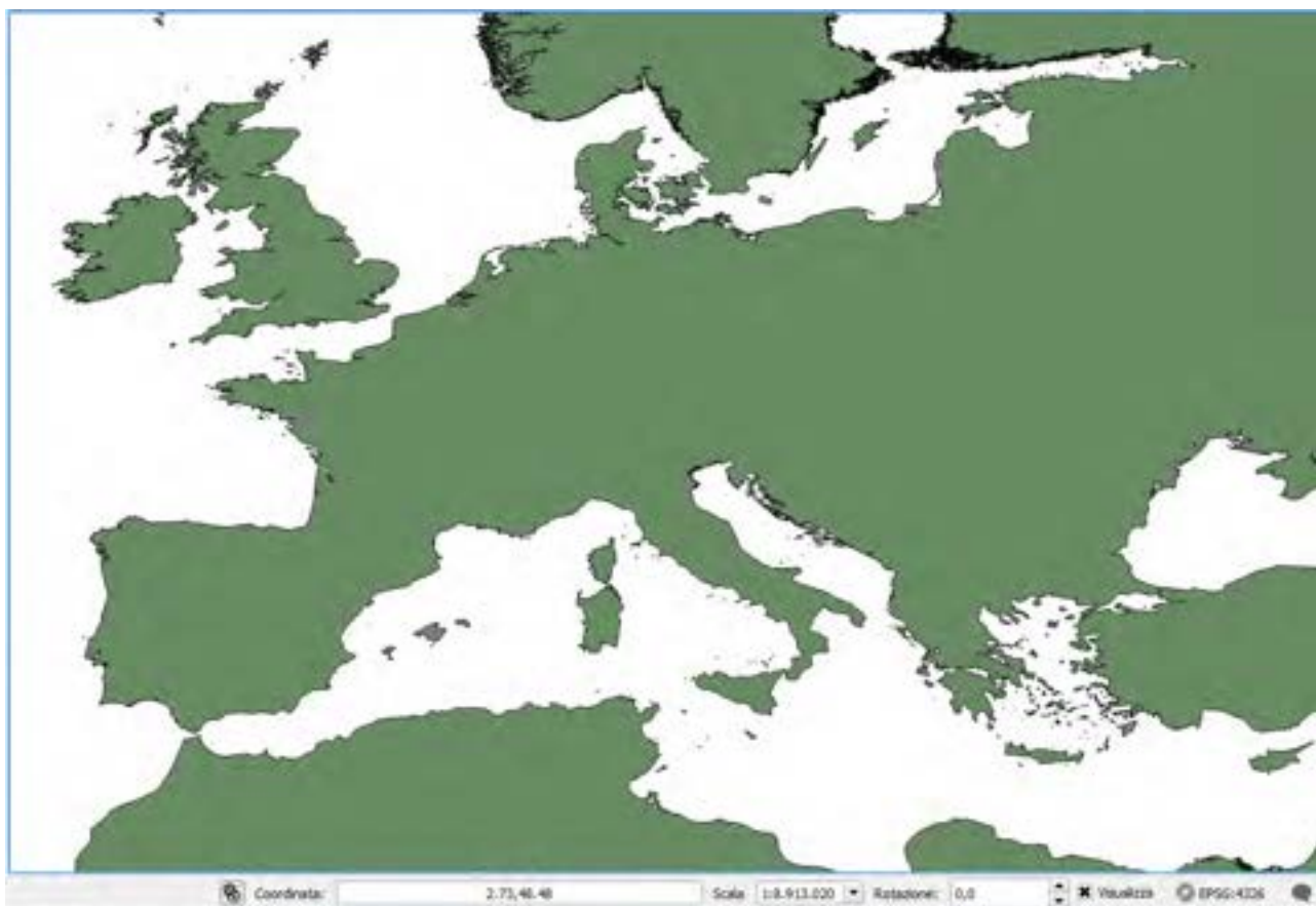
Fig. 5 – Rappresentazione QGIS del file relativo alla caratterizzazione dei dati riguardanti le linee di costa e dei corpi d'acqua
