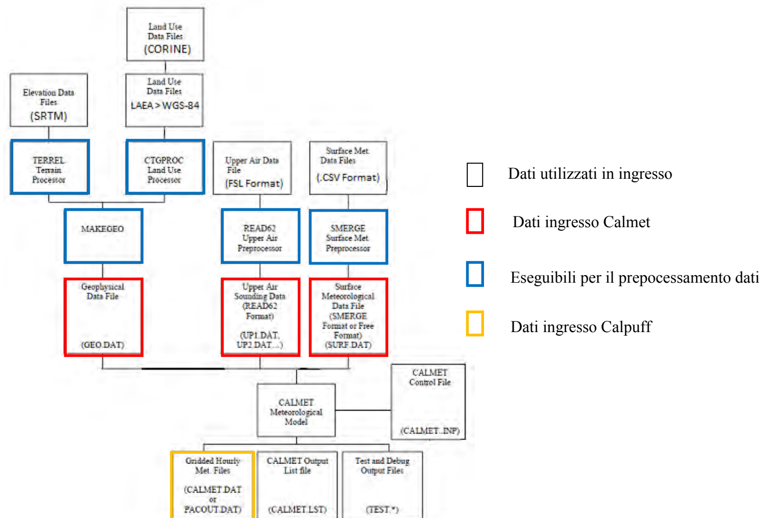
Fig. 2 - Flow Chart dei pacchetti di pre-processamento impiegati nella procedura messa a punto nell'ambito dell'attività di ricerca.
