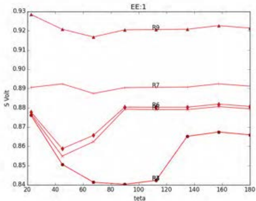
Fig. 20: Esempio di profili sperimentali ottenuti con l'eccitazione dell'elettrodo 1 e la lettura degli elettrodi residui ( R=2,9 ); ( \theta = 0 ).
