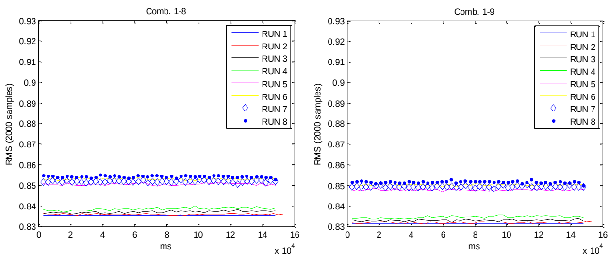
Fig. 21: Andamento temporale segnali sonda ECP – Prove dinamiche – Combinazioni elettrodo 1 – 2,9
