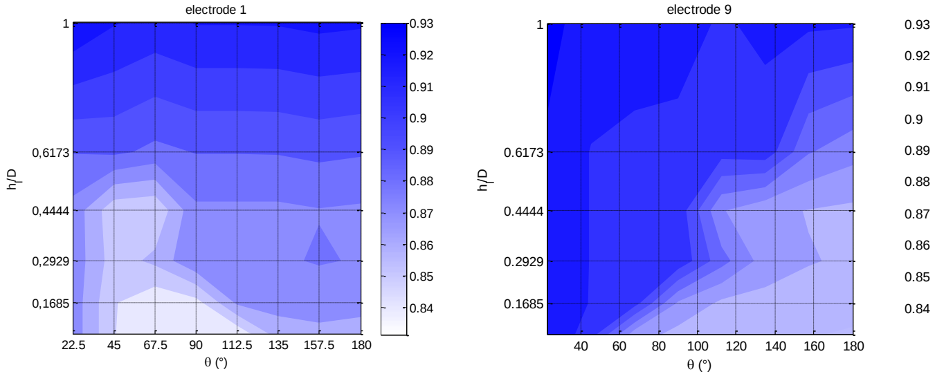
Fig. 18: Segnali medi sonda ECP V = f(\theta, h_i) – Prove statiche
