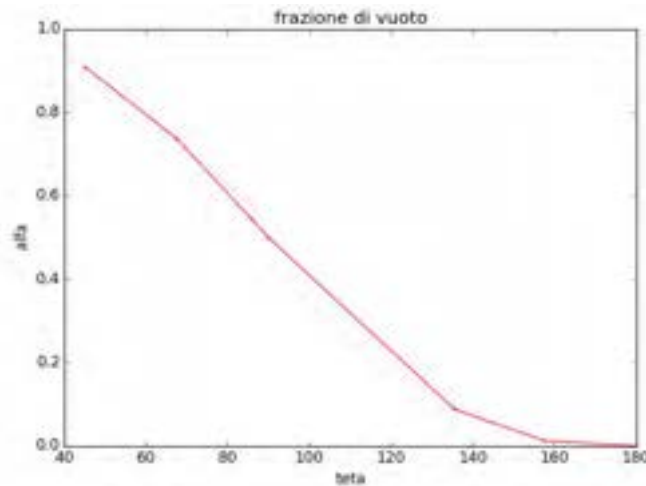
Fig. 16 Andamento della frazione di vuoto in funzione del semi angolo di bagnabilità (teta = 0)
