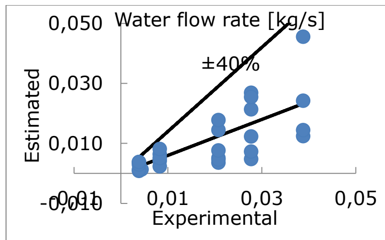
Fig. AD-2: Confronto tra le portate sperimentali e stimate per la fase liquida
