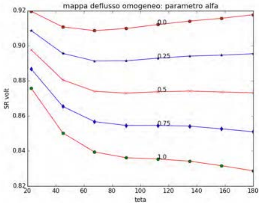
Fig. 19: Mappa della sonda ECP, relativa agli elettrodi esterni per alcuni valori della frazione di vuoto ( \theta = 0 ).
