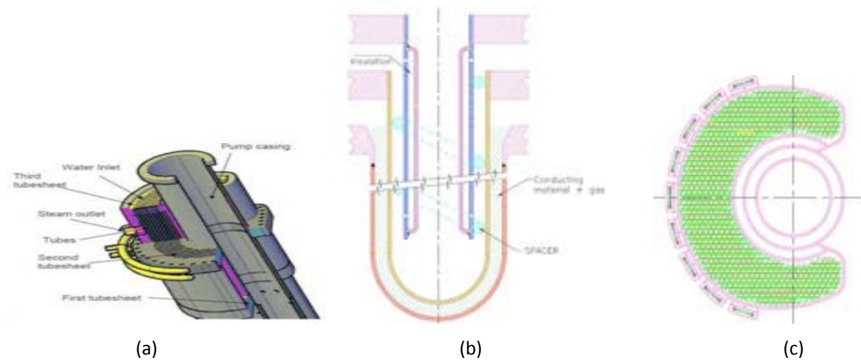
Figura 6. - Schema dello scambiatore di calore di tipo a baionetta che si pensa di utilizzare nell'impianto dimostrativo ALFRED.
