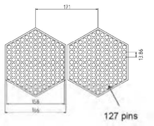
Figura 3 Fuel Assembly - nocciolo di ALFRED
