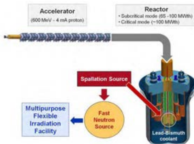
Figura 10 Schema Reattore MYRRHA
