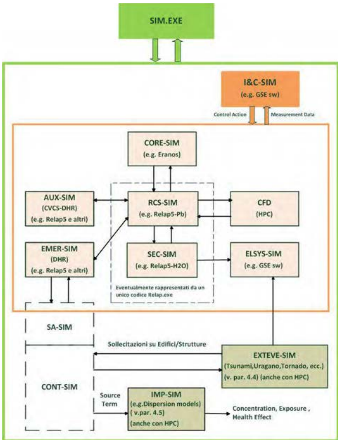
Figura 45 Possibile Architettura di Piattaforma di Simulazione Ingegneristica
