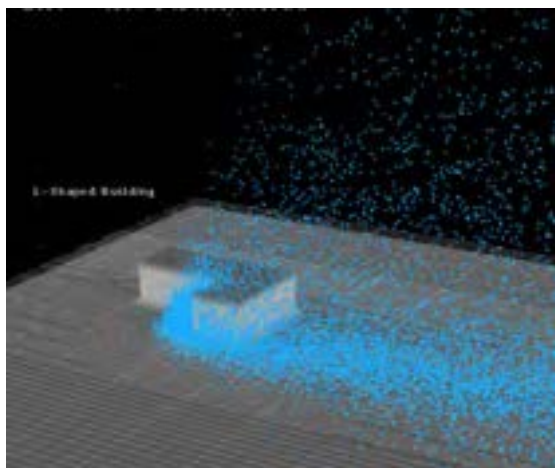
Figura 38 Visualizzazione di un pennacchio simulato da un modello lagrangiano “a particelle” (sinistra), emesse all’interno di un ostacolo a forma di “L” e trasportate dietro l’ostacolo stesso e corrispondenti involucri tridimensionali di concentrazione superiore a due differenti soglie (destra).
