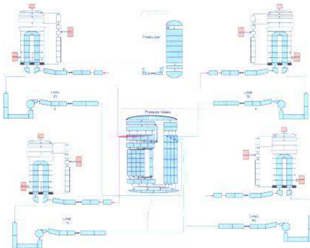
Figura 28 Il modello del reattore a quattro loop secondo la piattaforma RELAP5-HD
