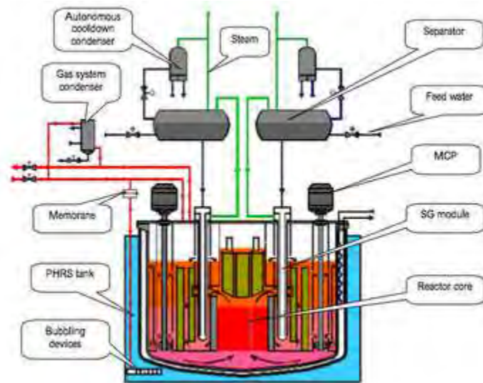
Figura 9 Sezione verticale Reattore SVBR 75
