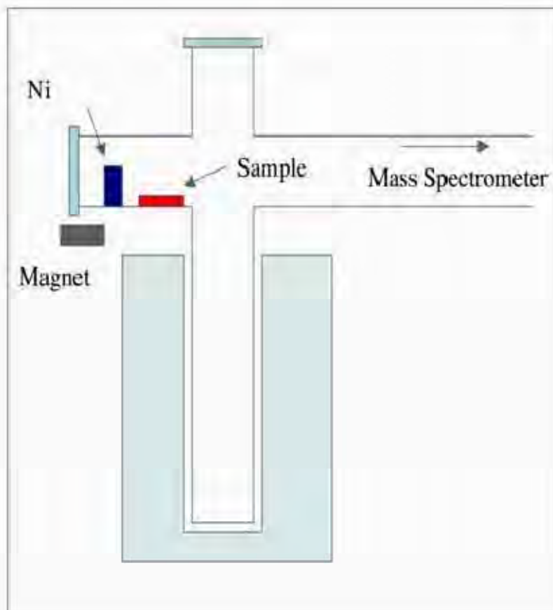
Fig. 1e : Area di stoccaggio e desorbimento del campione.
