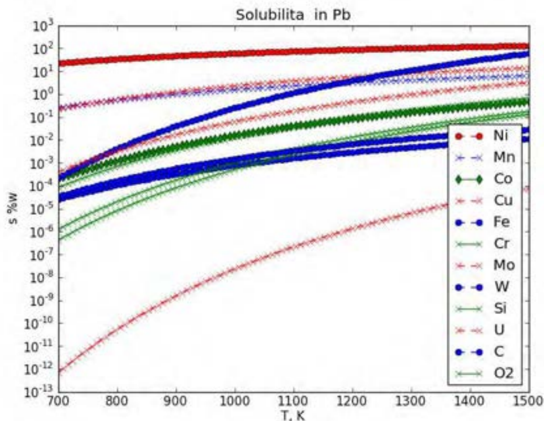
Figura 15 Solubilità di diverse specie chimiche in piombo (% wt)
