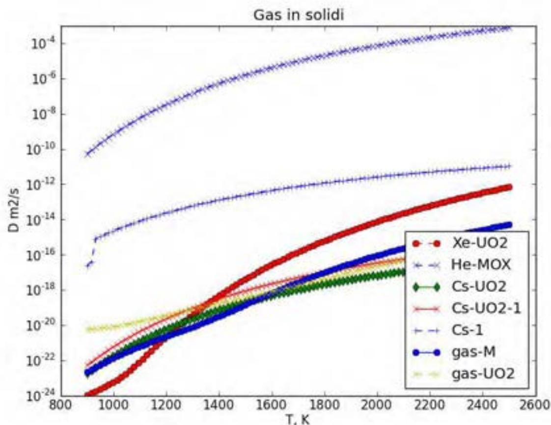
Figura 9 Coefficienti di diffusione di alcuni prodotti di fissione volatili in combustibili ceramici e metallici (Xeno,elio, Cesio, gas (G) in matrici metalliche M)
