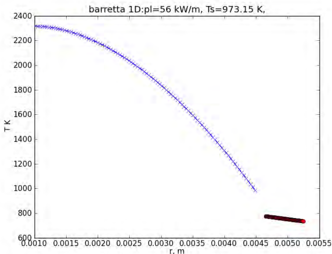
Fig. A1 Profilo di temperatura nella pastiglia e nella guaina stimato in condizioni stazionarie.
