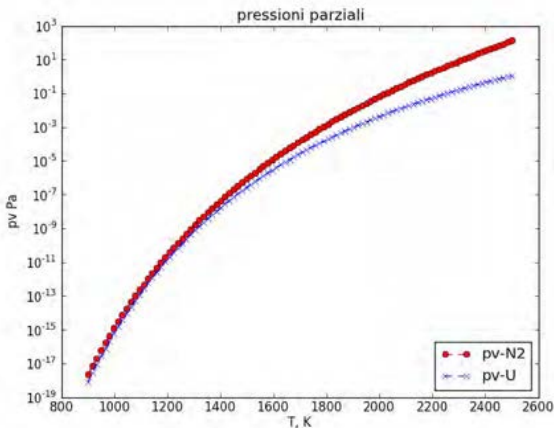
Fig. 7 Pressioni parziali dei vapori di azoto ed uranio in funzione della temperatura generate dal nitrato d'uranio.
