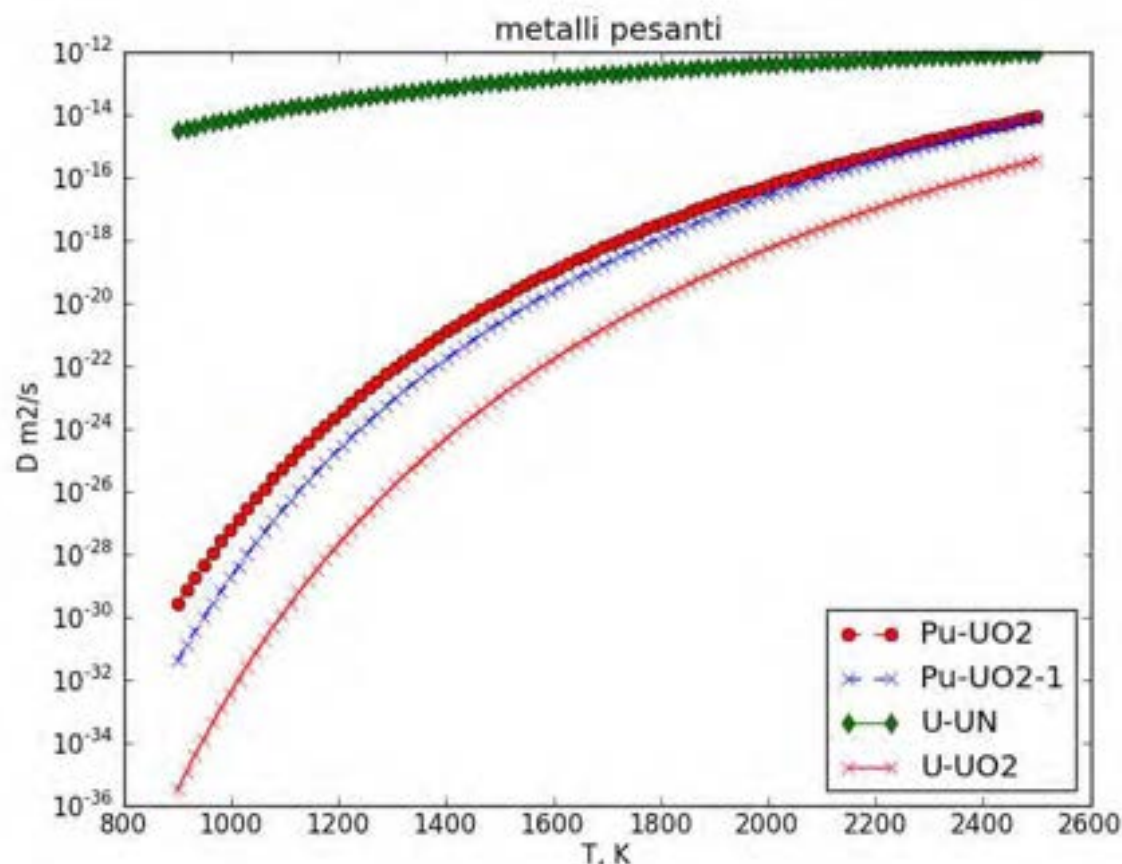
Figura 8 Coefficienti di diffusione per il plutonio e l'uranio nei combustibili in funzione della temperatura.
