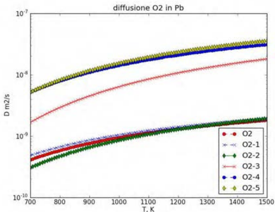
Figura 12: Coefficiente di Diffusione dell'Ossigeno in piombo (confronto tra correlazioni)
