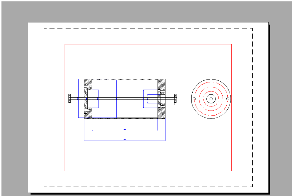
Fig. 1a Sezione di prova :Camere di misura
