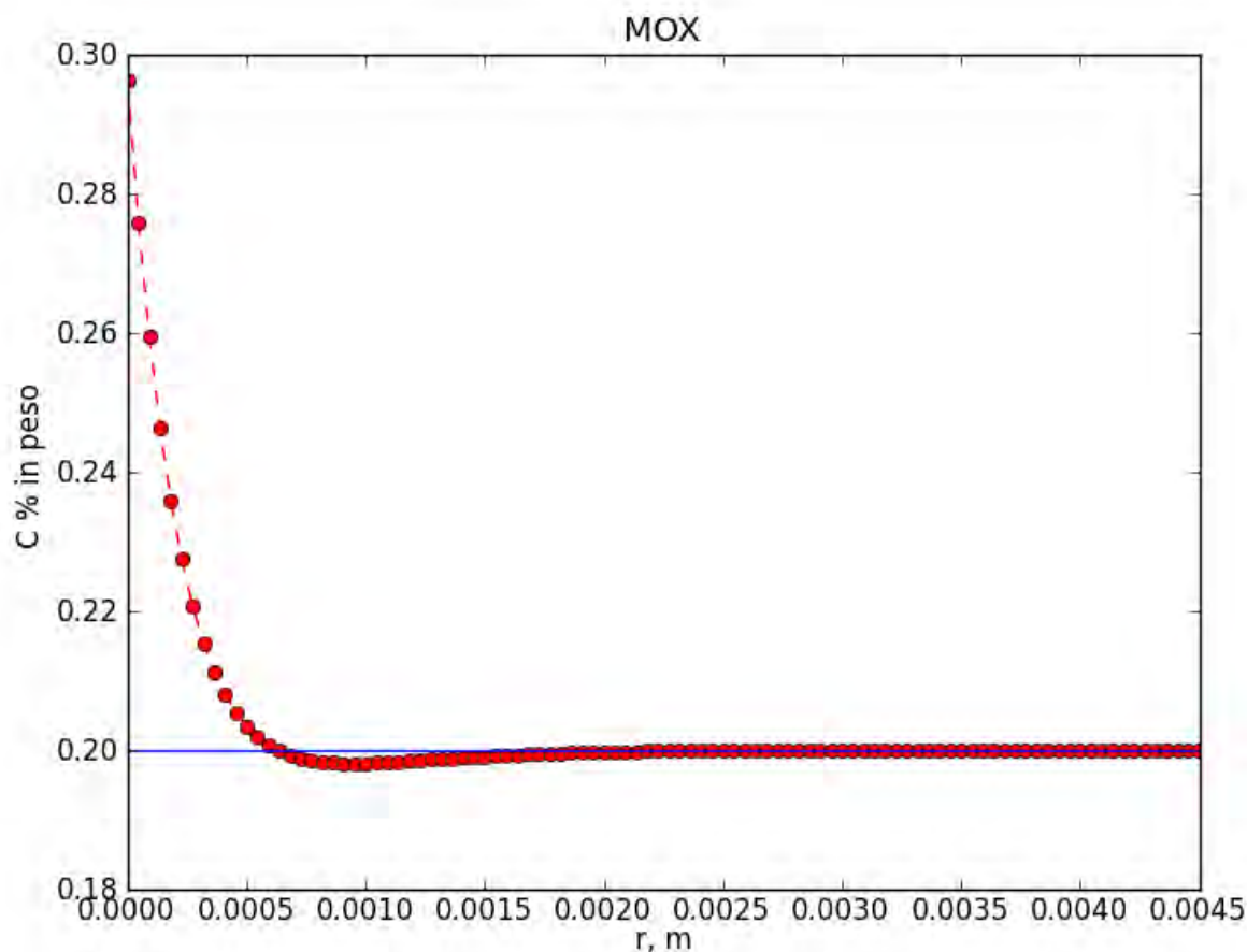
Fig. 2b: Ridistribuzione del plutonio (relazione empirica di Olander [16])
