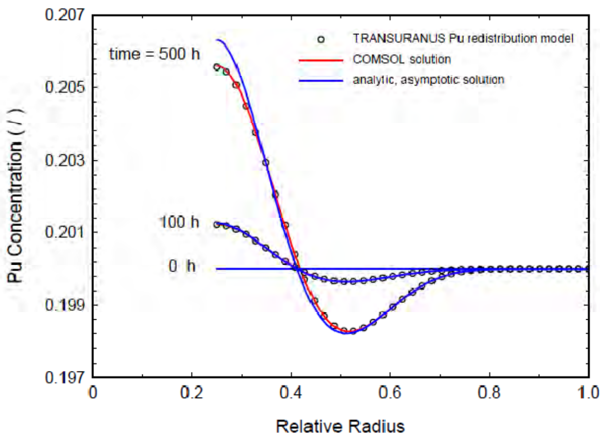
Fig. 2a Ridistribuzione del Plutonio valutata con diverse metodologie da Di Marcello et al [18].
