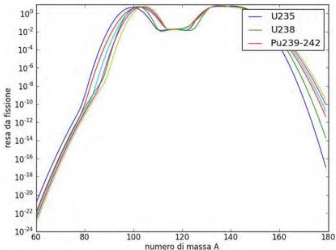
Figura 6. Rese di fissione stimate per gli isotopi fissili presenti nei MOX (Modello Wahle, IAEA-TecDoc-1168 [8]).
