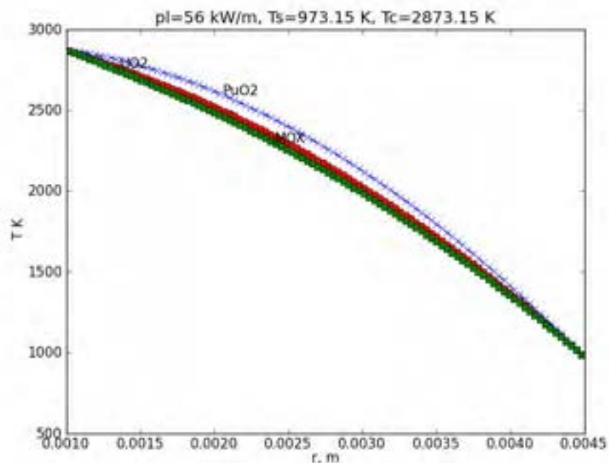
Figura 5b: Pastiglia cava con temperature imposte in corrispondenza del raggio interno ed esterno
