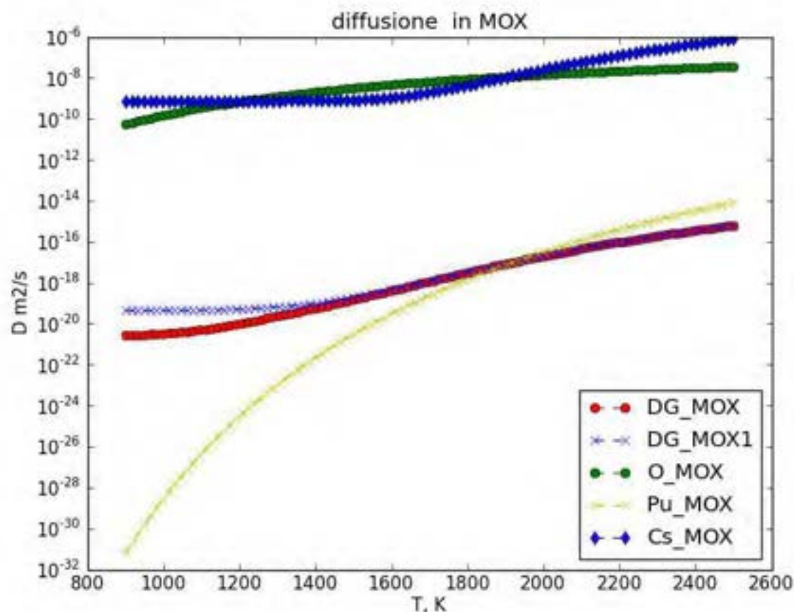
Figura 10 Coefficienti di diffusione in combustibili ad ossidi misti (Gas , ossigeno O, plutonio, Pu, Cesio Cs)
