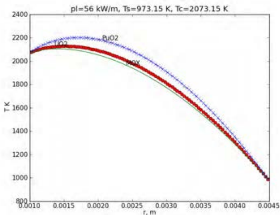
Figura 5c: Pastiglia cava con temperature imposte in corrispondenza del raggio interno ed esterno
