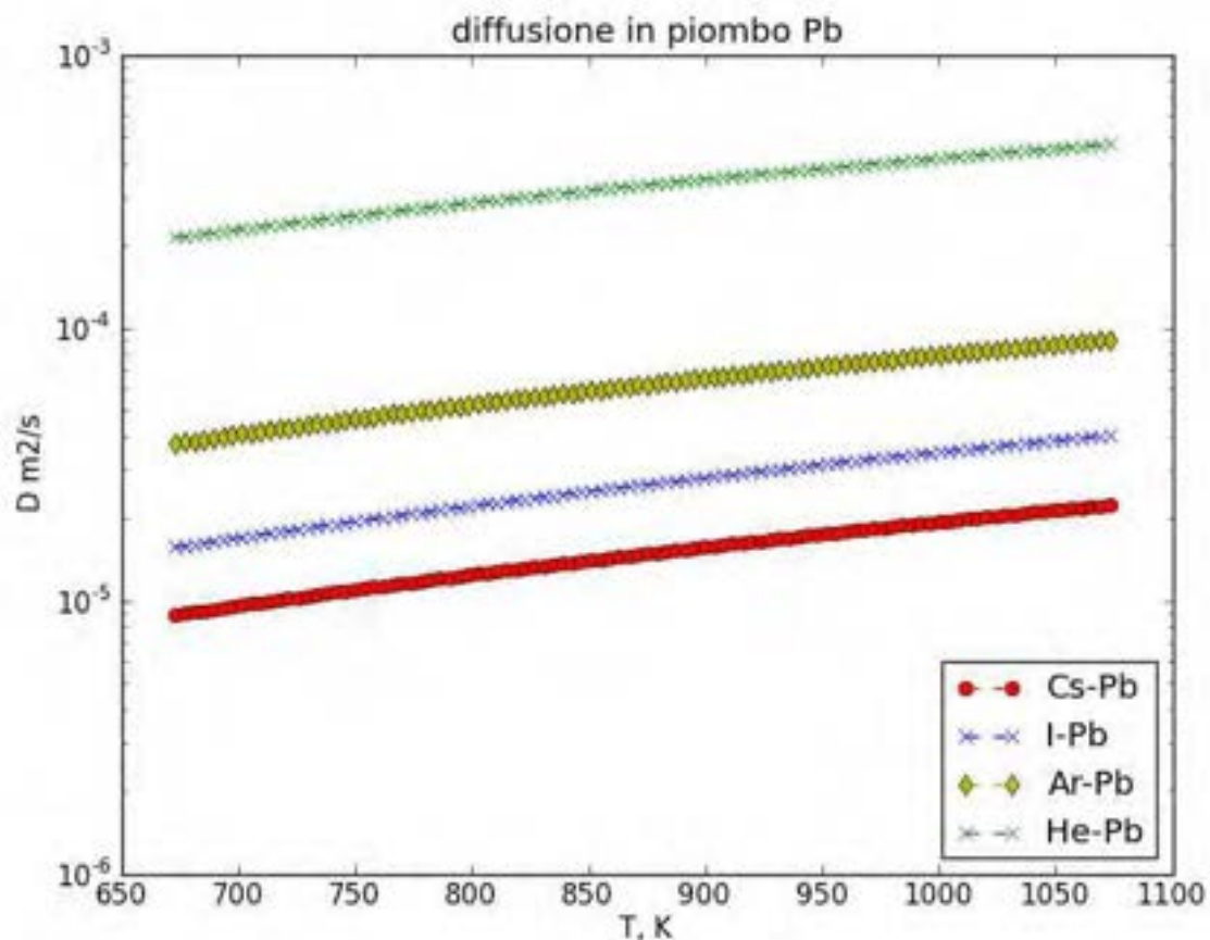
Figura 14a. Diffusione di alcune specie chimiche (Cesio, Iodio, Argon ed Elio) in Piombo (valori stimati)
