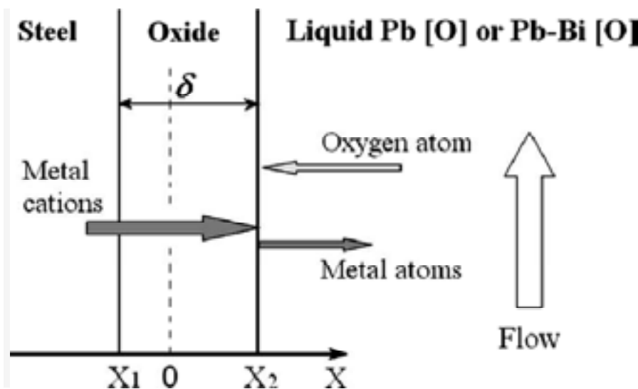
Figura. 66 Schematizzazione dei processi di corrosione/ossidazione.
