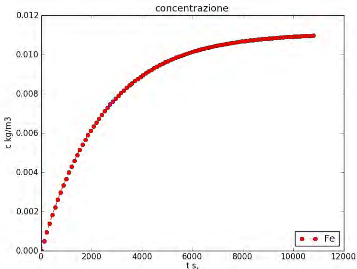
Figura 17 Evoluzione della concentrazione di una specie chimica (Ferro) in un metallo liquido stagnante (Sodio) inizialmente privo di ferro in soluzione.
