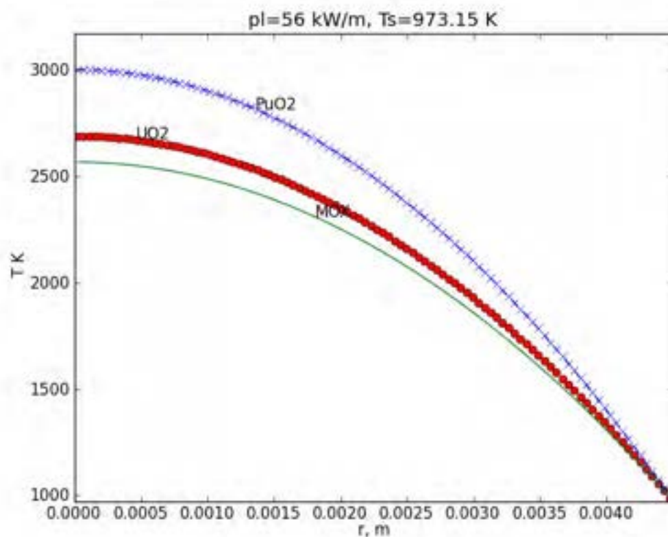
Figura 5a: Profilo di temperatura stimato con FiPy in un pastiglia non cava di raggio r=4.5 \text{ mm} . Temperatura di superficie T_s imposta
