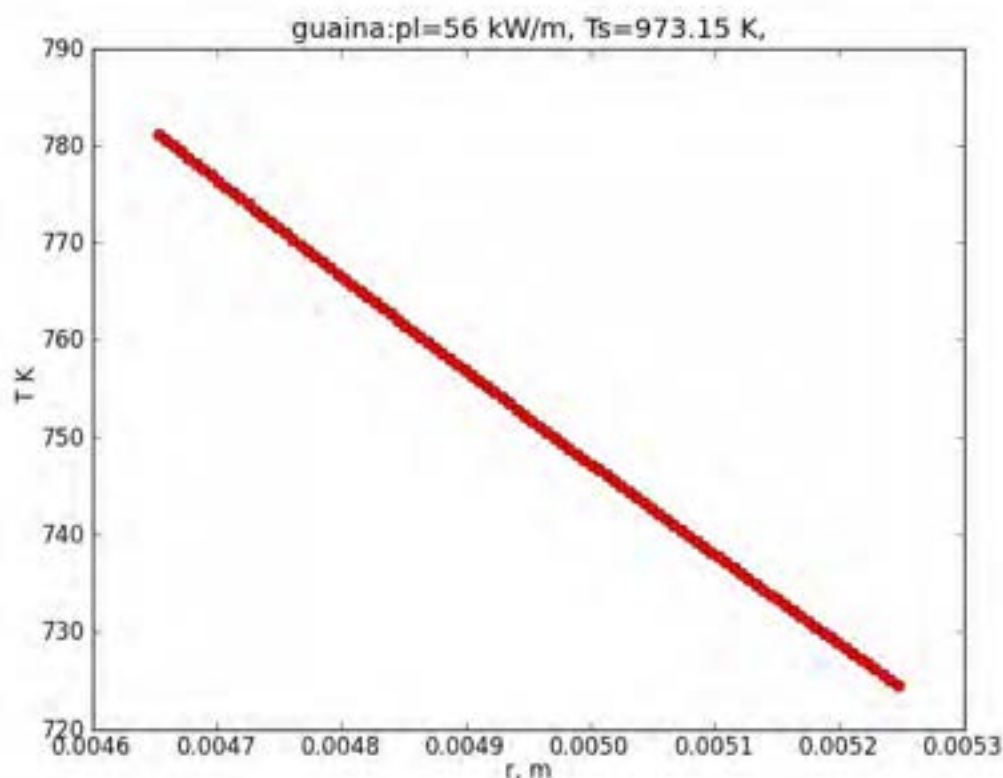
Figura 5e: Profilo di temperatura nella guaina in acciaio: Temperature di parete imposte
