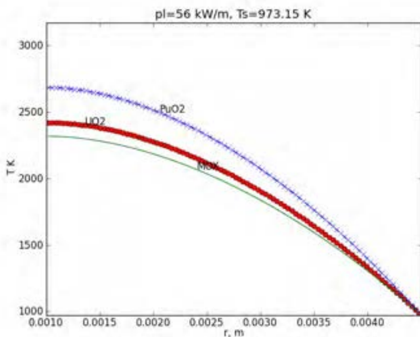
Figura 5d: Profilo stazionario di temperatura con imposti la temperatura di superficie T_s e flusso termico nullo in corrispondenza del raggio interno.
