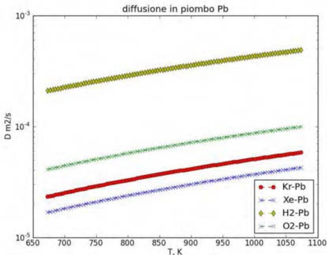
Figura 15b. Coefficienti di diffusione di alcune specie gassose (Krypton, Xeno, Idrogeno, Ossigeno) in Piombo (valori stimati).
