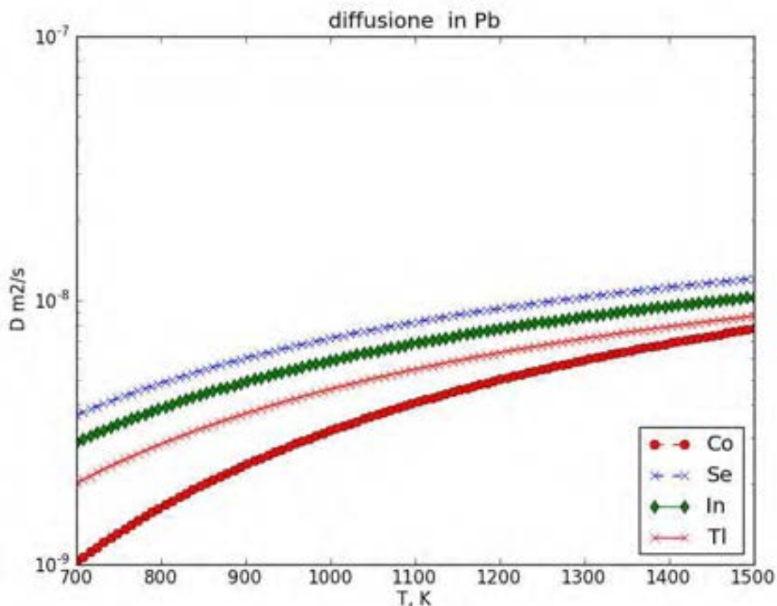
Figura 13: Coefficienti di diffusione di alcune specie chimiche in piombo.
