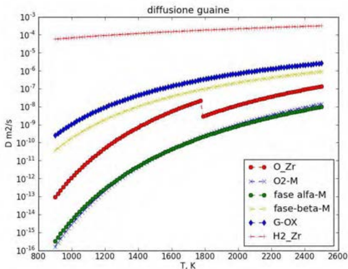
Figura 11 : Coefficienti di diffusione di specie chimiche gassose in guaine metalliche anche ossidate (Ox)
