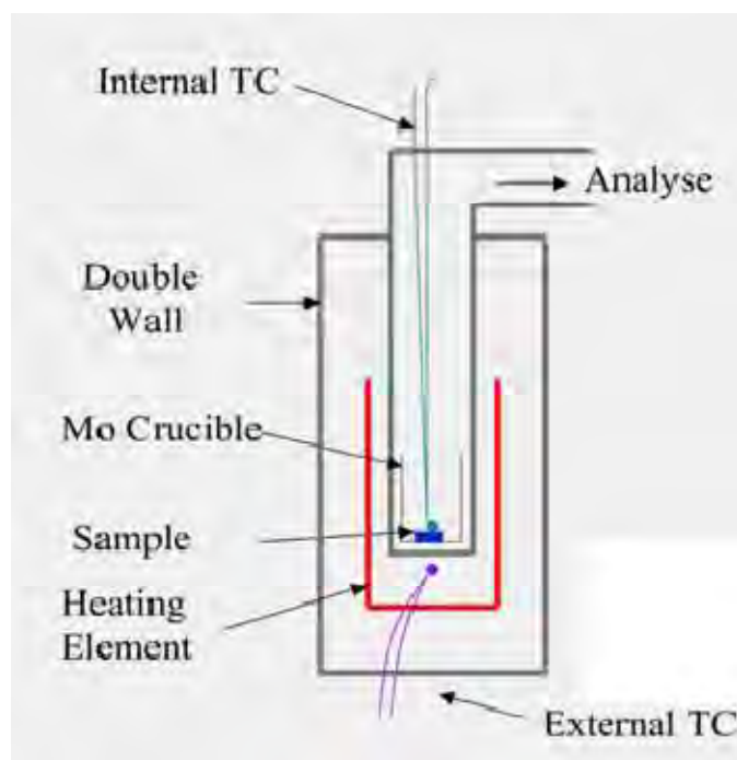
Fig. 1f Sistema di desorbimento ad alta temperatura
