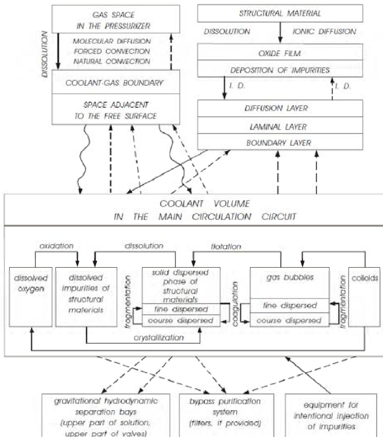
Fig. 4 Trasporti di massa in un circuito refrigerato con metallo liquido [20].
