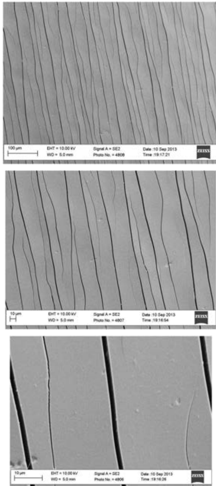
Figura 26. Micrografia SEM della superficie del campione spesso 5 µm e sottoposto ad elongazione pari al 6%.
