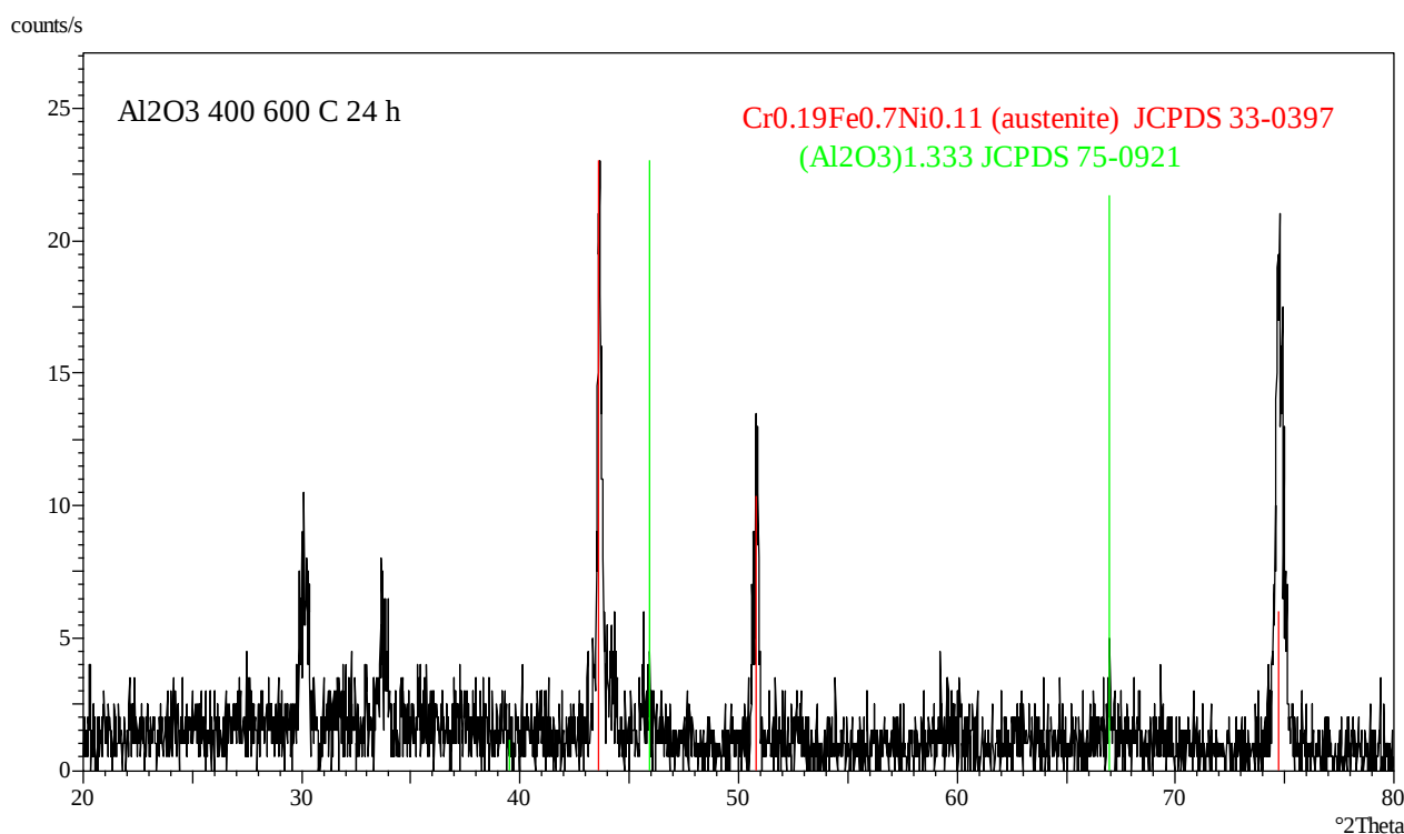
Figura 17. Pattern di diffrazione del campione Al 2 O 3 400 dopo trattamento termico a 600 °C per 24 h (rivestimento Al 2 O 3 depositato su 316L) acquisito utilizzando l'ottica thin film.
