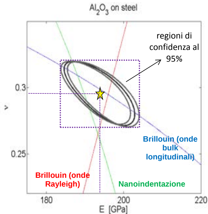
Figura 1. Rappresentazione nel piano E-v dei risultati delle misure di nanoindentazione e spettroscopia Brillouin, e la loro combinazione tramite uno stimatore che fornisce delle regioni di confidenza
