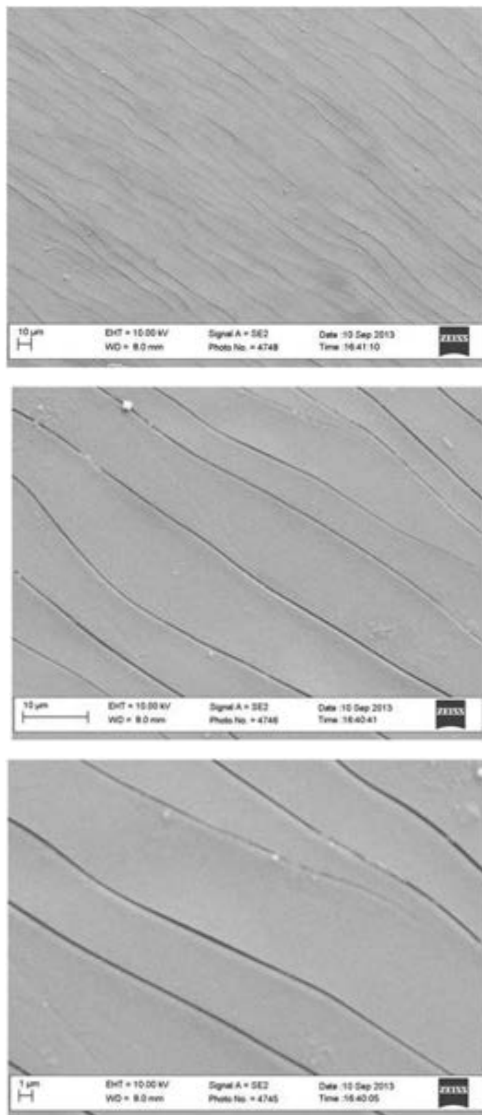
Figura 21. Micrografia SEM della superficie del campione spesso 1 \mu\text{m} e sottoposto ad elongazione pari al 3%.
