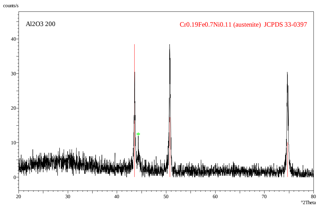
Figura 11. Pattern di diffrazione del campione \text{Al}_2\text{O}_3 200 (rivestimento \text{Al}_2\text{O}_3 depositato su 316L) acquisito utilizzando l'ottica thin film.
