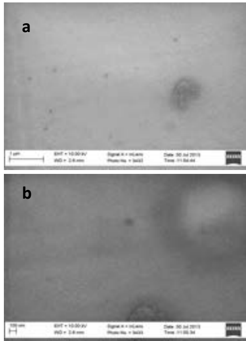
Figura 5. Micrografie SEM della superficie del rivestimento \text{Al}_2\text{O}_3 300 a) 50kx, b) 100kx.
