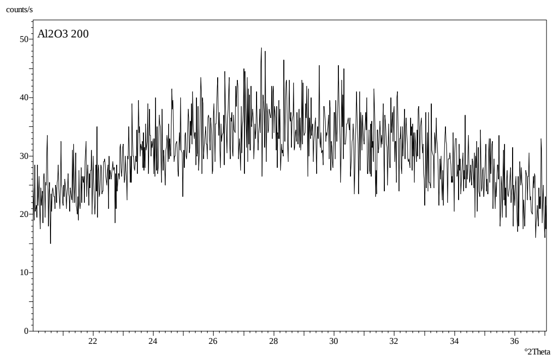
Figura 10. Pattern di diffrazione del campione \text{Al}_2\text{O}_3 200 (rivestimento \text{Al}_2\text{O}_3 depositato su 316L) acquisito utilizzando l'ottica delle polveri.
