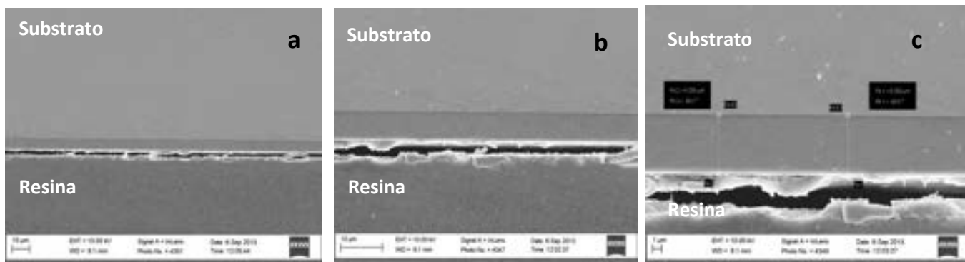
Figura 7. Micrografie SEM della sezione del rivestimento \text{Al}_2\text{O}_3 200 a) 2kx, b) 5kx, c) 10kx.
