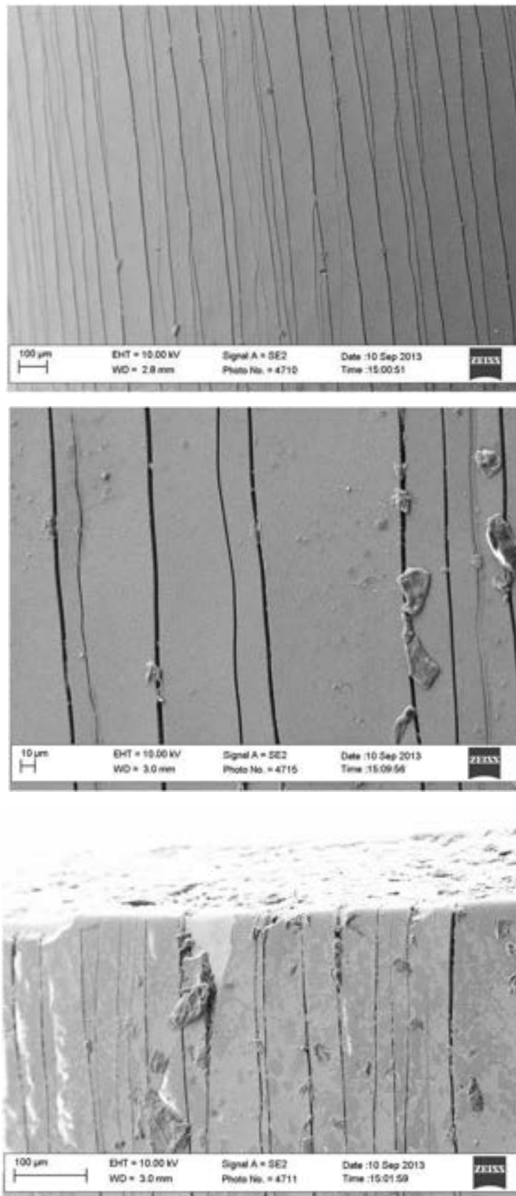
Figura 29. Micrografia SEM della superficie del campione spesso 10 µm e sottoposto ad elongazione pari al 6%.
