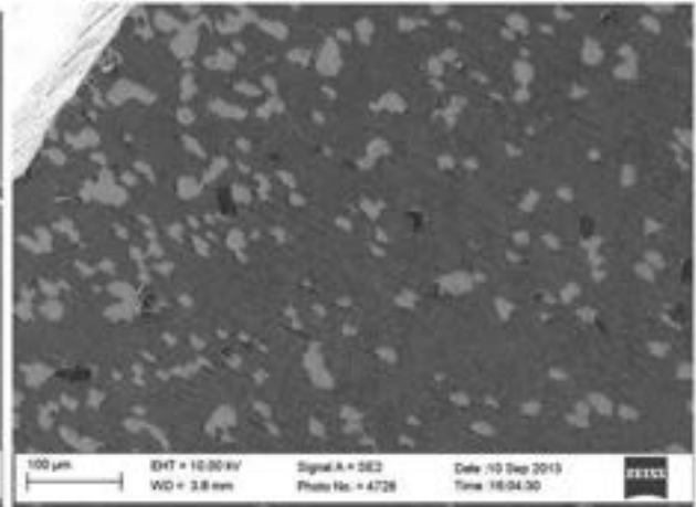
Figura 22. Micrografia SEM della superficie del campione spesso 1 \mu\text{m} e sottoposto ad elongazione pari al 6%.
