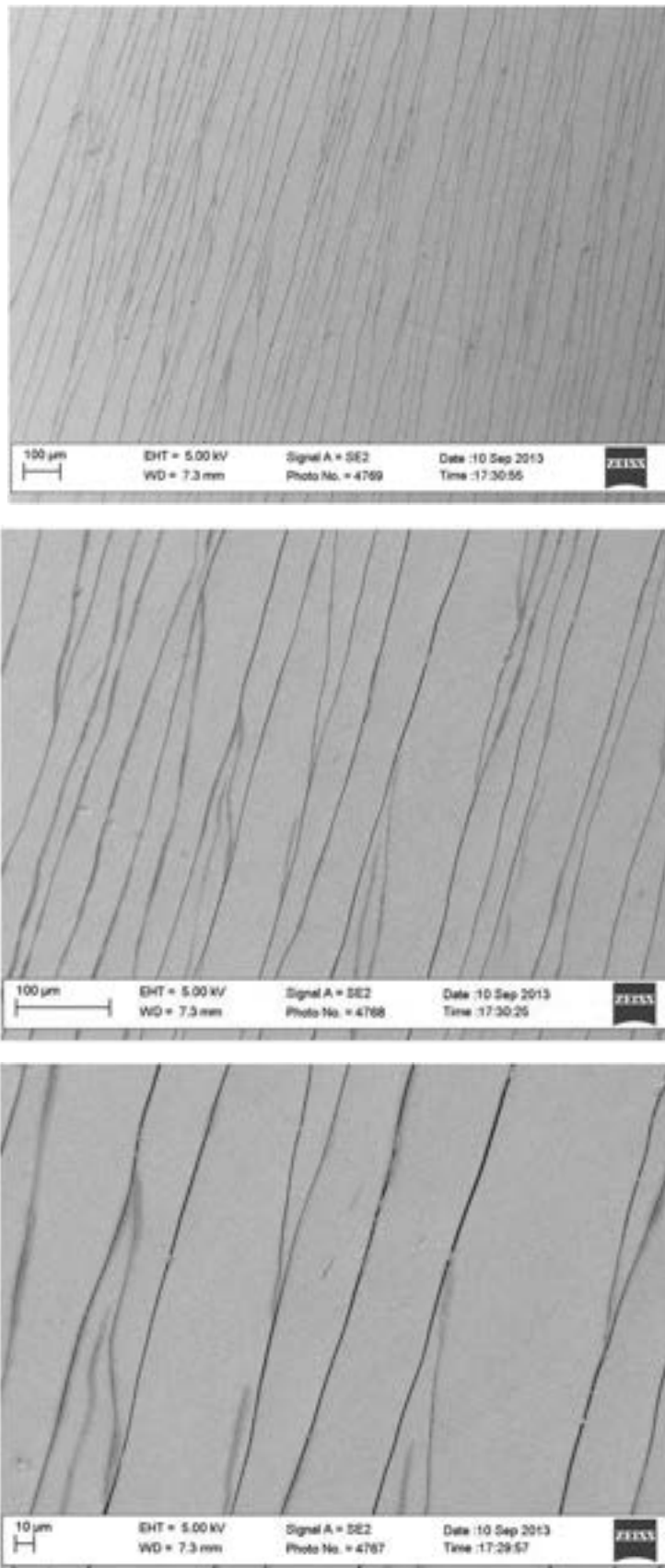
Figura 25. Micrografia SEM della superficie del campione spesso 5 µm e sottoposto ad elongazione pari al 3%.
