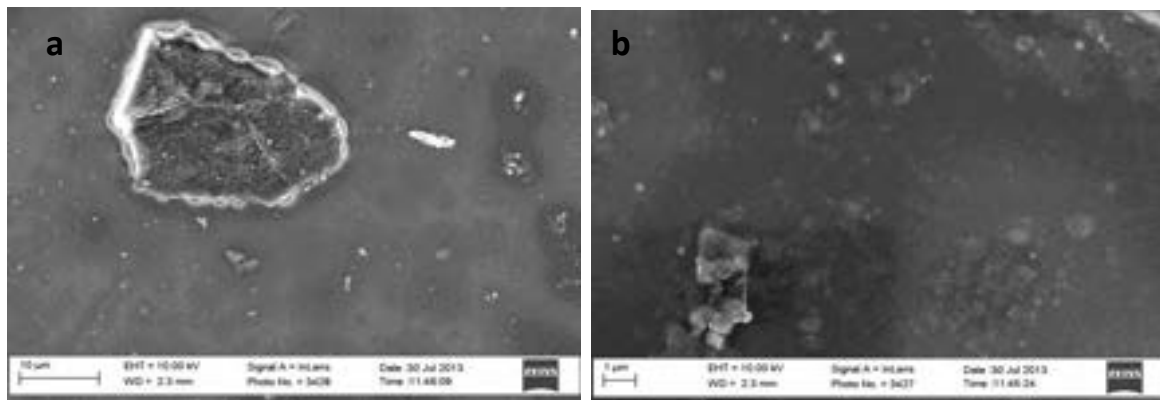
Figura 4. Micrografie SEM della superficie del rivestimento \text{Al}_2\text{O}_3 200 a) 5kx e b) 20kx.
