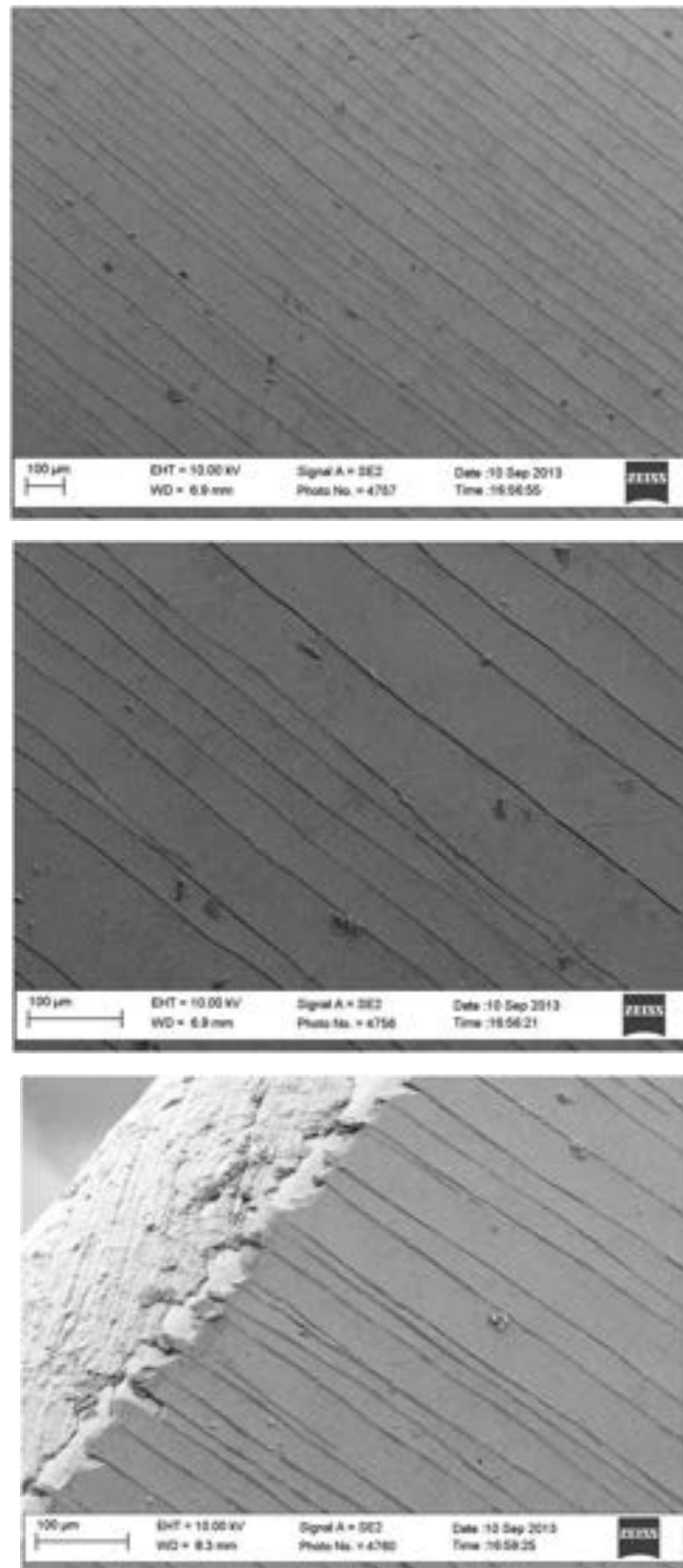
Figura 28. Micrografia SEM della superficie del campione spesso 10 µm e sottoposto ad elongazione pari al 3%.
