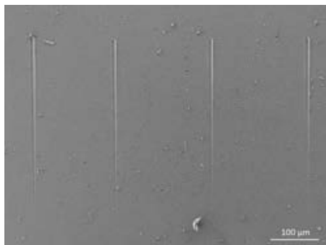
Figura 2. Immagine SEM della superficie dei rivestimenti di allumina dopo prove di nanoscratch (punta conica da 10 μm, carico massimo 500 mN). Non è stata osservata la delaminazione dei rivestimenti e, pertanto, non è stato possibile definire un carico critico per la delaminazione.
