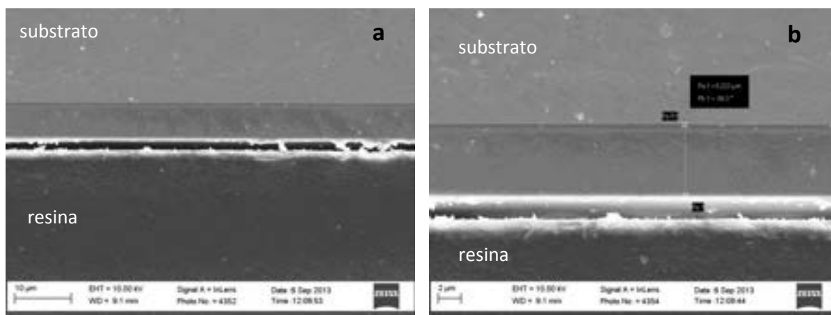
Figura 7. Micrografie SEM della sezione del rivestimento \text{Al}_2\text{O}_3 200 a) 2kx, b) 5kx, c) 10kx.
