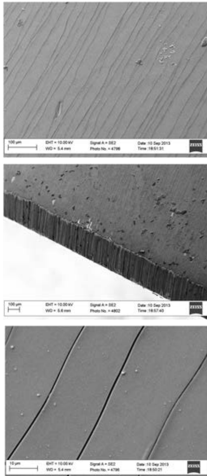
Figura 24. Micrografia SEM della superficie del campione spesso 5 µm e sottoposto ad elongazione pari al 2%.
