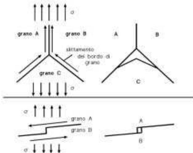
Fig. 10 – Meccanismi di danneggiamento intergranulare dovuti allo slittamento dei bordi di grano.
