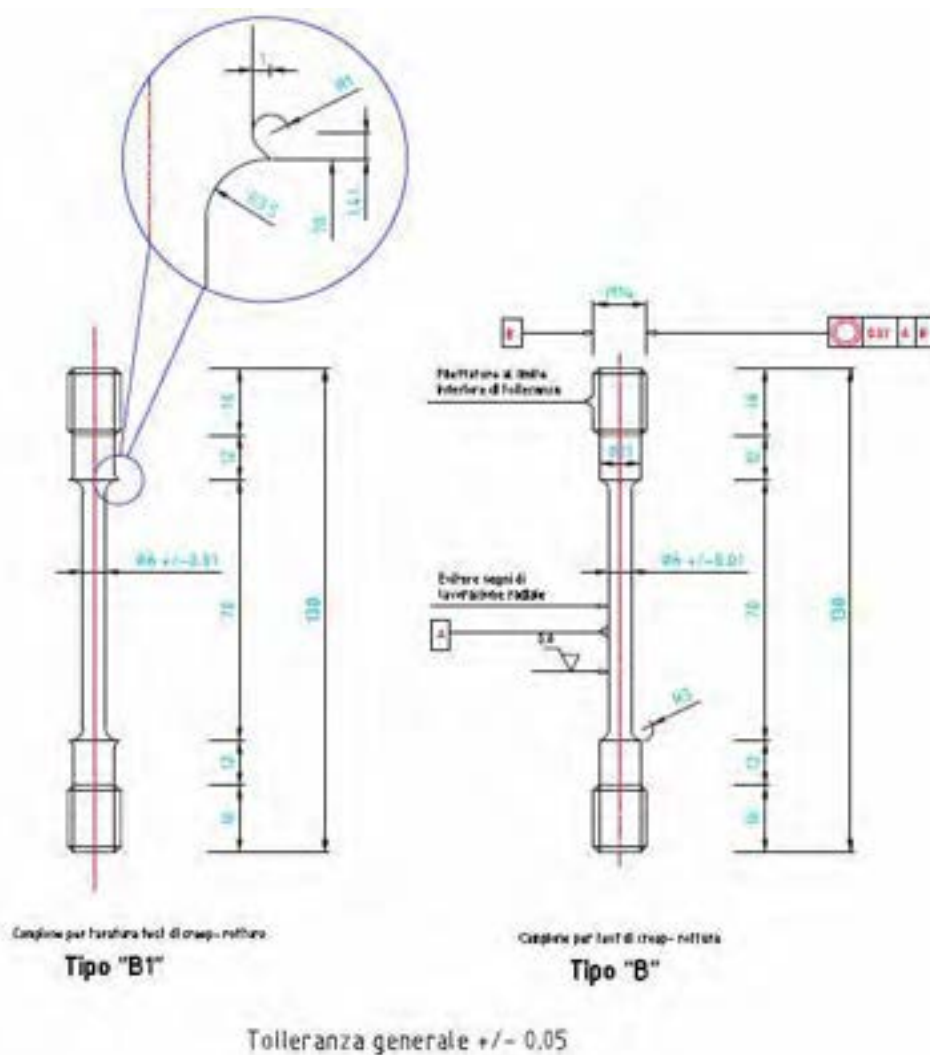
Dis.1: disegno dei campioni
