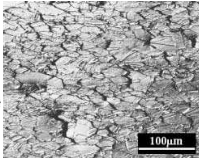
Fig. 11 – Esempio di cavità di tipo w in un acciaio AISI347 sottoposto a creep a 650°C.
