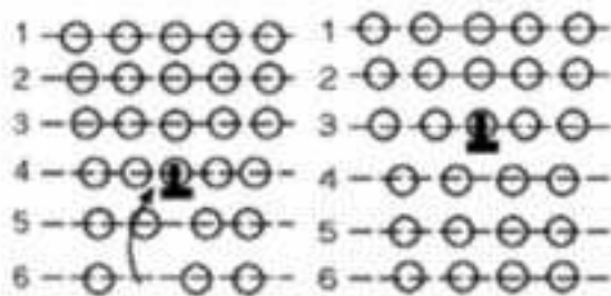
Fig. 1 – La vacanza sul piano 6 si sposta verso il bordo del emipiano della dislocazione a spigolo; il flusso di una serie di vacanze permette lo spostamento della dislocazione dal piano 4 al piano 3.
