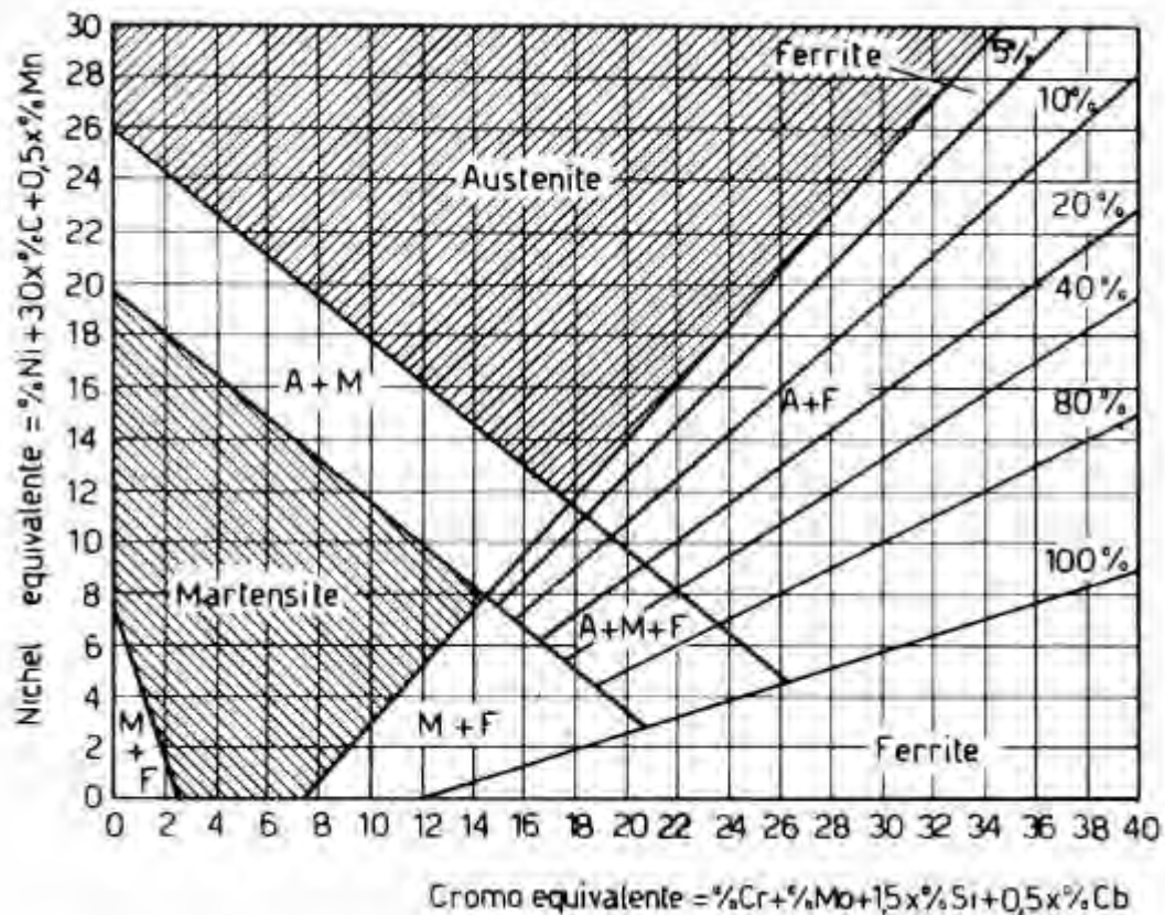
Fig. 7 – Diagramma Cr-Ni
