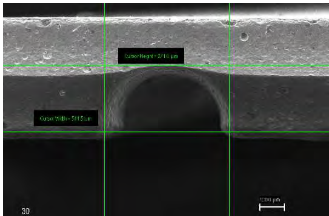
Fig. 48 – Misura di una gola a 30° di lamina trattata
