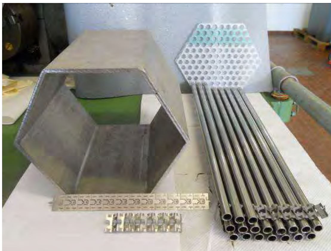
Fig. 65 – Componenti nella fase di montaggio del mock-up.
