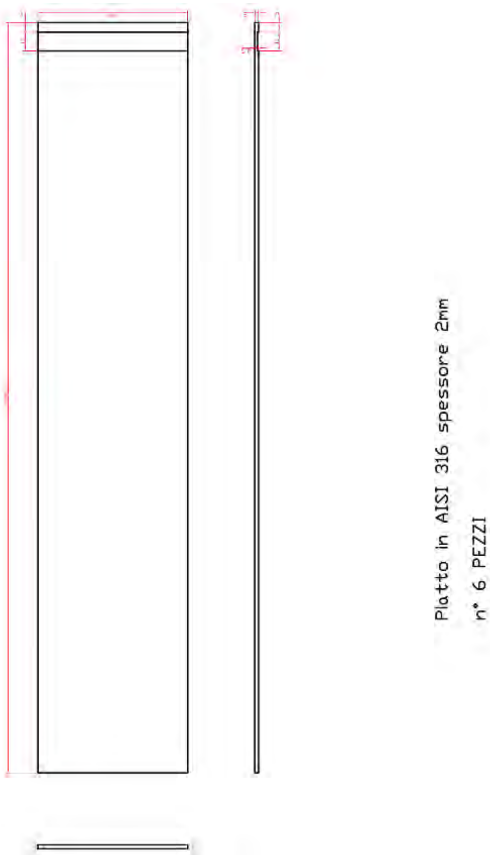
Fig. 9 – Lamine da inserire all'interno della scatola esagonale
