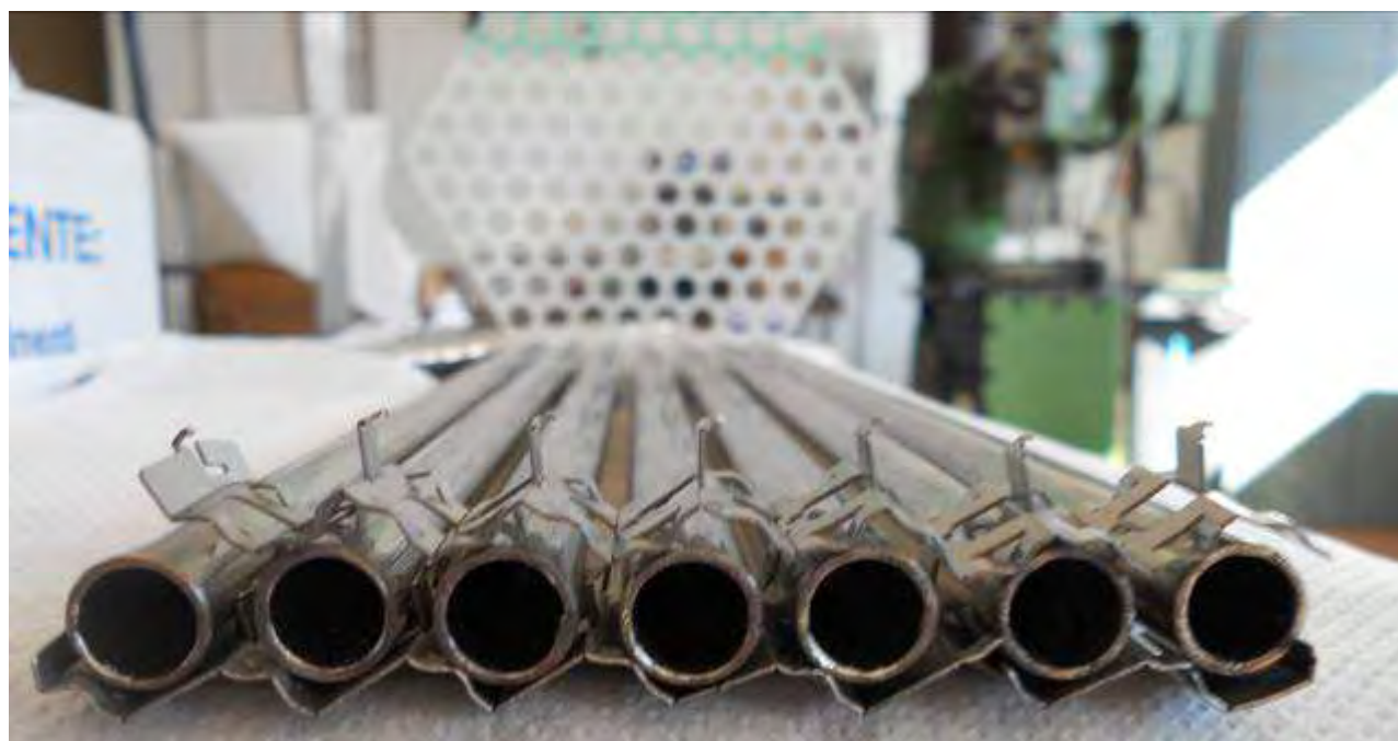
Fig. 59 – Fase di montaggio della seconda componente di griglia
