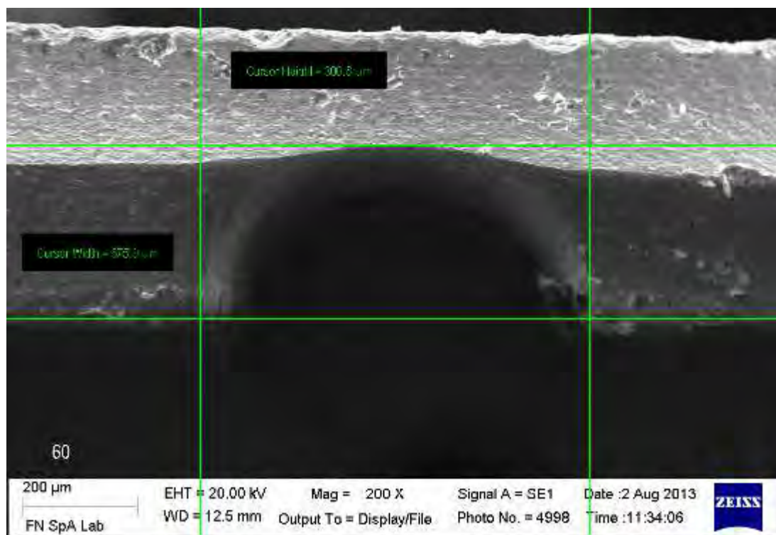
Fig. 50 – Misura di una gola a 60° su lamina incrudita al 50% tal quale
