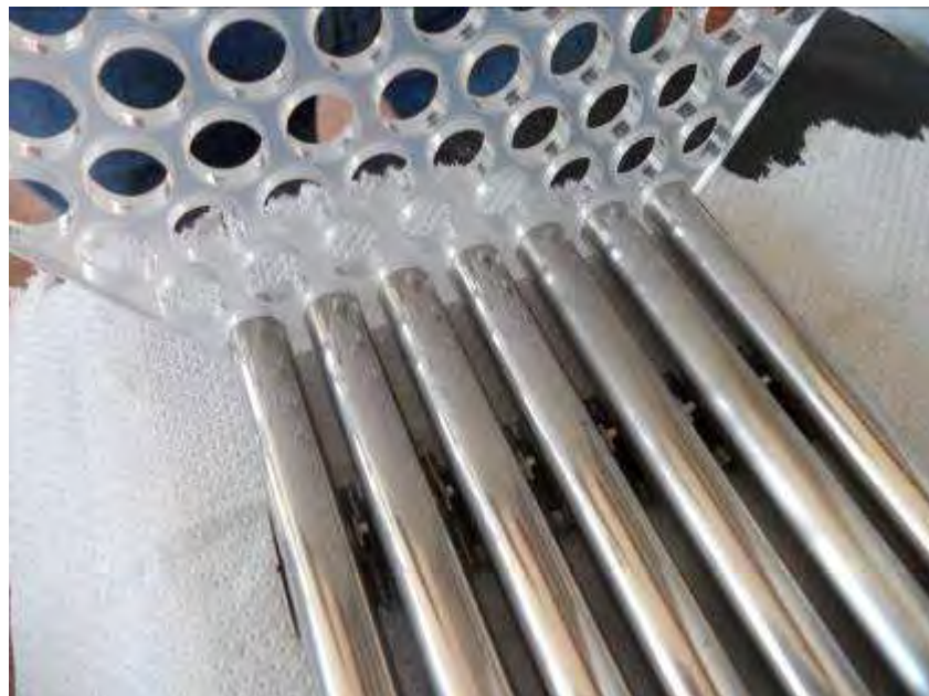
Fig. 56 – Particolare del piatto esagonale in plexiglass realizzato per mantenere in posizione distanziata le barrette all’atto del montaggio e visione degli uncini della prima componente di griglia che passano fra una barretta e l’altra in attesa della componente 2 della griglia cui agganciarsi.
