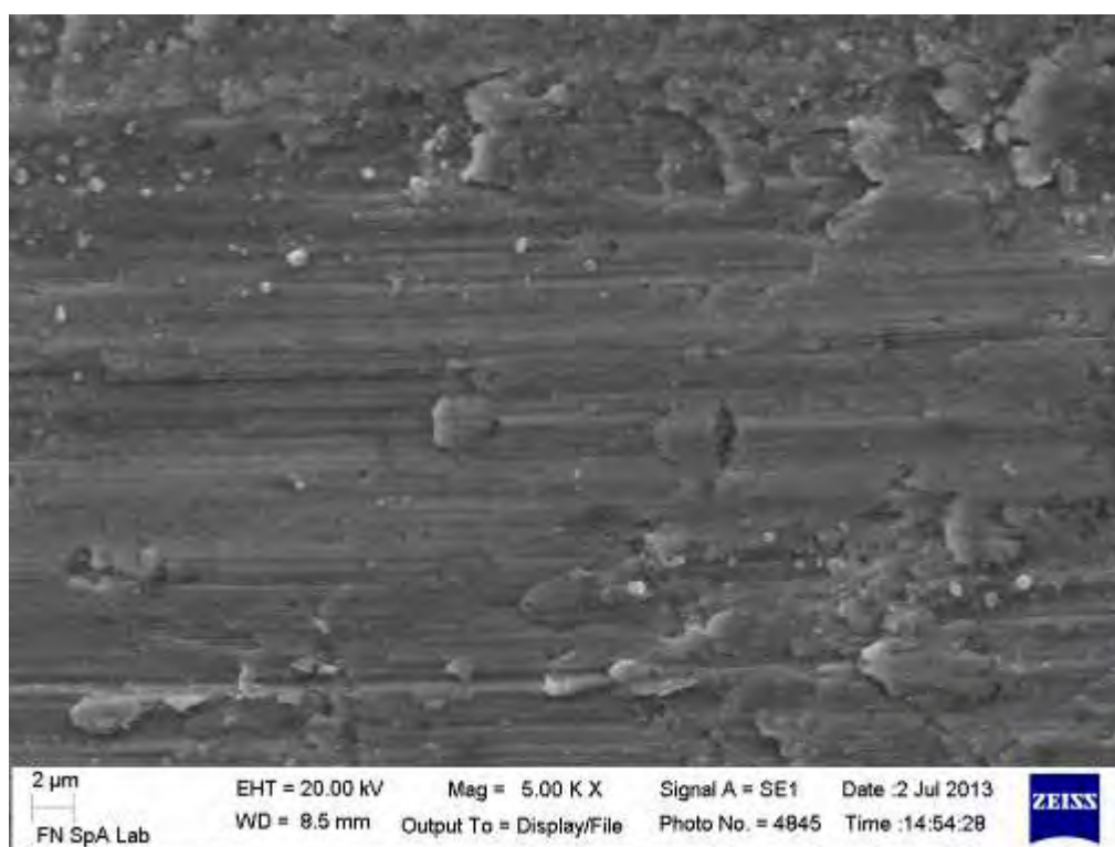
Fig. 35 – Immagine al SEM della lamina incrudita al 75% - superficie a 5000 X
