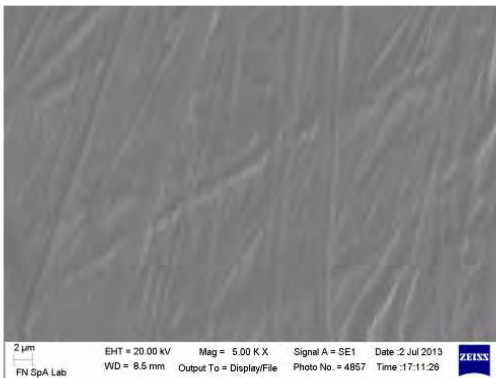
Fig. 37 – Immagine al SEM della lamina incrudita al 50% dopo solubilizzazione - 5000 X
