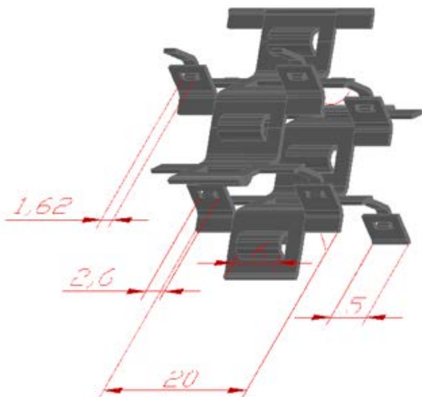
Fig. 4 – Vista in 3D della griglia proposta
