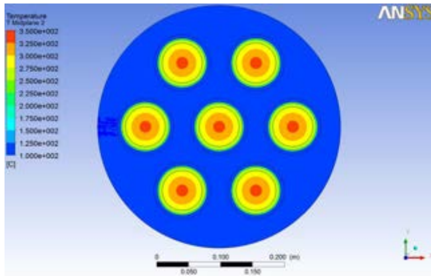
Figura 11 Distribuzione di temperatura sul piano medio.
