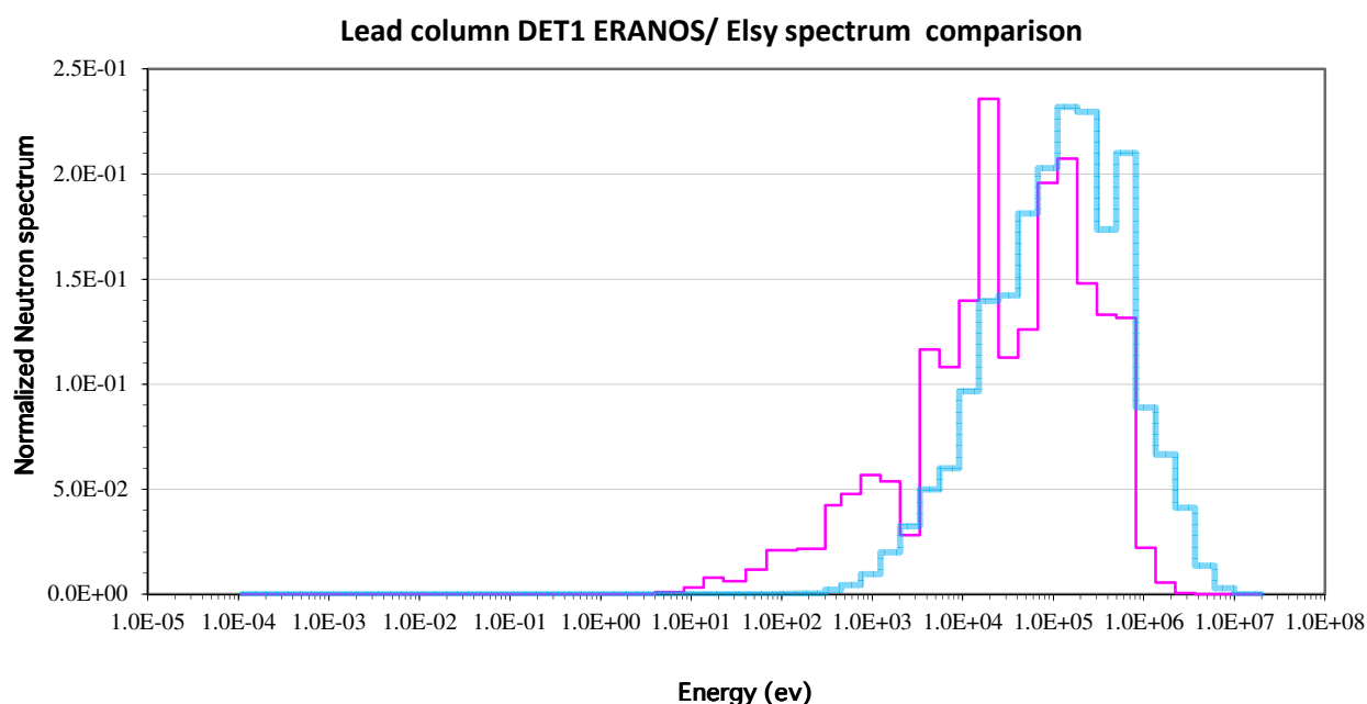
Fig. 10. Confronto degli spettri neutronici in TAPIRO (DET1) ed ELSY
