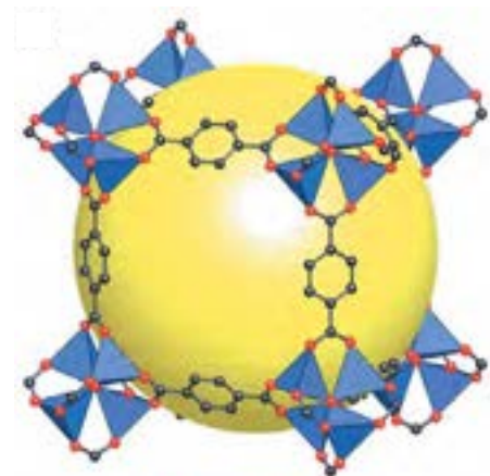
Figura 7. La struttura del MOF-5 presentata come tetraedri di ZnO_4 (poliedri di colore azzurro) uniti da legami con dicarbossilato di benzene (atomi di O in rosso e di C in nero), dando luogo ad un'ampia struttura cubica in 3D con pori interconnessi aventi un'apertura di 8 Å di larghezza e 12 Å di diametro (sfera gialla, rappresentante la sfera più grande che i pori possono occupare senza coincidere con l'ampiezza di van der Waals della struttura) [8]
