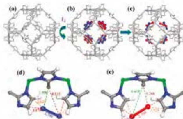
Figura 10. (a) Modello molecolare a sfere della struttura attivata prima dell'assorbimento di I_2 . (b) Due singoli siti di assorbimento delle molecole di I_2 all'interno del -cage, "Ia" (blu) e "Ib" (rosso). (c) Effettiva struttura molecolare (atomi di H tralasciati per chiarezza). (d, e) Distanze I_2 .....struttura a (d) sito Ia e (e) sito Ib. Gli atomi H dei gruppi -CH_3 sono stati tralasciati per chiarezza. Zn, verde; C, grigio; N, blu; H, bianco [12]
