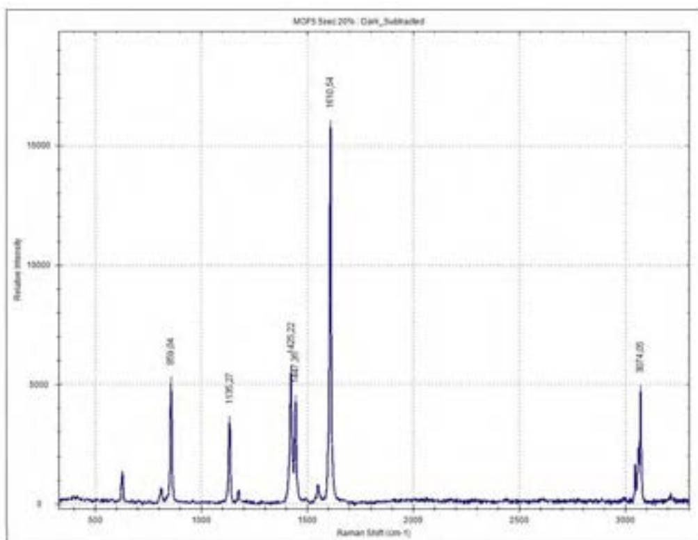
Figura 8. Spettro RAMAN di MOF-5
