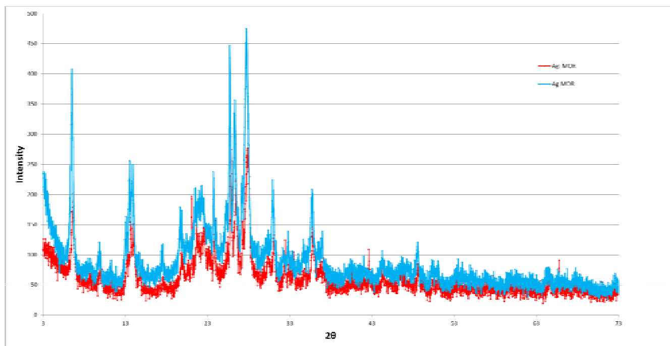
Figura 4b – Spettri XRD di Ag-MORDENITE
