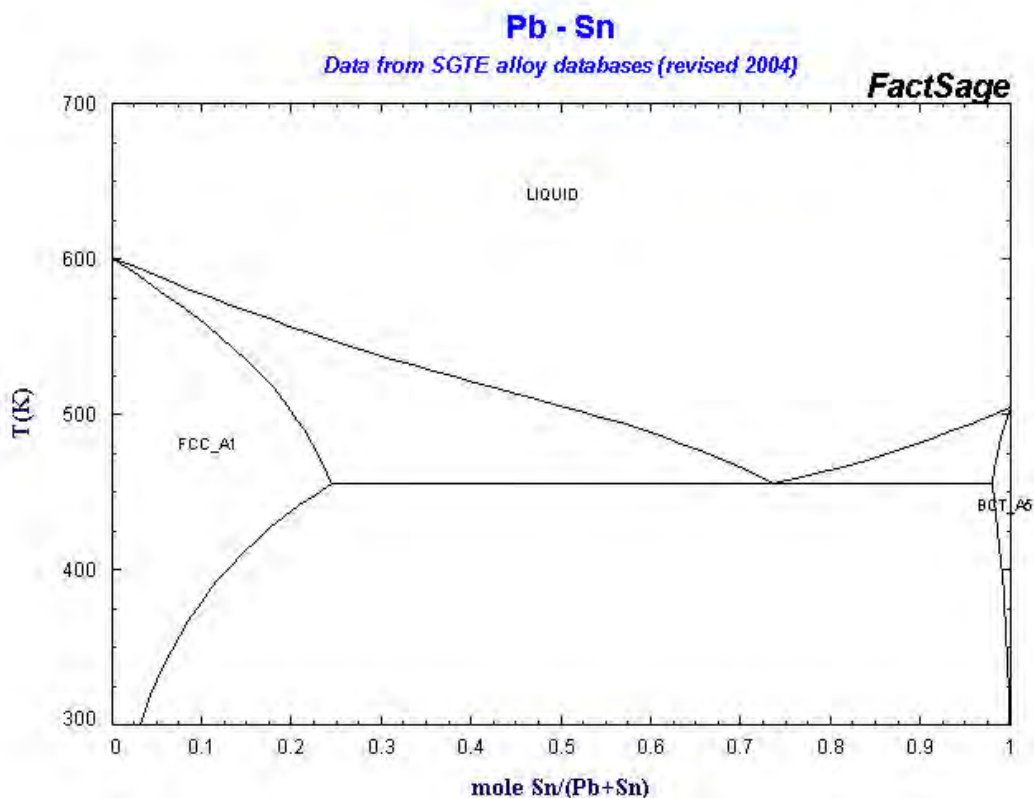
Figura 16. Diagramma di fase binario Pb-Sn [3]
