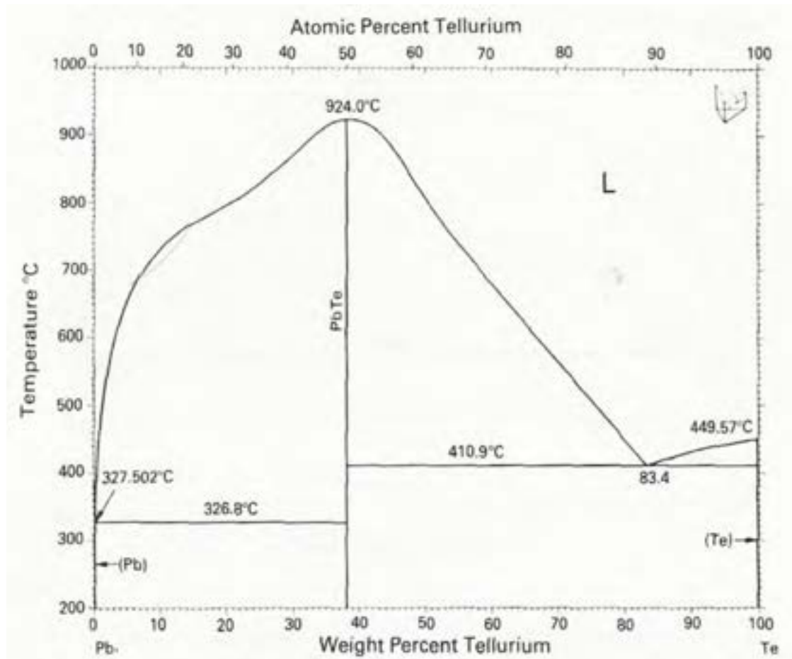
Figura 17. Diagramma di fase binario Pb-Te [4]
