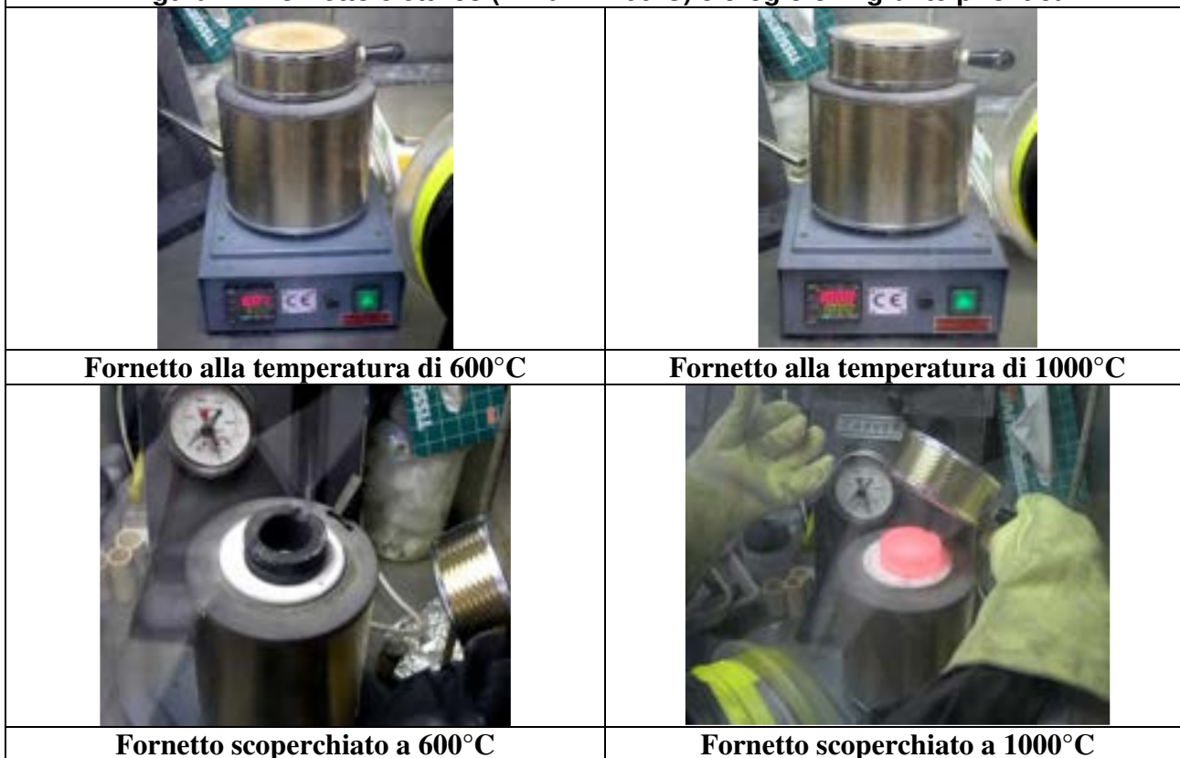
Figura 2 – Fornetto elettrico (T max: 1100°C) e crogiolo in grafite pirolitica
