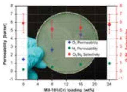
Figura 11. Struttura del MIL-101 (Molecola metallorganica di Chromo (III) Tereftalato (a sinistra). I microcristalli MIL-101 stabili all'acqua aderiscono bene al polisolfone (PSF) e danno luogo ad una membrana molto resistente in matrice mista MIL-101-PSF per la separazione O_2/N_2 con una selettività di 5–6 ed un aumento di permeabilità ad O_2 di un fattore da 4 ad oltre 6 per carichi di MIL-101 del 24% (a destra) [13]
