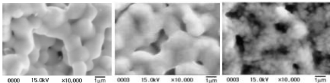
Figura 4. Fotografie al microscopio elettronico di fibre di yttria prima (a sinistra), dopo intrappolamento a 950°C (nel centro), e dopo intrappolamento a 1100°C (a destra) di ossidi di rutenio [4]
