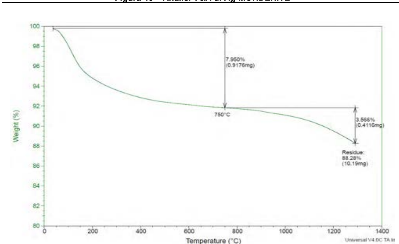
Figura 4c – Analisi TGA di Ag-MORDENITE
