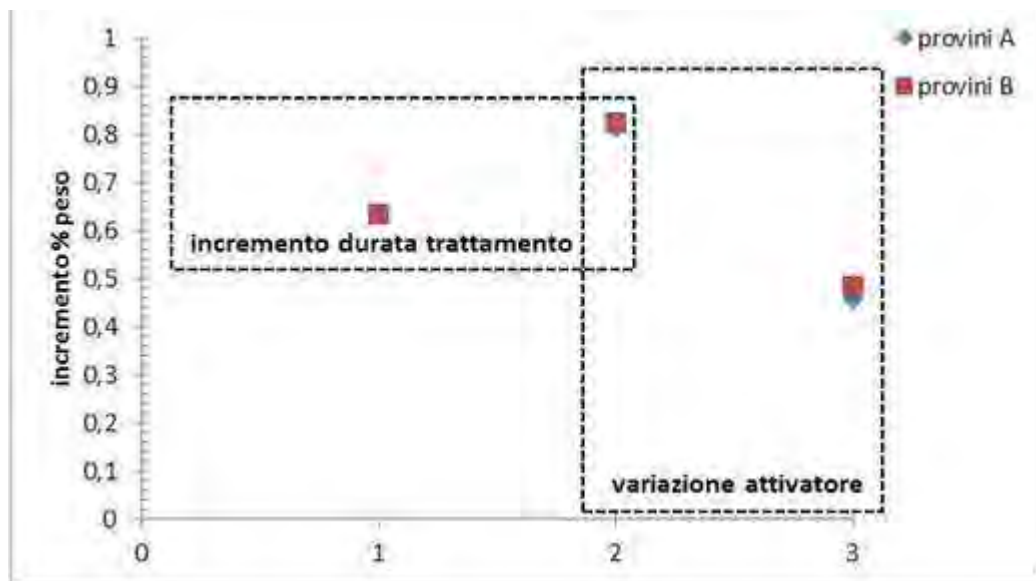
Figura 10 – Effetto della variazione dei parametri di processo sull'arricchimento in Al dei campioni
