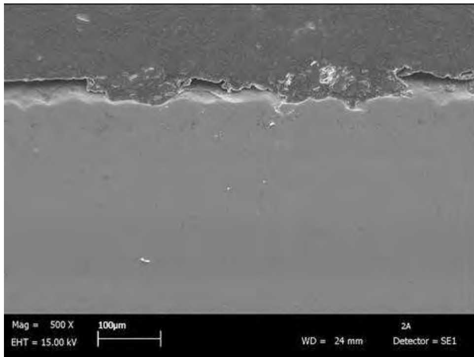
Figura 13 – Campione2A_500X (processo 1)
