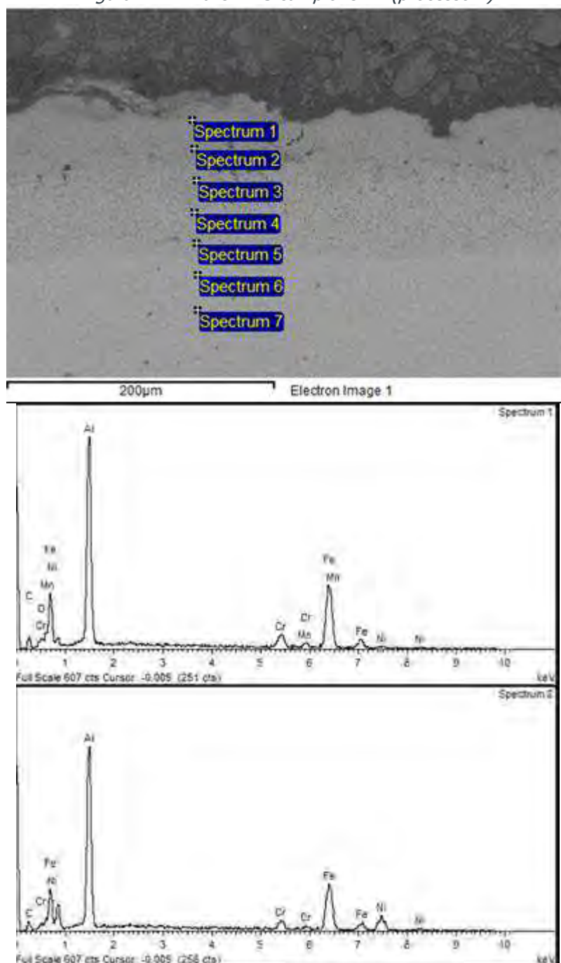
Figura 17 – Analisi EDS campione 2A (processo 1)
