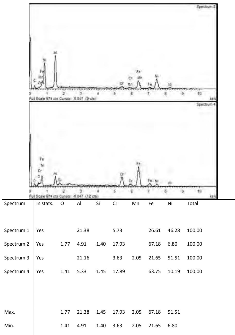
Figura 34 – Analisi EDS campione 5A (processo 2)
