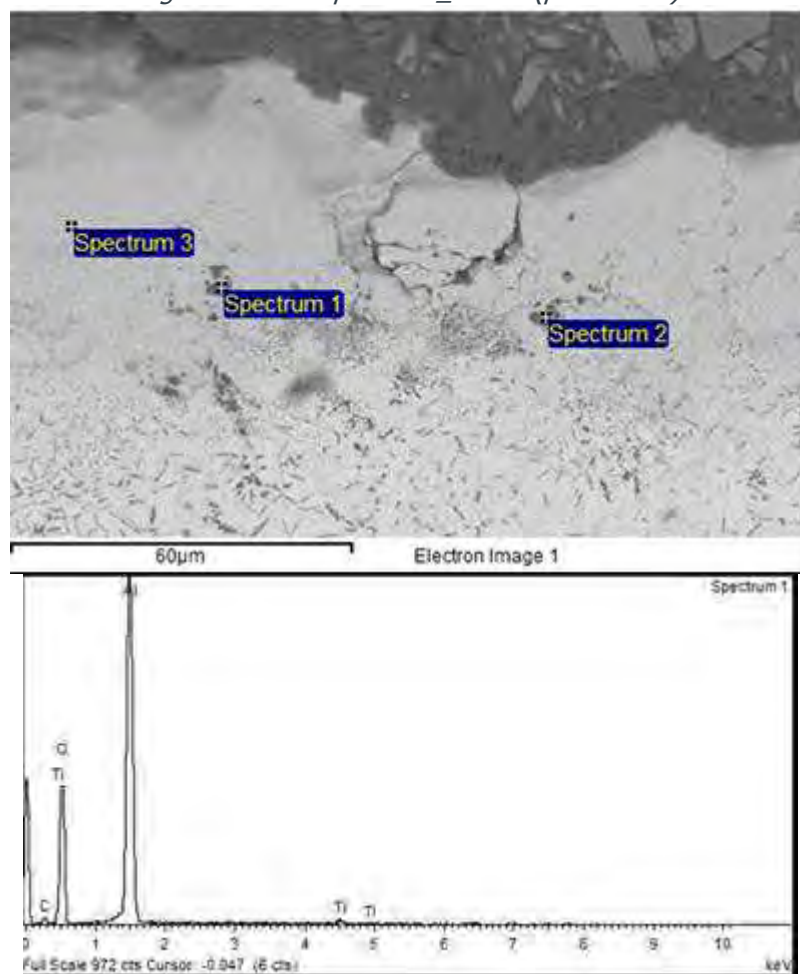
Figura 19 – Campione 2A_3000X (processo 1)
