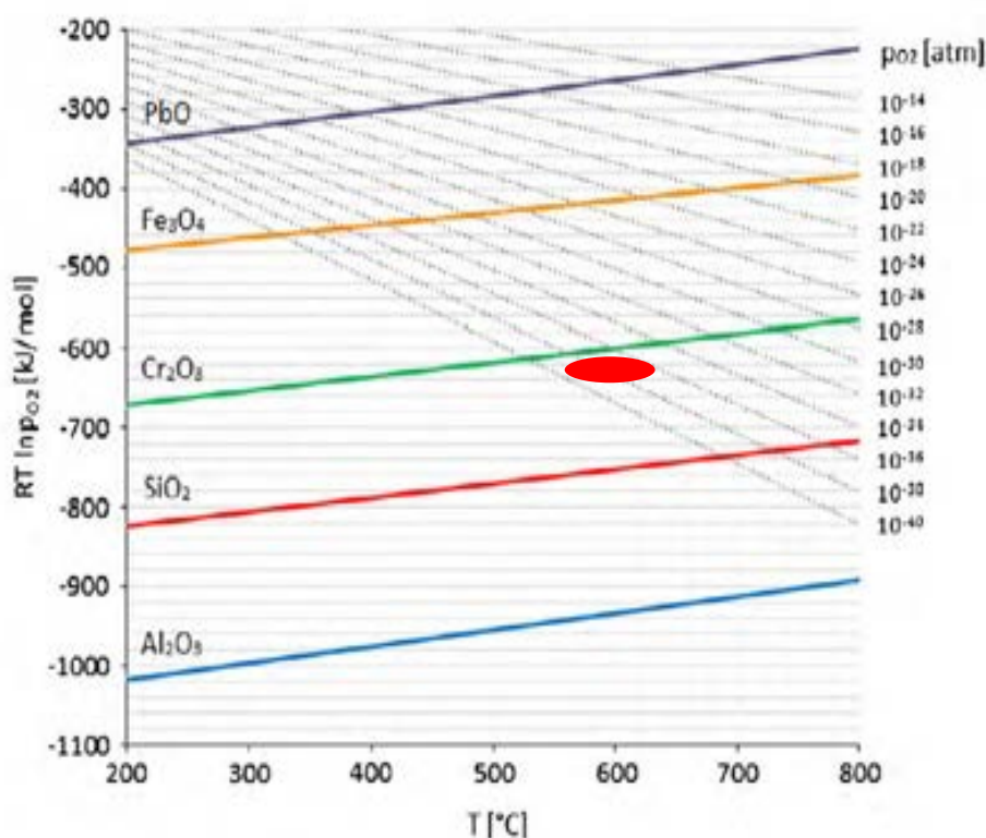
Figura 6. Condizioni in cui sono state svolte le prove di corrosione in Pb stagnante. Le condizioni sono ‘dissolutive’ perché il contenuto di ossigeno è insufficiente a formare ossidi di cromo e di ferro stabili, in grado di contrastare l’azione di dissoluzione da parte del Pb liquido.
