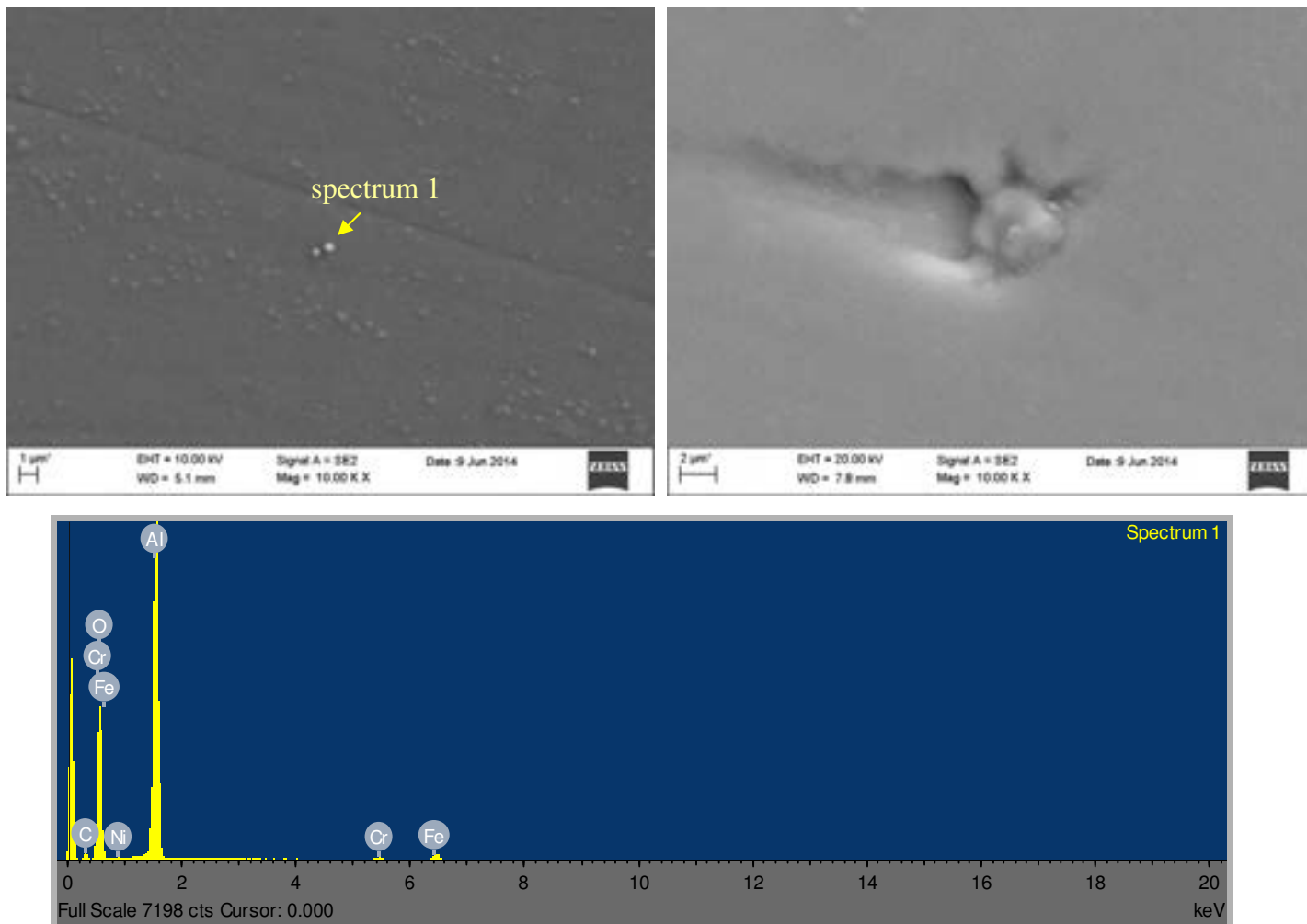
Fig. 8 Micrografie SEM e analisi EDS della superficie del rivestimento PLD di \text{Al}_2\text{O}_3 0 dpa. Ingrandimento 10 kx.
