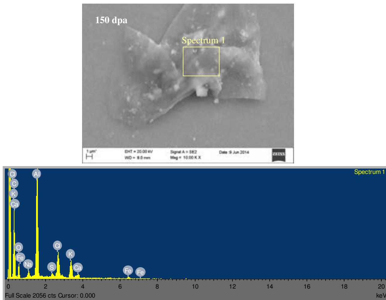
Fig. 10 Micrografie SEM e analisi EDS della superficie del rivestimento PLD di \text{Al}_2\text{O}_3 150 dpa. Ingrandimento 10 kx.
