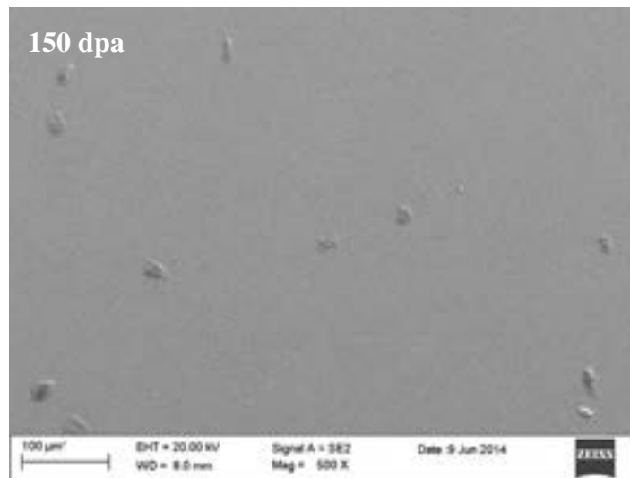
Fig. 5 Micrografie SEM della superficie dei rivestimenti PLD di \text{Al}_2\text{O}_3 (0, 50 e 150 dpa). Ingrandimento 500 x.
