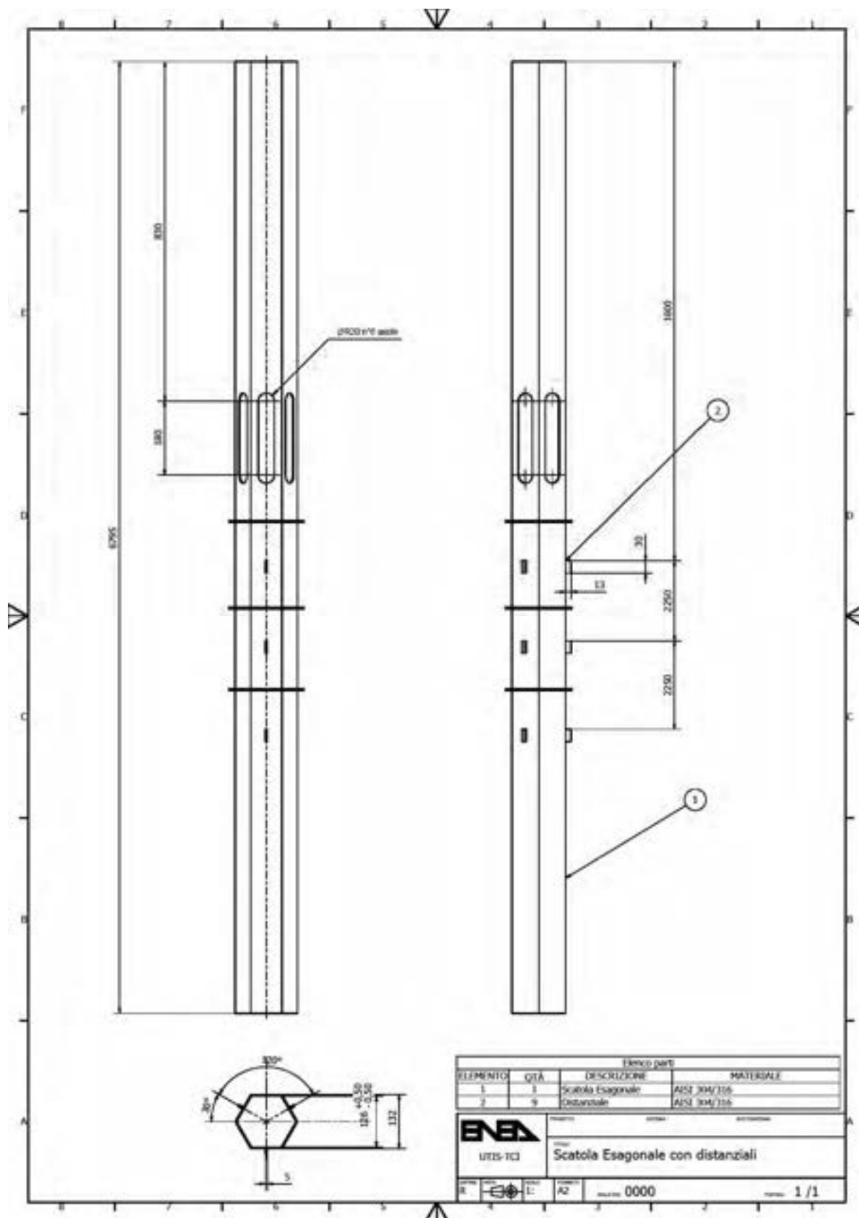
Fig. A. 4 – HERO-CIRCE SGBT hexagonal inner wrap.
