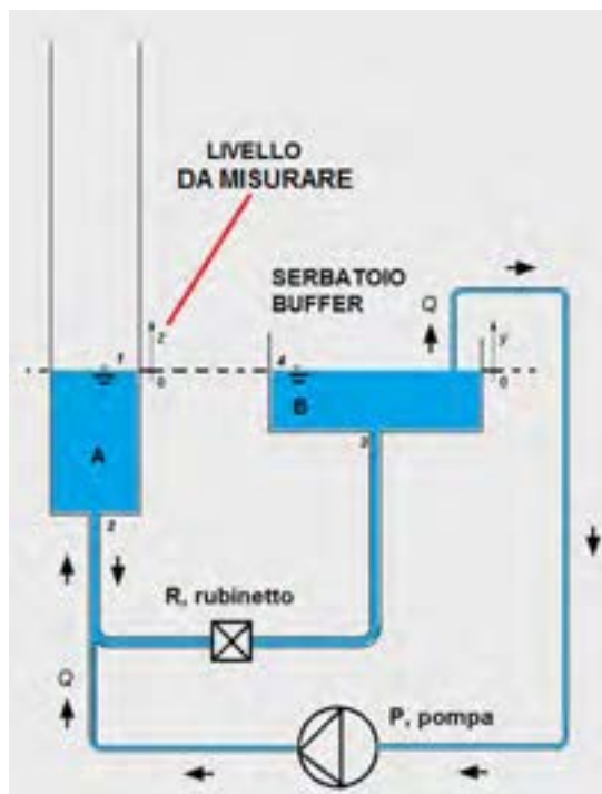
Figura 18: schema del prototipo a PTA in misura dinamica
