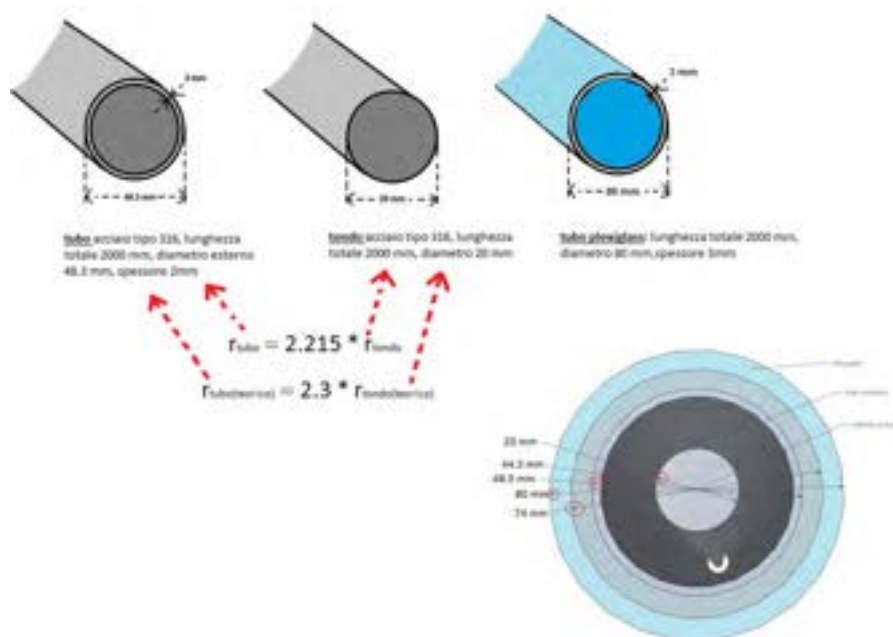
Figura 22: parametri geometrici della sezione a PTA
