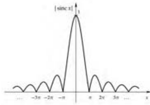
Figura 7: modulo di sinc(x)
