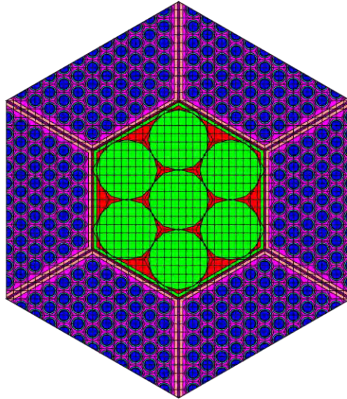
Fig. 69 – SCALE Dummy SA model.
