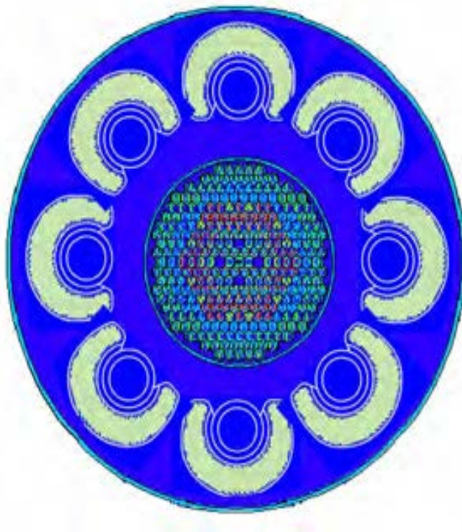
Figura 1 - Vista in pianta del nocciolo del reattore ALFRED e dei generatori di vapore.
