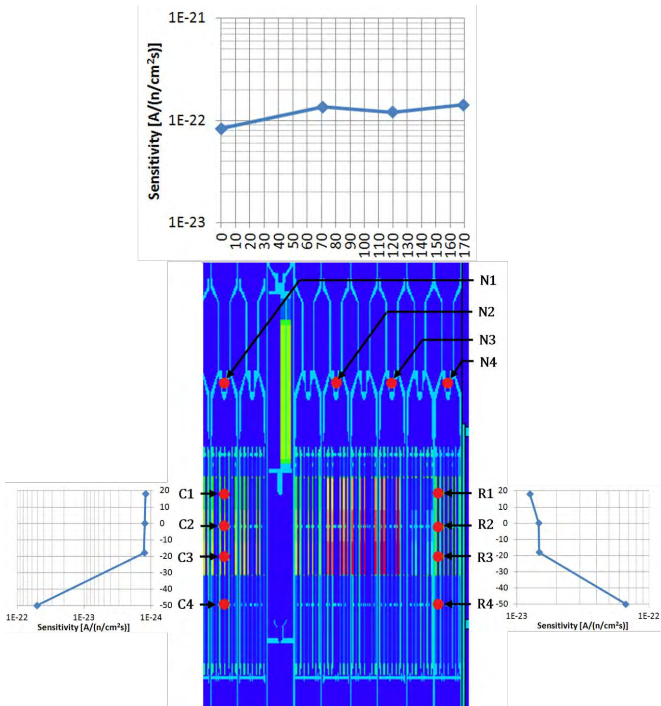
Figura 14 - Sensibilità del SPND THERMOCOAX Co-type (current mode) in funzione della posizione d'installazione in ALFRED.
