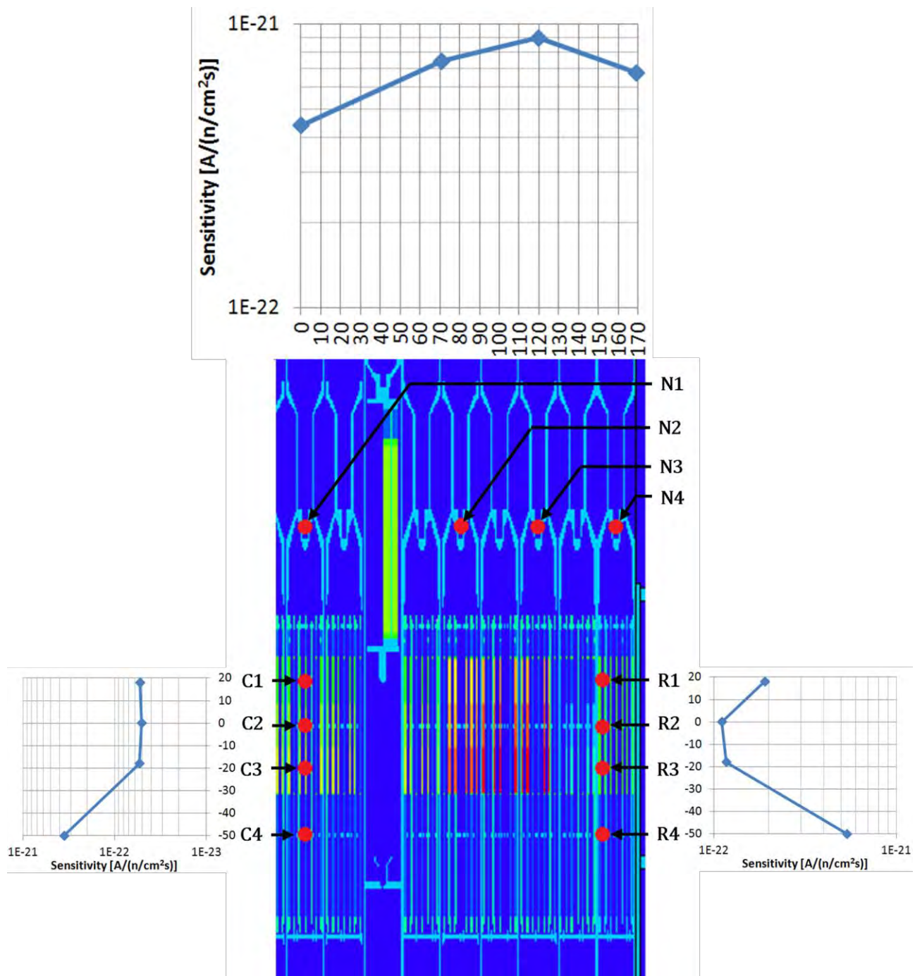
Figura 15 - Sensibilità del SPND THERMOCOAX Pt-type (current mode) in funzione della posizione d'installazione in ALFRED
