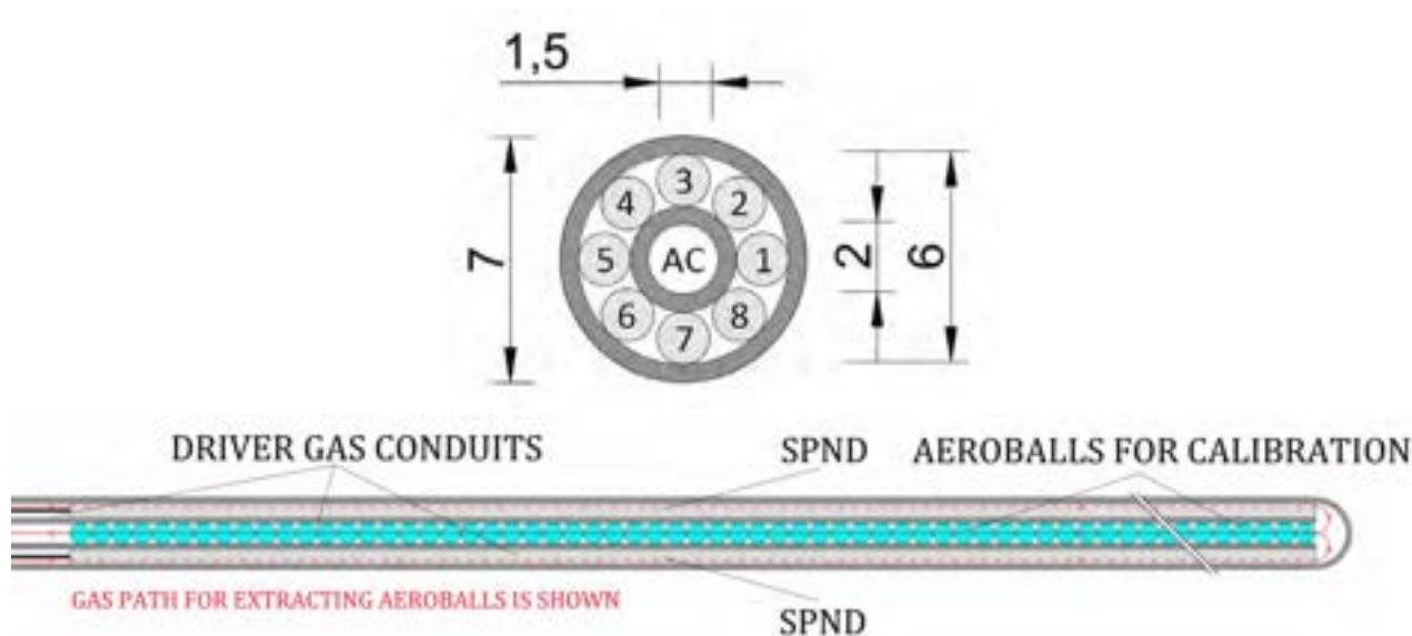
Figura 27 - Struttura della sonda in-core proposta, costituita da 8 SPND disposti radialmente attorno ad un canale centrale ricavato per la taratura della sonda stessa mediante attivazione neutronica di opportuno materiale. Tutte le dimensioni sono in [mm].
