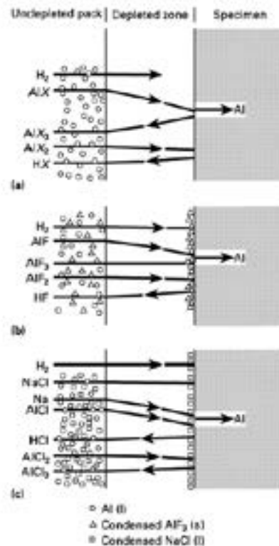
Figura II.1.1 – Diagramma schematico dei flussi delle principali specie gassose diffondenti nei pack di alluminizzazione attivati con (a) \text{NH}_4\text{X} ( \text{X}=\text{Cl}, \text{Br}, \text{I} ), (b) \text{NH}_4\text{F} , (c) \text{NaCl} (figura tratta da rif. 2)
