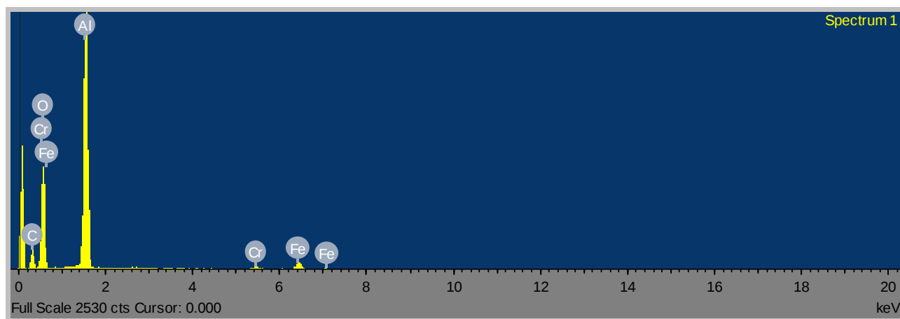
Fig. 3 Micrografie SEM e analisi EDS della superficie del campione 5\ \mu\text{m}\ \text{Al}_2\text{O}_3/500\ \text{nm}\ \text{FeCrAlY}/316 dopo irraggiamento a 16 dpa a RT
