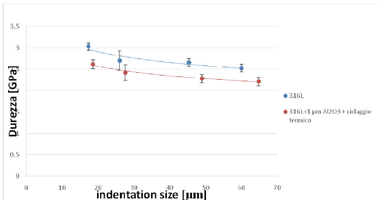
Fig. 20 Andamento microdurezza Vickers in funzione della dimensione dell'impronta del campione 134 (1 \mu\text{m} Al 2 O 3 /316L ciclatο termicamente in Ar) e dell'acciaio 316L
