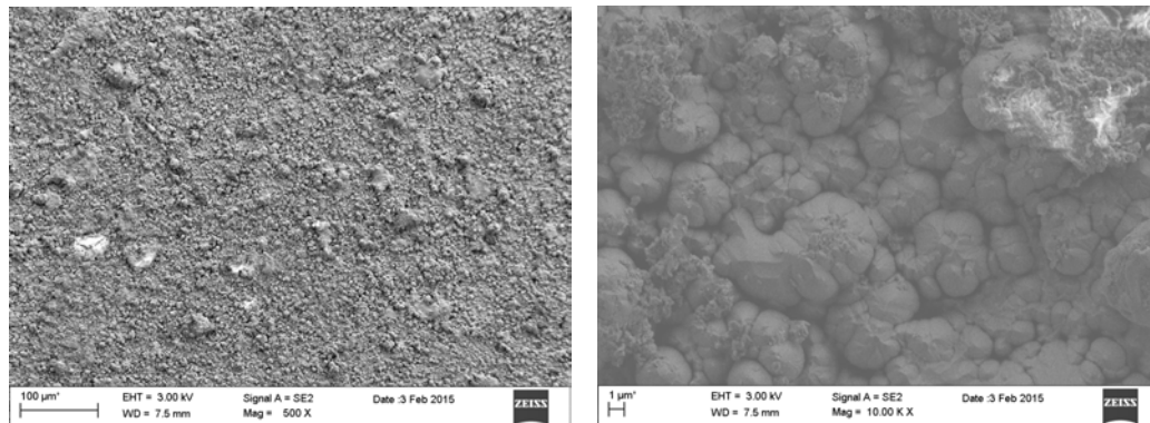
Fig. 9 Micrografie SEM della superficie del campione \text{Al}_2\text{O}_3 (RF sputtering)/FeCrAl (arc-PVD)/ 316 as-deposited
