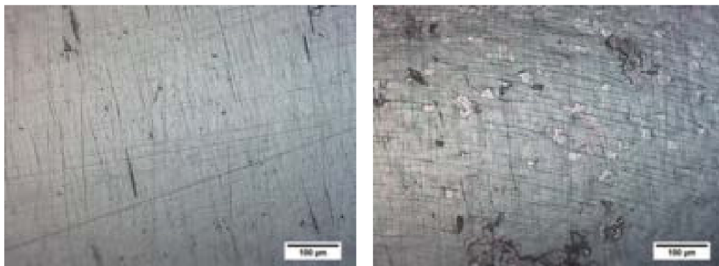
Fig. 25 Microscopia ottica della superficie inferiore del campione 134 ( 1\text{ }\mu\text{m Al}_2\text{O}_3/316\text{L} ciclato termicamente in Ar) (sinistra) e superficie laterale (destra)
