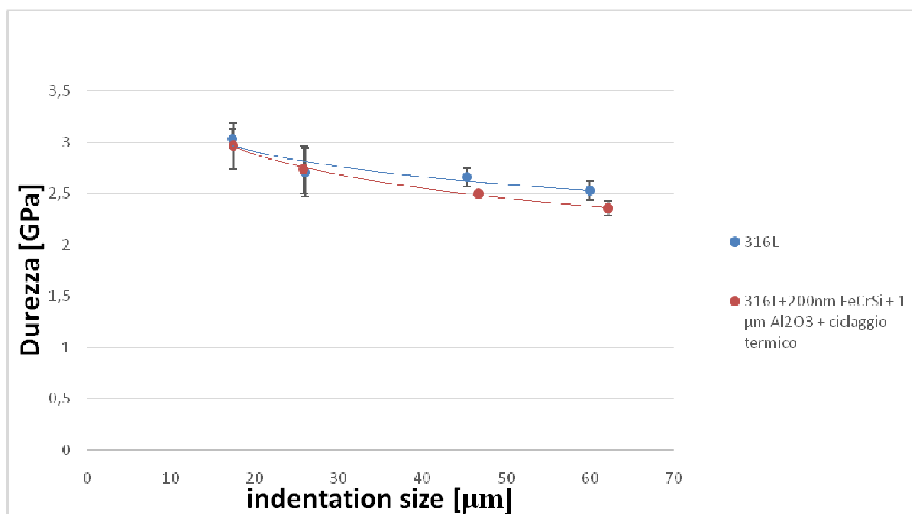
Fig. 21 Andamento microdurezza Vickers in funzione della dimensione dell'impronta del campione 136 ( 1 \mu\text{m Al}_2\text{O}_3/200 \text{ nm FeCrSi}/316\text{L} ciclato termicamente in Ar) e dell'acciaio 316L
