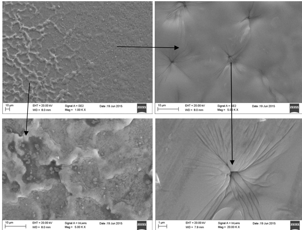
Fig. 4 Micrografie SEM della superficie del campione 5\text{ }\mu\text{m Al}_2\text{O}_3 / 500\text{ nm FeCrAlY/316} dopo irraggiamento a 16 dpa a 550^\circ\text{C}
