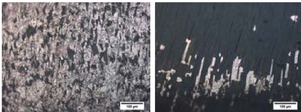
Fig. 27 Microscopia ottica della superficie del campione 137 ( 1\text{ }\mu\text{m Al}_2\text{O}_3/200\text{ nm FeCrSi}/1515\text{Ti} ciclato termicamente in Ar) zona sottoposta a freccia massima (sinistra) e zona laterale (destra)
