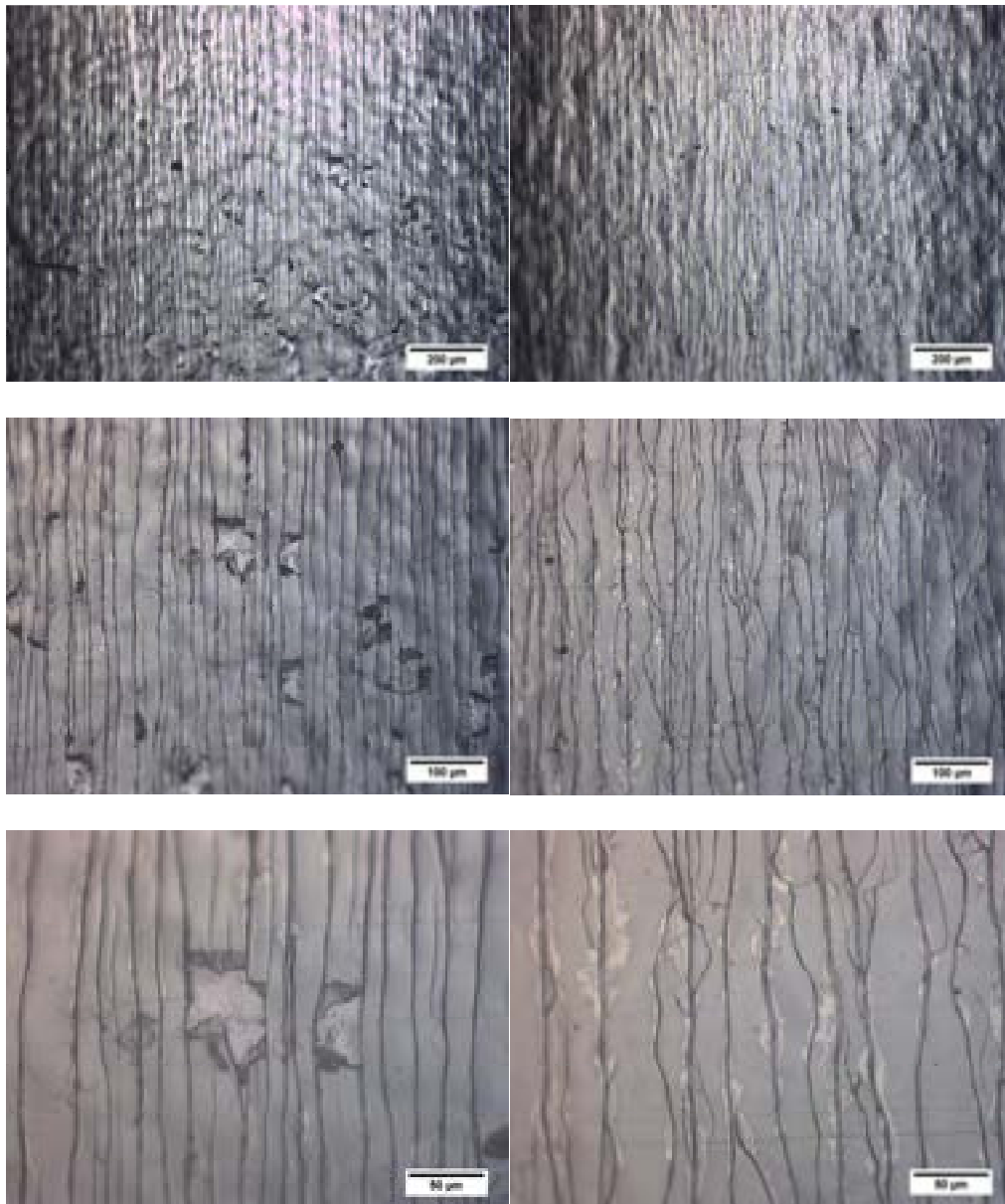
Fig. 17 Microscopia ottica della superficie del campione 10 \mu\text{m} \text{Al}_2\text{O}_3 /316L sottoposta a freccia massima nella prova di flessione
