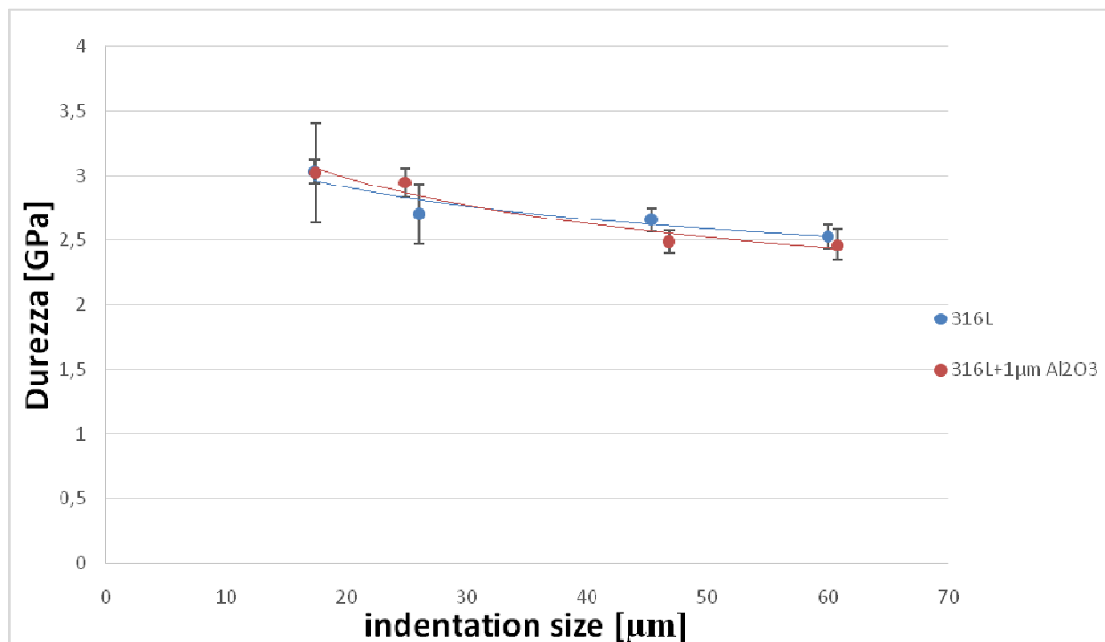
Fig. 19 Andamento microdurezza Vickers in funzione della dimensione dell'impronta del campione 163 (1 \mu\text{m} Al 2 O 3 /316L) e dell'acciaio 316L
