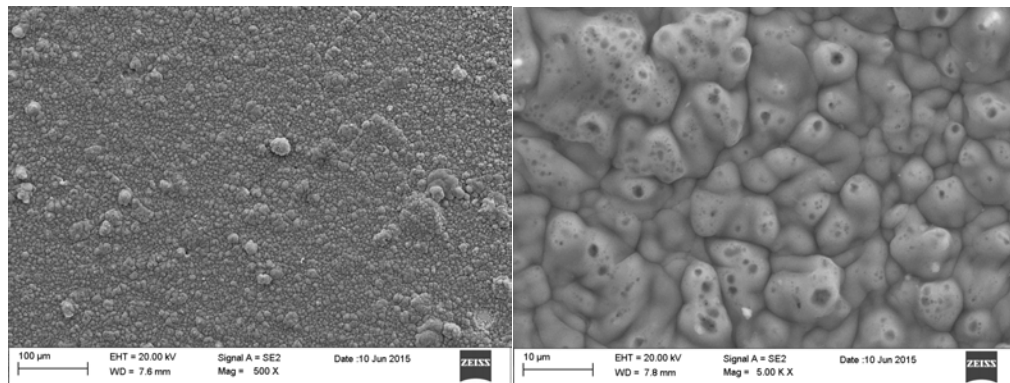
Fig. 10 Micrografie SEM della superficie del campione \text{Al}_2\text{O}_3 (RF sputtering)/FeCrAl (arc-PVD)/ 316 dopo irraggiamento a 16 dpa a RT
