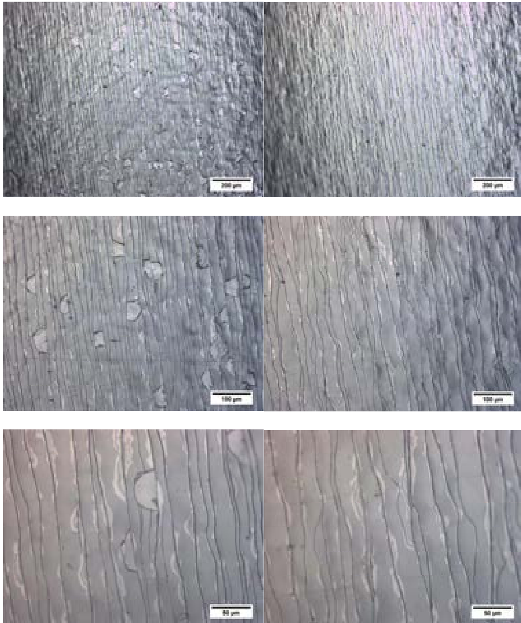
Fig. 16 Microscopia ottica della superficie del campione 5μm Al 2 O 3 /316L sottoposta a freccia massima nella prova di flessione
