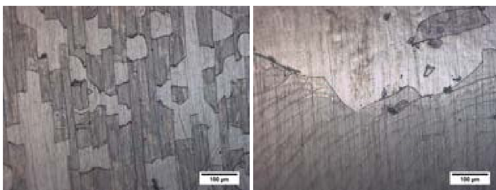
Fig. 28 Microscopia ottica della superficie del campione 162 ( 5\text{ }\mu\text{m Al}_2\text{O}_3/316\text{L} ) zona sottoposta a freccia massima (sinistra) e zona laterale (destra)
