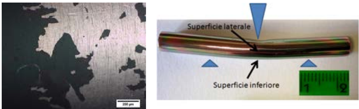
Fig. 26 Microscopia ottica della superficie del campione 136 ( 1\text{ }\mu\text{m Al}_2\text{O}_3/200\text{ nm FeCrSi/ 316L} ciclato termicamente in Ar) relativa alla zona sottoposta a freccia massima
