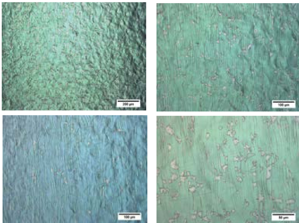
Fig. 15 Microscopia ottica della superficie del campione 1 \mu m Al 2 O 3 /316L sottoposta a freccia massima nella prova di flessione
