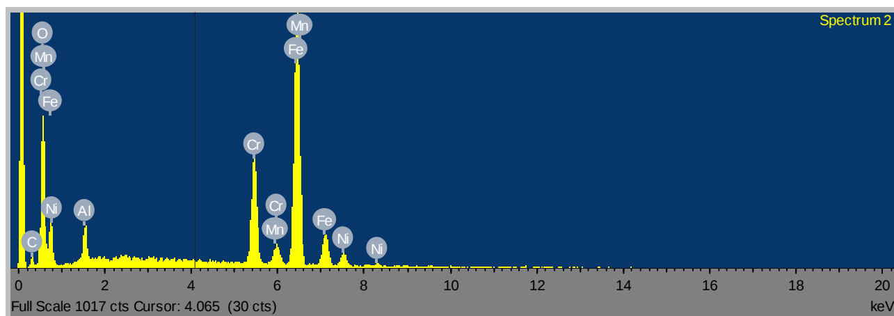
Fig. 2 Micrografia SEM e analisi EDS della superficie del campione 5\ \mu\text{m}\ \text{Al}_2\text{O}_3/500\ \text{nm}\ \text{FeCrAlY}/316 dopo irraggiamento a 16 dpa a RT
