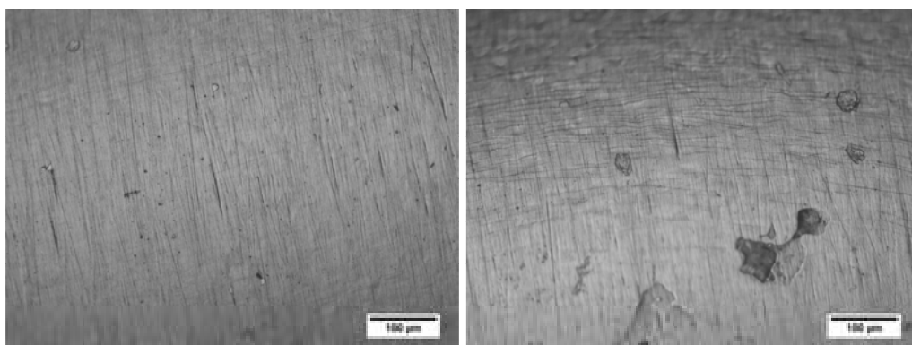
Fig. 29 Microscopia ottica della superficie del campione 163 ( 1\text{ }\mu\text{m Al}_2\text{O}_3/316\text{L} ) zona sottoposta a freccia massima (sinistra) e zona laterale (destra)
