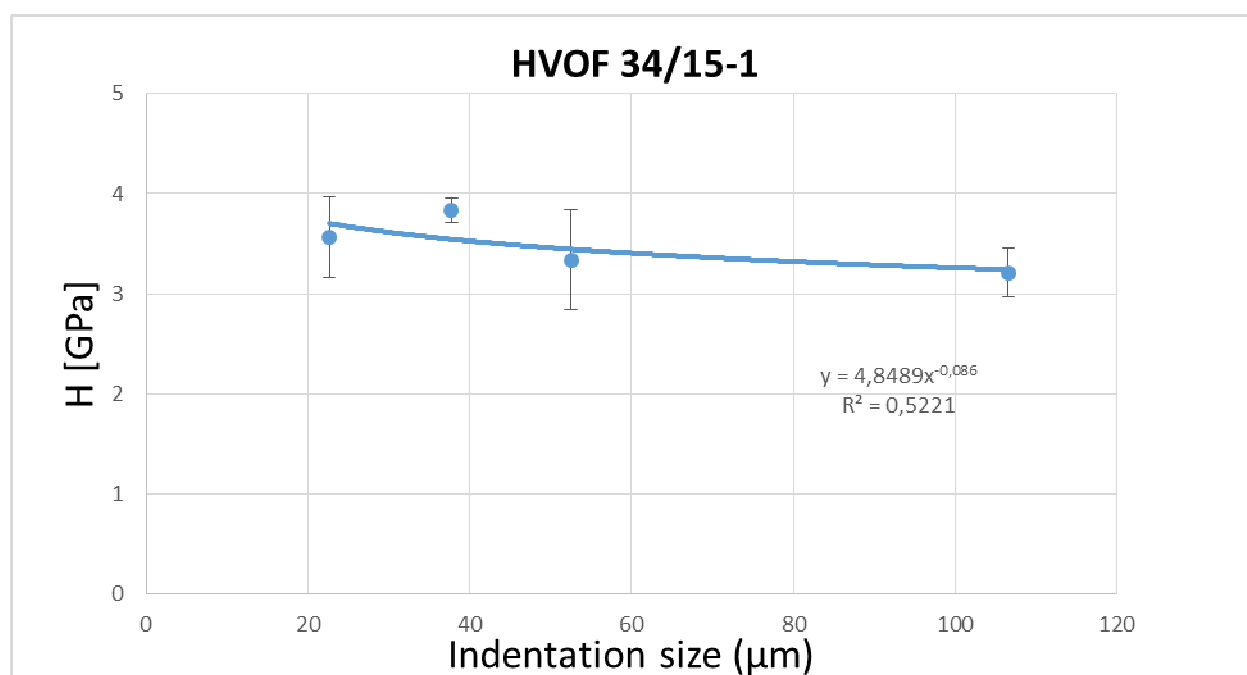
Fig. 40 Valori di Microdurezza Vickers del campione 34/15-1
