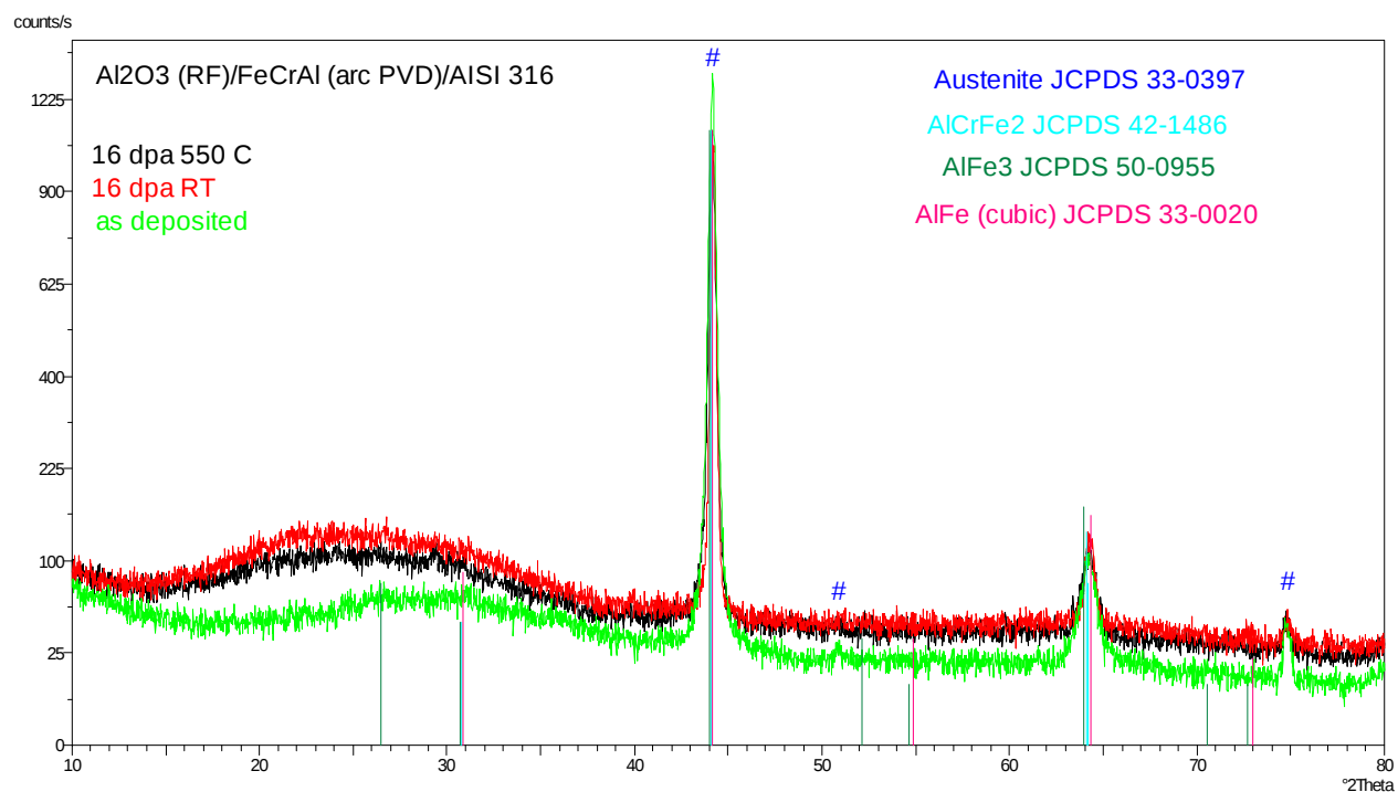
Fig. 12 Pattern di diffrazione di raggi X dei campioni (\text{RF sputtering})/\text{FeCrAl} (\text{arc-PVD})/ 316 as-deposited e sottoposti a irraggiamento
