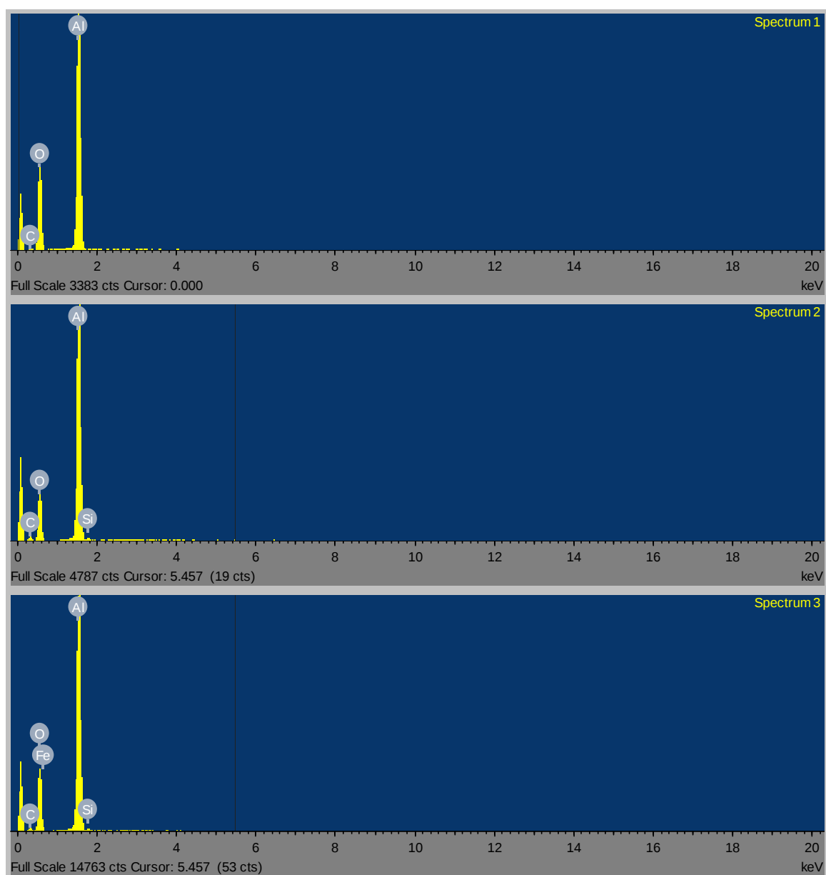
Fig. 5 Micrografie SEM e analisi EDS della superficie del campione 5 \mu\text{m} \text{Al}_2\text{O}_3 / 500 nm FeCrAlY/ 316 dopo irraggiamento a 16 dpa a 550°C
