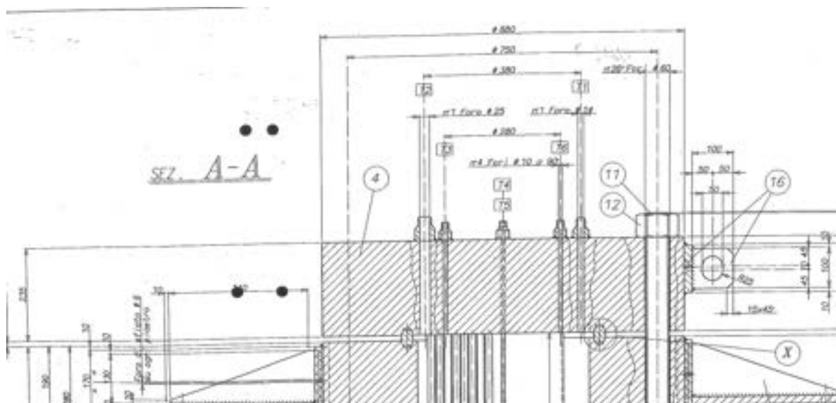
Fig. 5.13 – Disegni “originali” della flangia superiore del serbatoio di prova S1.
