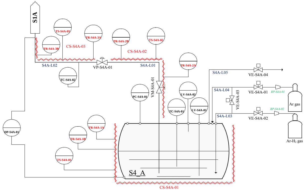
Fig. 5.1 – P&I sistema “fill and drain” e tanca stoccaggio S4_A.
