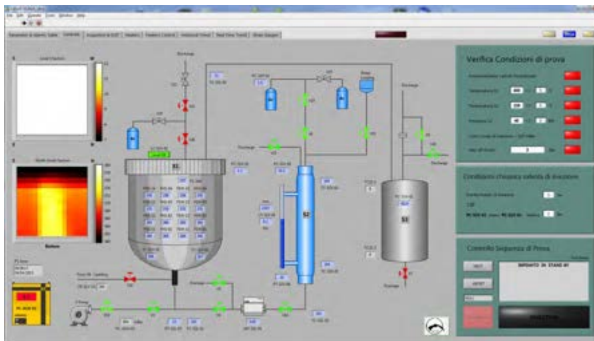
Fig. 4.5 – LIFUS5/Mod2. Configurazione THINS: sinottico di impianto (Test A1.2 – fase di caricamento LBE).
