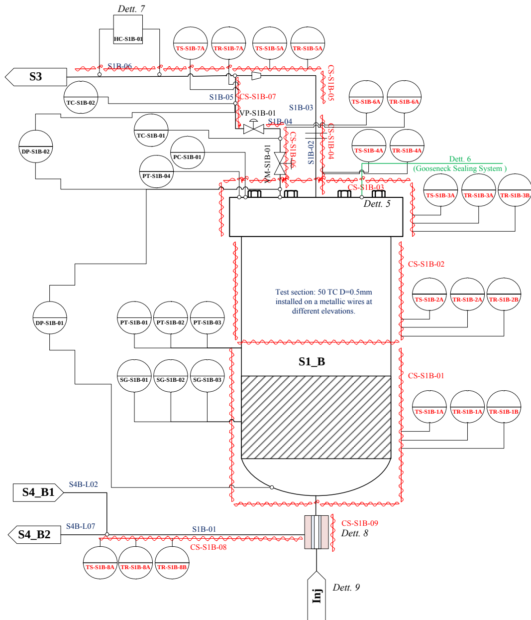
Fig. 5.4 – P&I preliminare sistema S1_B dell'impianto LIFUS5/Mod3.
