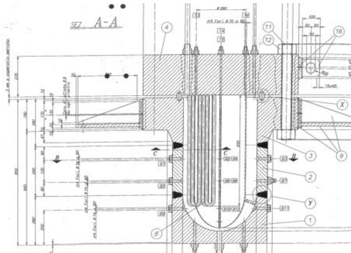
Fig. 5.12 – Disegni “originali” del serbatoio di prova S1 (parte 2 di 2).
