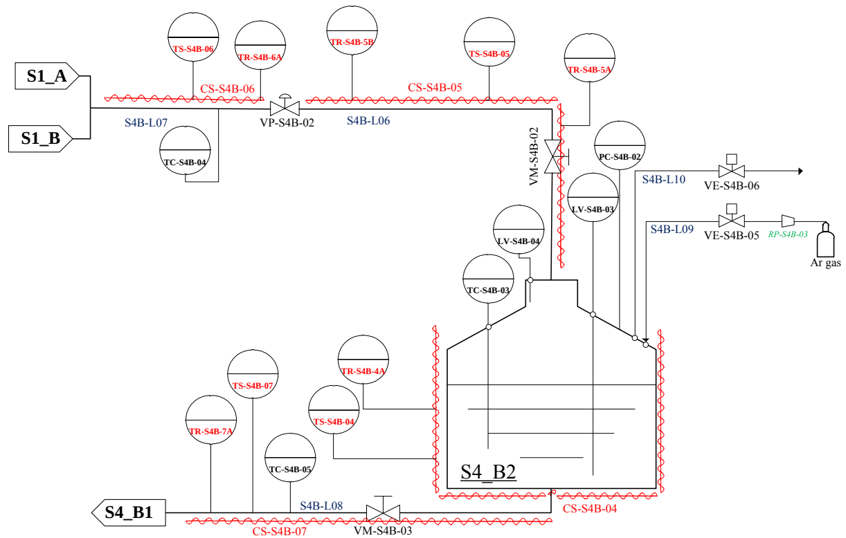
Fig. 5.3 – P&I sistema “fill and drain” e tanca stoccaggio S4_B2.
