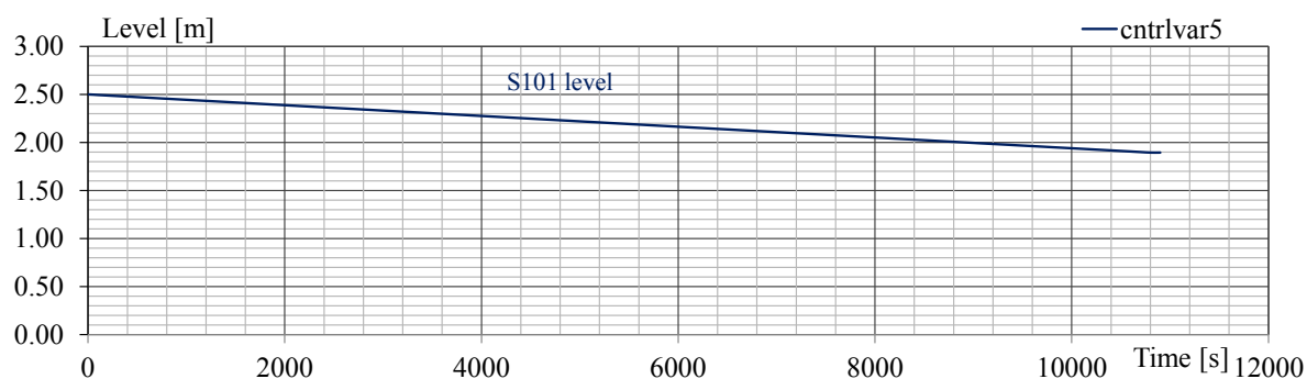
Fig. A. 12 – Level in S101 (water tank)
