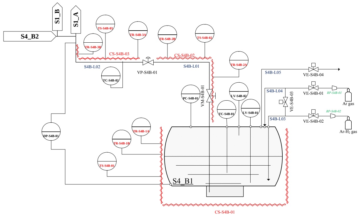
Fig. 5.2 – P&I sistema “fill and drain” e tanca stoccaggio S4_B1
