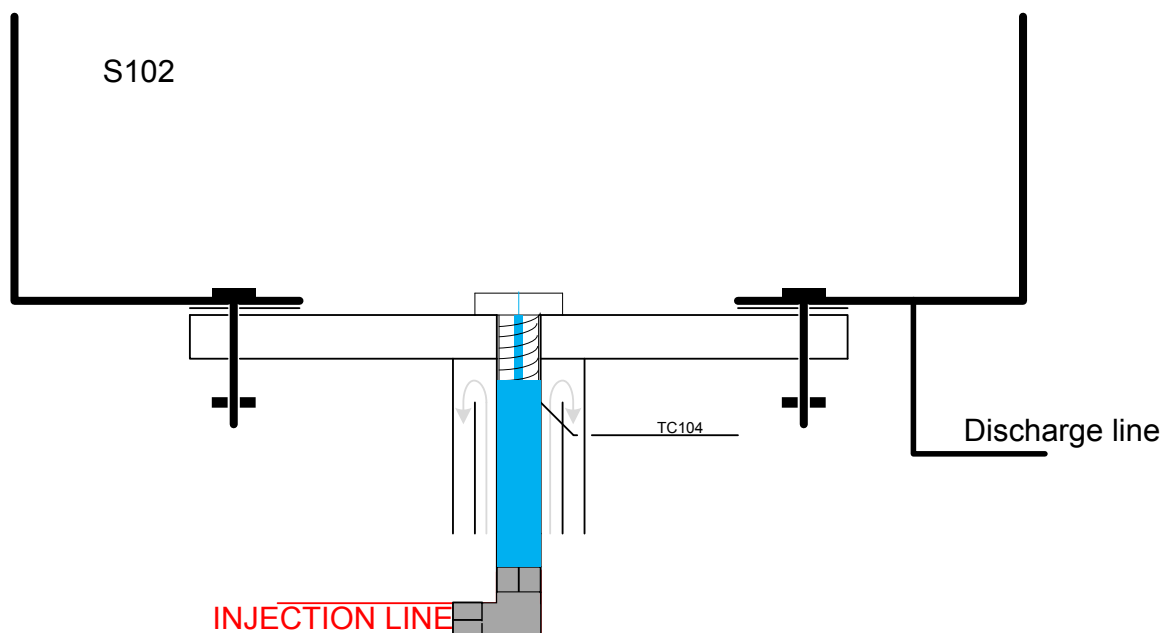
Fig. 5.15 – Principio di funzionamento del sistema iniezione e refrigerazione.
