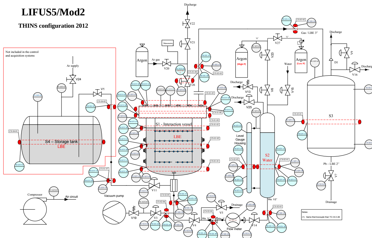
Fig. 4.4 – LIFUS5/Mod2. P&I configurazione THINS (parte 3 di 3): sistemi di controllo e regolazione.
