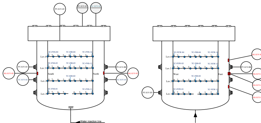
Fig. 4.3 – LIFUS5/Mod2. P&I configurazione THINS (parte 2 di 3): sistemi di controllo e acquisizione.
