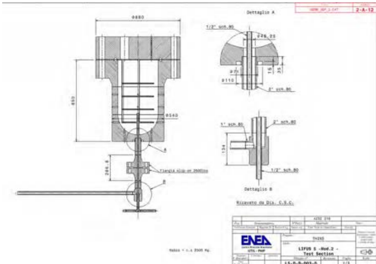
Fig. 5.14 – Assieme serbatoio S1 e particolari del sistema caricamento e iniezione dell'attuale configurazione LIFUS5/Mod2.
