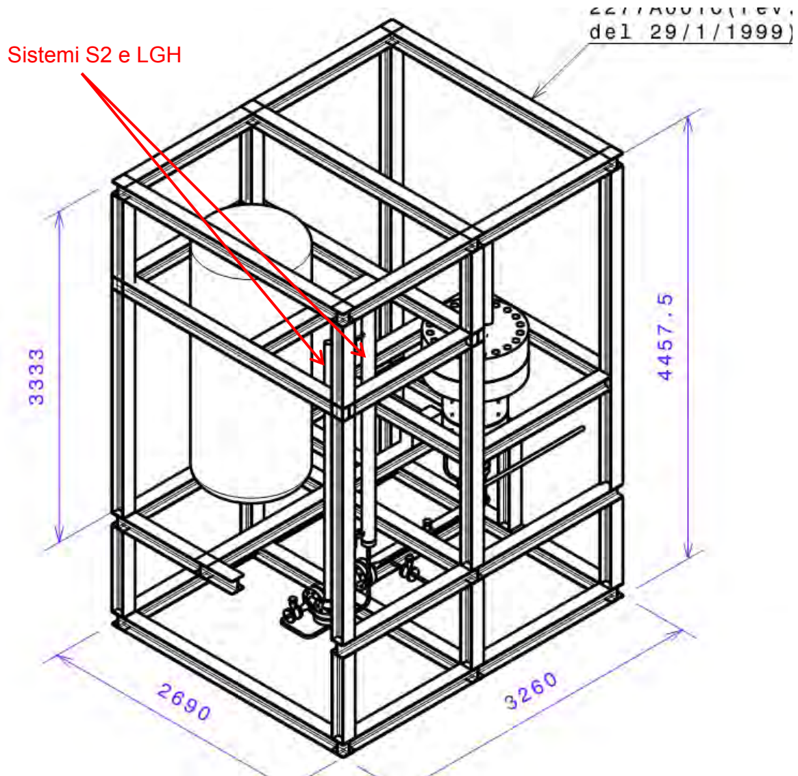
Fig. 5.16 – Struttura di supporto impianto LIFUS5.
