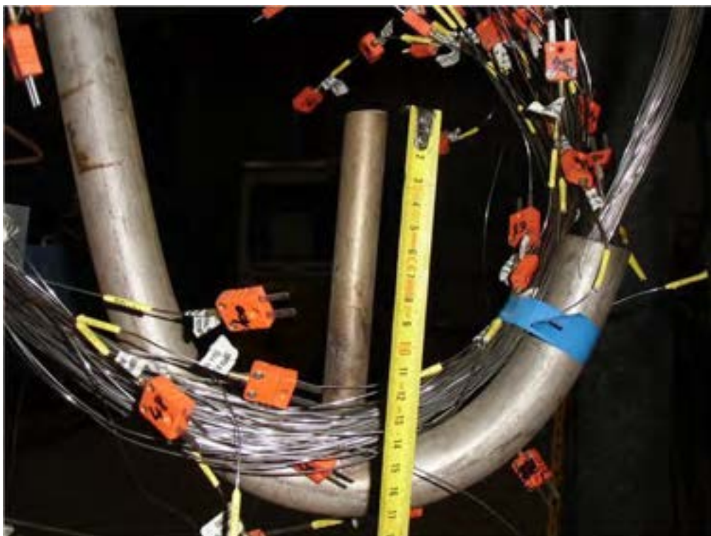
Fig. 5.9 – Tenuta TC con tubo collo d’oca (3 di 3).
