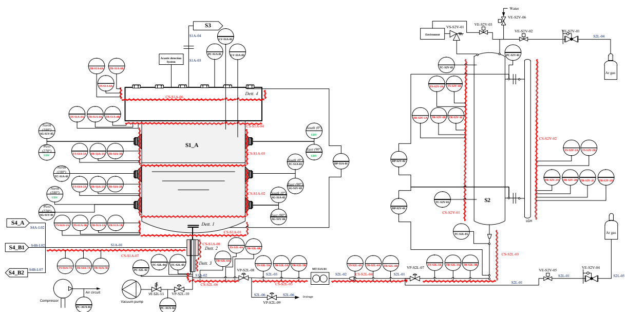
Fig. 5.10 – P&I preliminare sistema S1_A ed S2 dell'impianto LIFUS5/Mod3.
