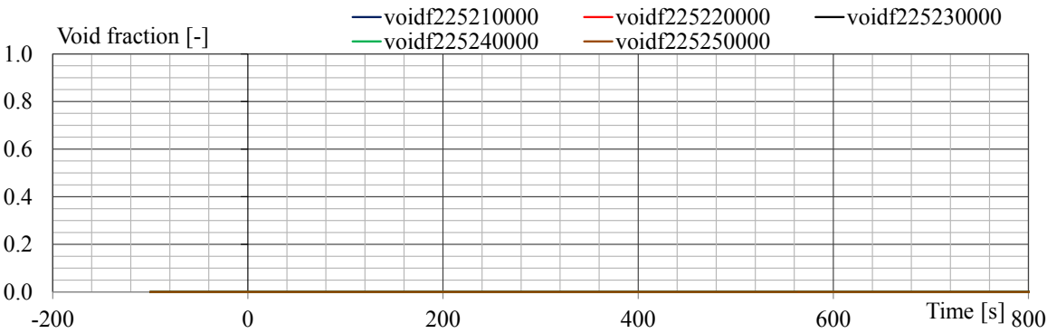
Fig. A. 5 – Void fraction in PIPE-225
