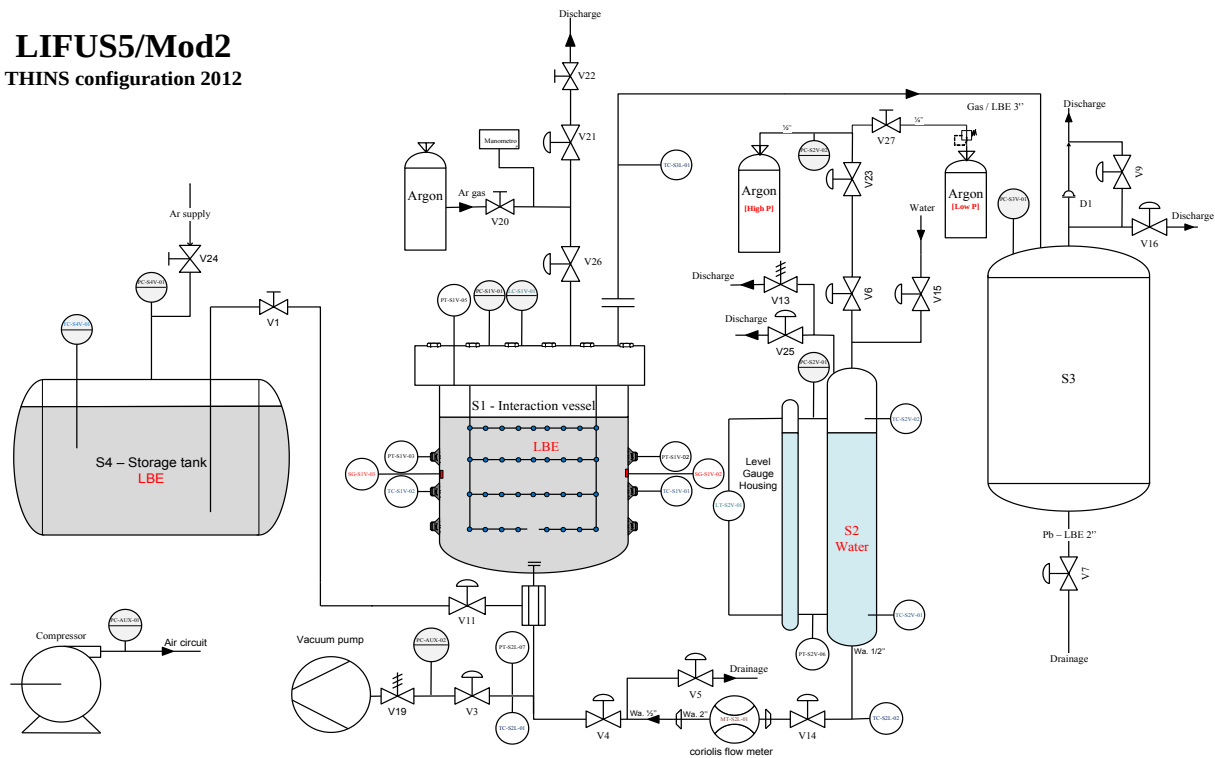
Fig. 4.2 – LIFUS5/Mod2. P&I configurazione THINS (parte 1 di 3): sistemi di controllo e acquisizione.
