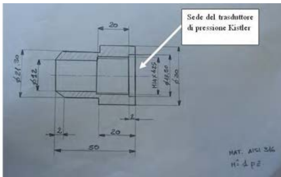
Fig. 5.5 – Adattatore trasduttore KISTLER
