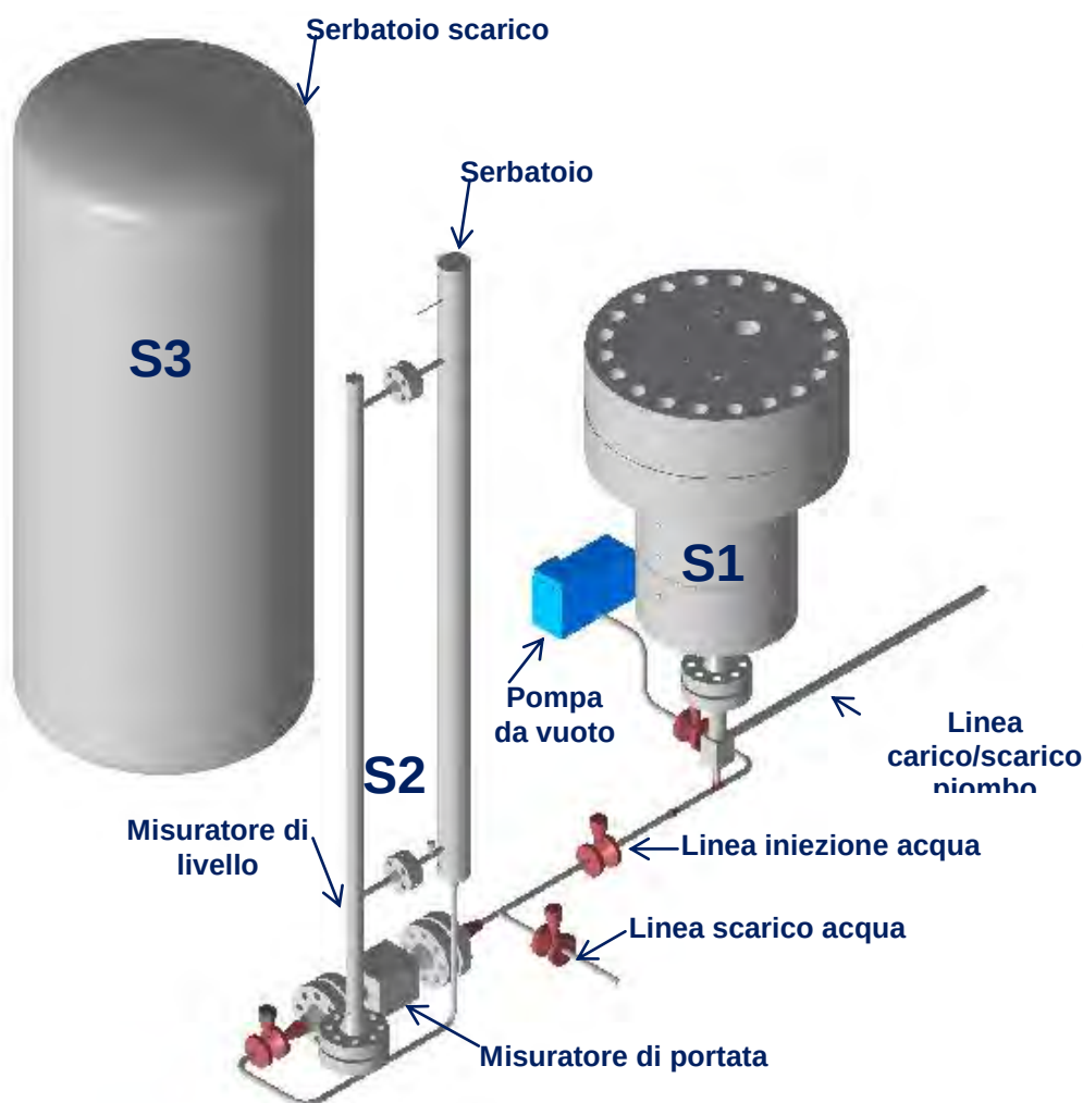
Fig. 4.1 – LIFUS5/Mod2, configurazione THINS: insieme del sistema, serbatoio di scarico disconnesso.
