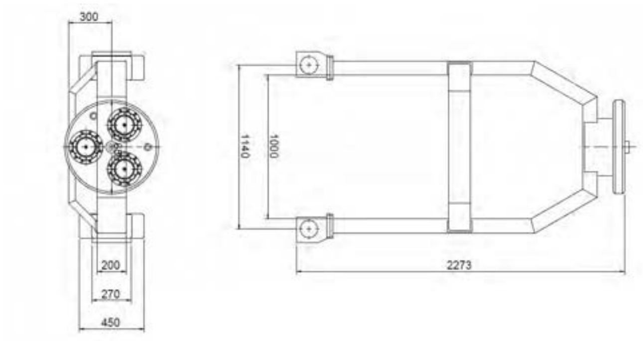
Fig. 2.26 - TA gripper dimensions
