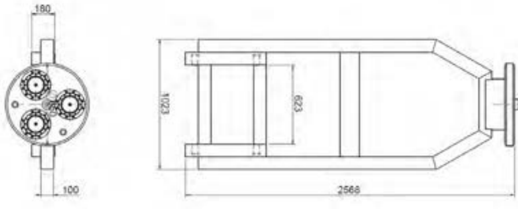
Fig. 2.23 - BP gripper dimensions
