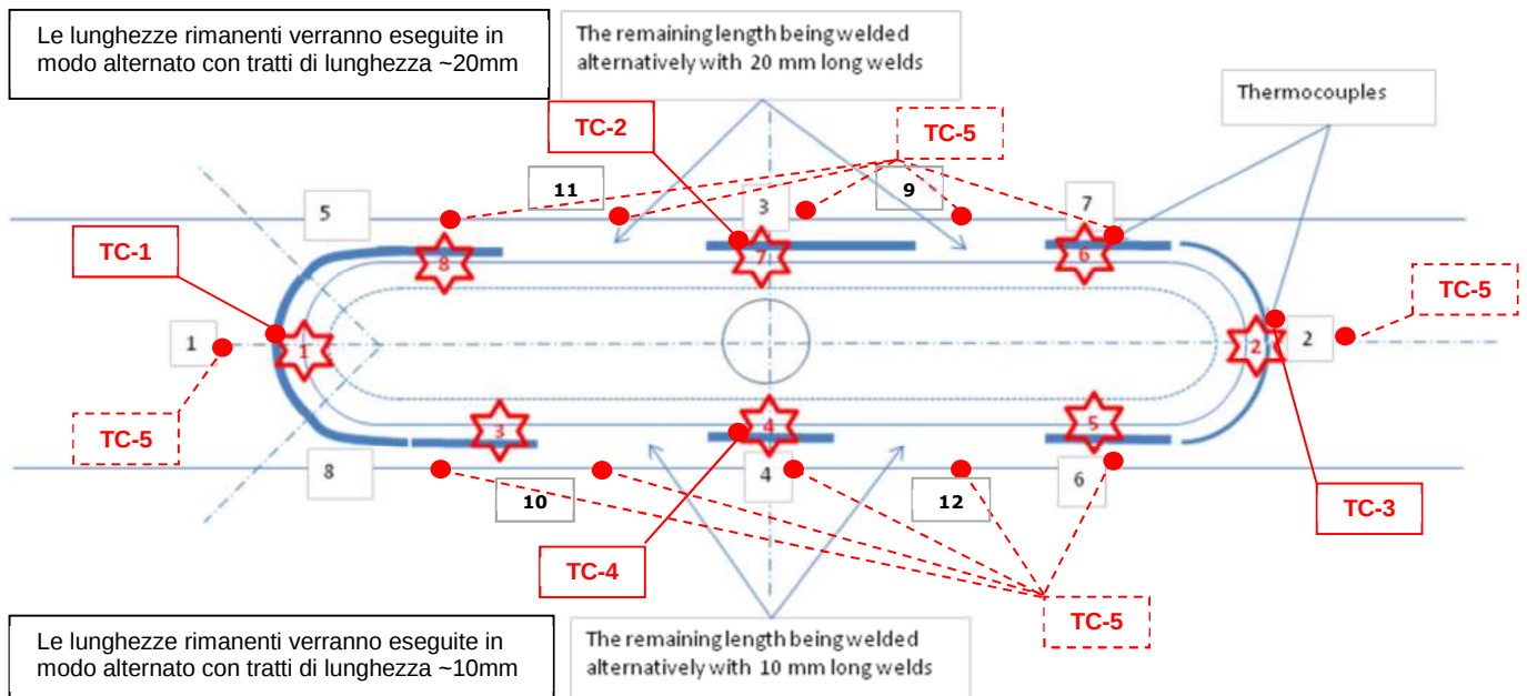
Fig.2 - Identificazione saldature di completamento (1 ÷ 12) e posizione termocoppie (TC-1 ÷ TC-4 +TC-5 esterna, posizionata sul jacket a seconda del tratto dalla saldatura) Welds identification (1 ÷ 12) and positioning of thermocouples (TC-1 ÷ TC-4 +TC-5 external TC, moved on the jacket on different positions)
