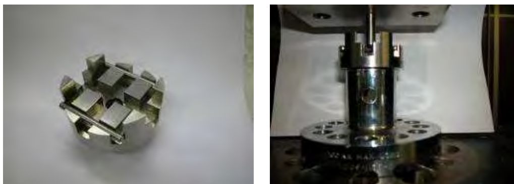
Figura 12 – Particolari dell'attrezzatura per le prove di trazione
