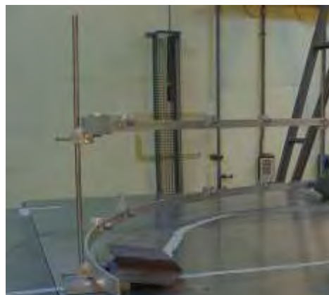
Figura 19 - Piattaforma d'acciaio posta in corrispondenza della piscina e dettaglio di un arco portadosimetri.
