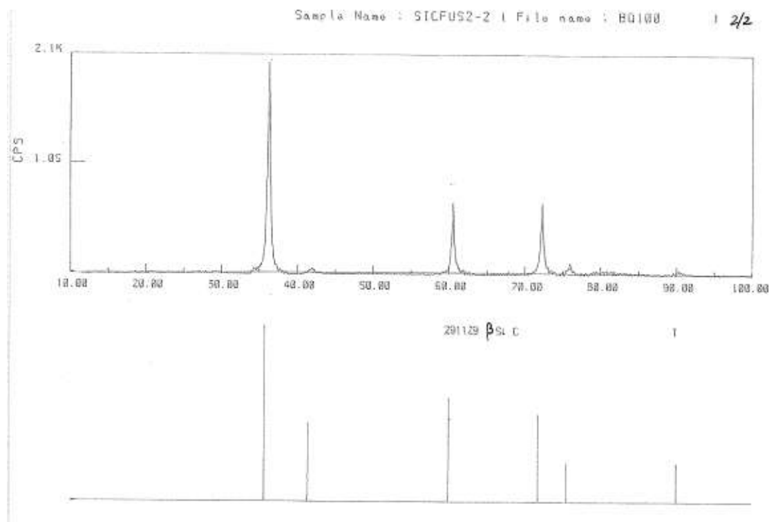
Figura 10 – XRD analisi
