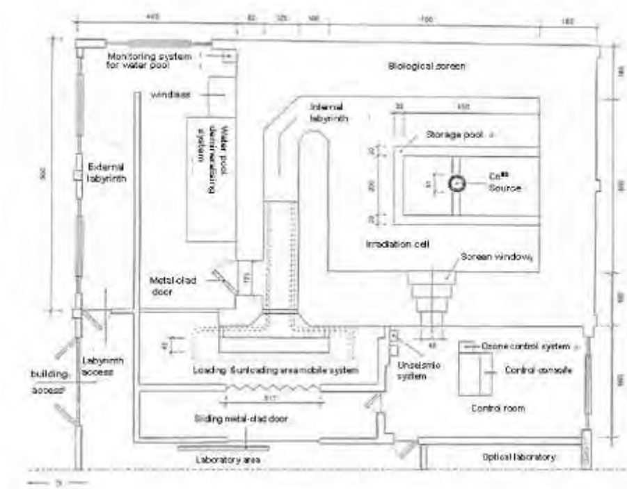
Figura 18 - Pianta dell'impianto Calliope
