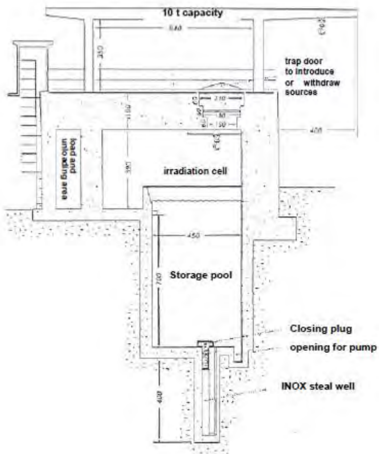
Figura 17 - Vista laterale dell'impianto Calliope
